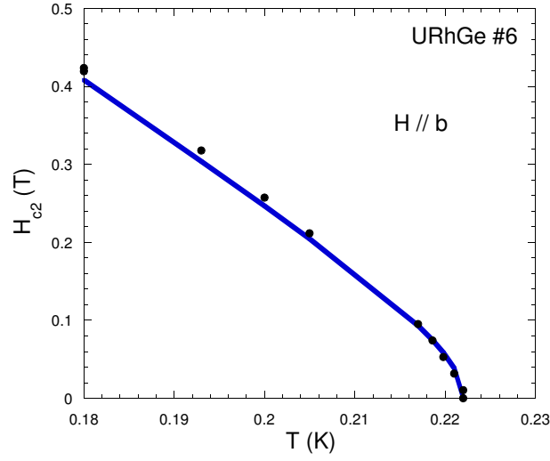
FIG. 7.17 – Ajustement de H_{c2}(T) près de T_c pour rendre compte de l'effet des domaines (direction \vec{b} ).
