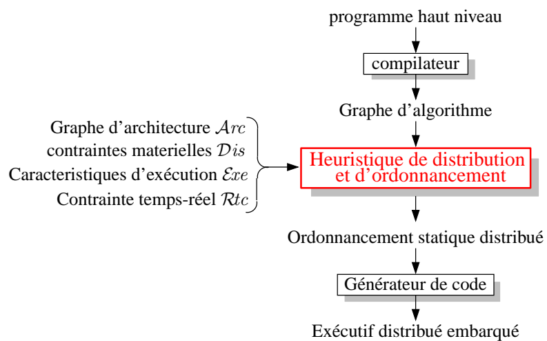
FIG. 9.10 – Processus de génération d'un exécutable par SYNDEX.
