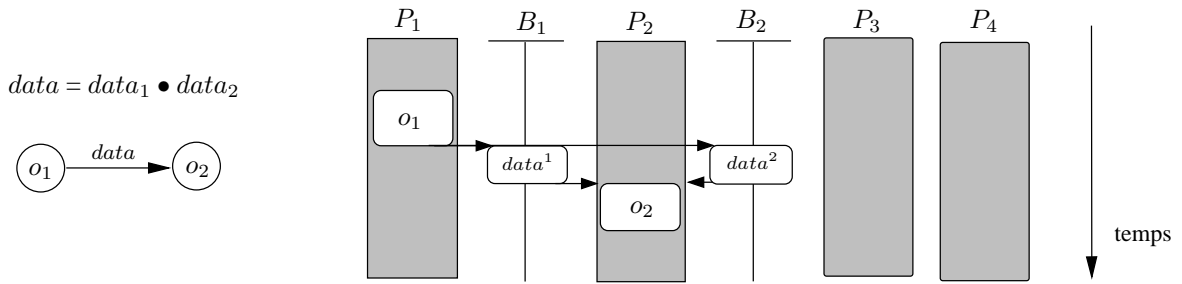
a. Graphe d'algorithme \mathcal{Alg}
