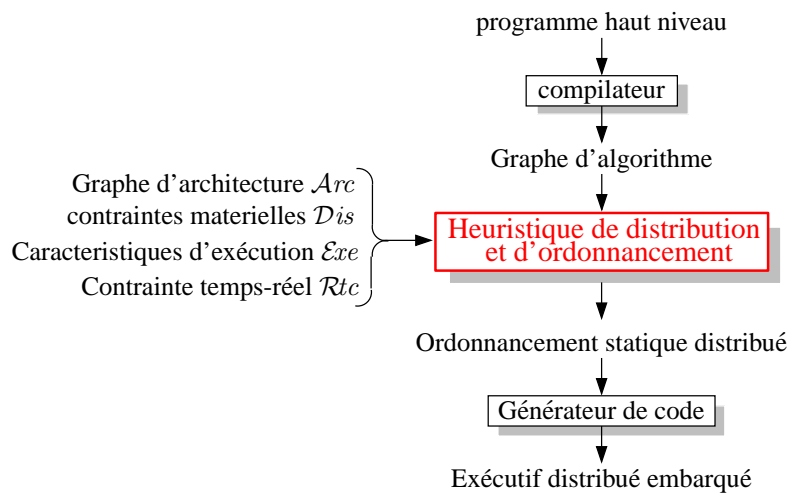
FIG. 9.10 – Processus de génération d'un exécuteur par SYNDEX.
