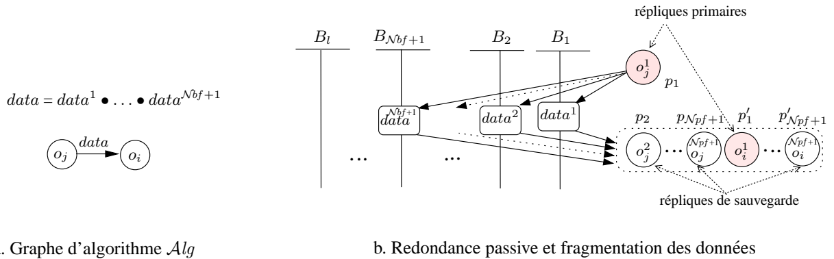
FIG. 7.9 – Tolérance aux fautes des processeurs et des bus de communication.
