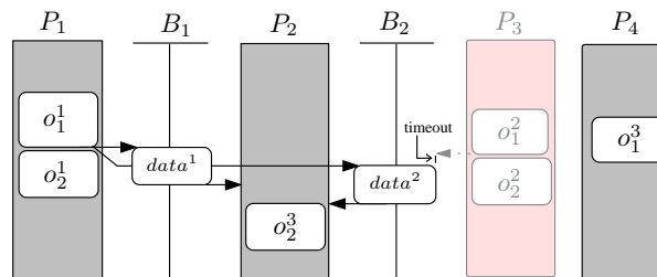
FIG. 7.7 – Recouvrement rapide des erreurs.
