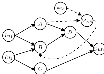
FIG. 4.3 – Exemple d'un graphe d'algorithme factorisé.
