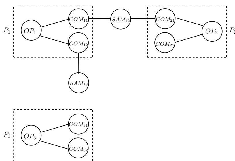
FIG. 4.8 – Modèle d'une architecture à liaisons point-à-point.
