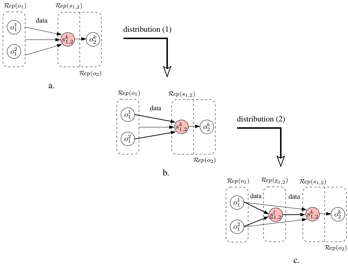
FIG. 6.8 – Schéma de transformation de Alg en Alg^* pour Npf = 1 et Nlf = 1 .
