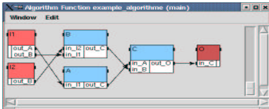
FIG. 9.2 – Exemple d'un graphe d'algorithme Alg .
