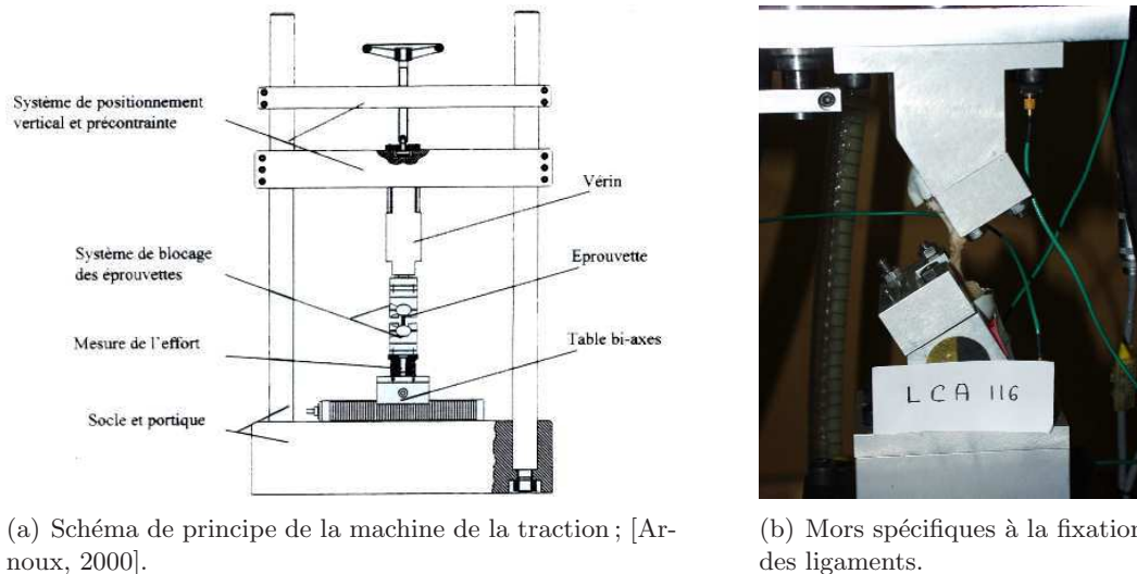
Fig. 5.9 - Machine de traction pour les essais des ligaments dans la direction des fibres.
