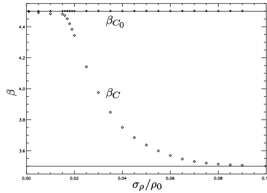
FIG. XII.18 – Évolution des indices spectraux \beta_C (losanges) et \beta_{C0} (croix) en fonction du rapport \sigma_\rho/\rho_0 , pour un cube de densité d'indice spectral \beta_\rho = 3,5 et un cube de vitesse \beta_v = 4,5 dont la valeur moyenne est v_0 = 30 \text{ km s}^{-1} . Les pointillés indiquent les asymptotes à \beta = 3,5 et \beta = 4,5 .
