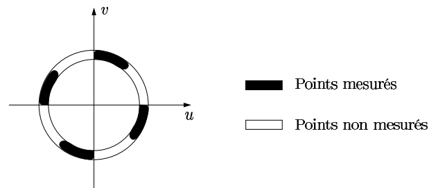
FIG. XVI.11 – Schéma du principe de la méthode de renormalisation décrite dans le texte. L'anneau compris entre les nombres d'onde k - \Delta k/2 et k + \Delta k/2 est séparé en régions pour lesquelles on dispose de mesures de visibilité (en noir) et pour lesquelles on n'a pas d'information (en blanc). Dans le cadre de l'hypothèse d'isotropie, la contribution de l'ensemble de l'anneau à la \Delta -variance de l'image non dégradée est proportionnelle à sa contribution à la \Delta -variance de l'image filtrée, le facteur de proportionnalité étant le rapport de l'aire totale de l'anneau à l'aire des régions noires.
