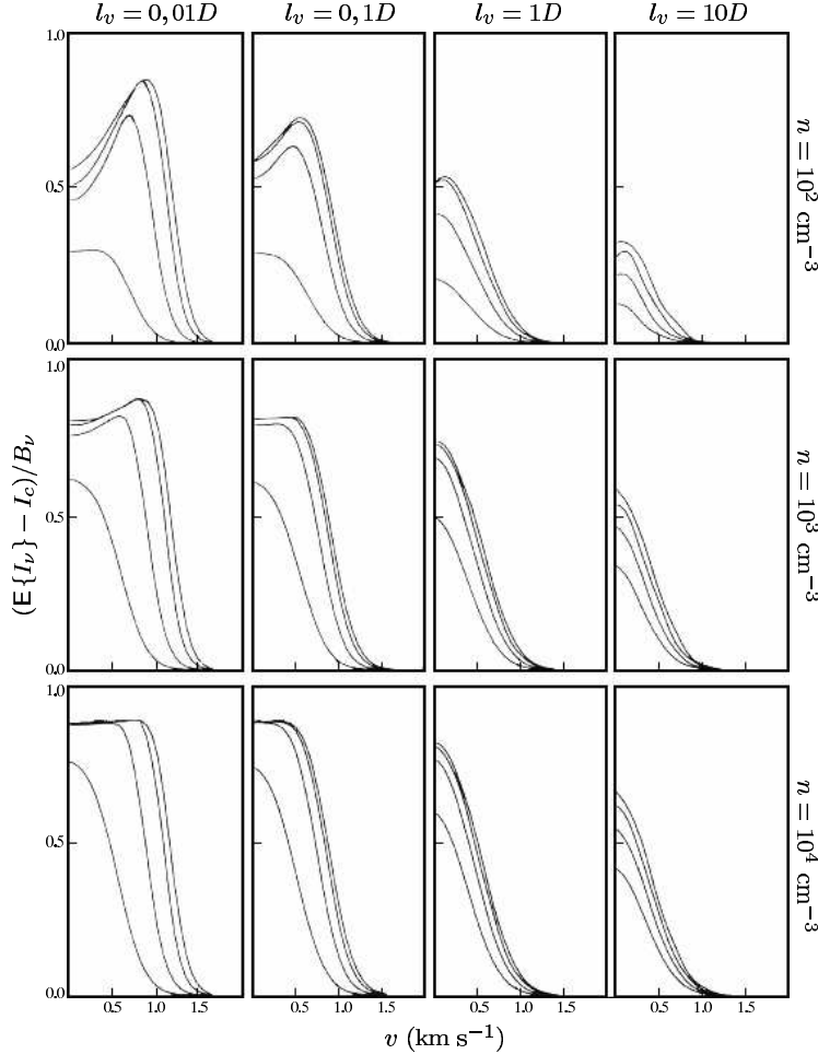
FIG. XIX.5 – Profils de raie calculés pour la transition J = 1 \rightarrow 0 du monoxyde de carbone. La vitesse turbulente \sigma_v est prise égale à 3\sigma_{th} , pour T_k = 10 K. Les différentes sous-figures correspondent à différentes valeurs de la densité n et de la longueur de corrélation l_v , comme indiqué en regard, en rappelant que D est la profondeur de la couche turbulente. Sur chacune des sous-figures, les quatre courbes correspondent aux différentes densités de colonne de CO considérées, soit N_{CO} = 10^{16} \text{ cm}^{-2} , N_{CO} = 10^{17} \text{ cm}^{-2} , N_{CO} = 10^{18} \text{ cm}^{-2} et N_{CO} = 10^{19} \text{ cm}^{-2} , en partant de la raie la moins intense. Figure issue de [Albrecht & Kegel, 1987].
