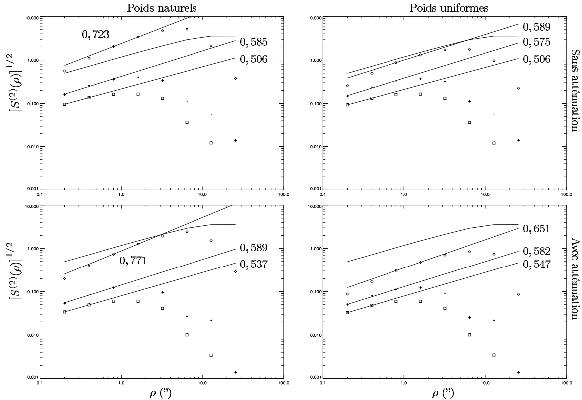
FIG. XVI.16 – Fonctions de structure grossières d'ordre deux calculées sur les images filtrées obtenues à partir de la distribution de brillance modèle \beta = 3, 1 . La première ligne correspond au cas sans atténuation par le lobe primaire, la seconde au cas où cette atténuation est prise en compte. Les deux colonnes correspondent aux deux fonctions de poids, comme indiqué. En ce qui concerne les configurations, les notations sont identiques à celles de la figure XVI.14, à savoir des losanges pour la configuration F, des croix pour la configuration E et des carrés pour la configuration D. La courbe en trait plein représente la fonction de structure calculée sur la distribution de brillance initiale. Les tirets indiquent les ajustements de lois de puissance décrits dans le texte. Les exposants de Hurst correspondants sont indiqués en regard.
