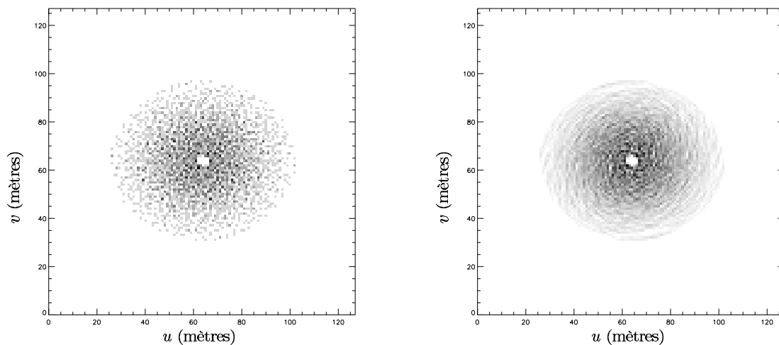
FIG. XV.7 – Couvertures (u, v) rééchantillonnées sur une grille orthonormée. Il s'agit des couvertures illustrées sur la première ligne de la figure XV.6 . La taille des cellules dans les deux directions u et v est égale au rayon d'une antenne.
