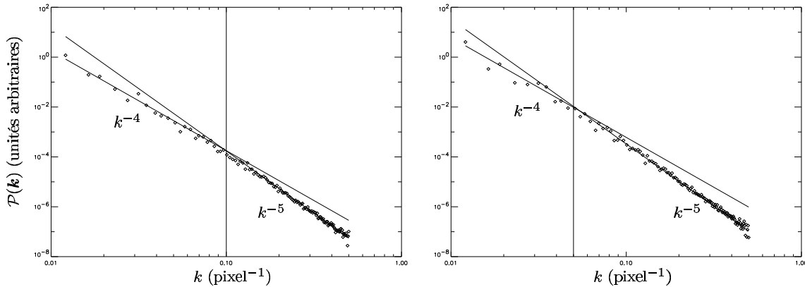
FIG. XII.9 – Spectres de puissance de cartes bidimensionnelles construites en sommant respectivement cinq plans (figure de gauche) et dix plans (figure de droite) consécutifs extraits du cube de densité \beta_\rho = 5 . Les mesures sont indiquées par des losanges, et les droites représentent les régimes limites R \ll d et R \gg d . Les pointillés correspondent au nombre d'onde de la transition k_d = 1/2d .
