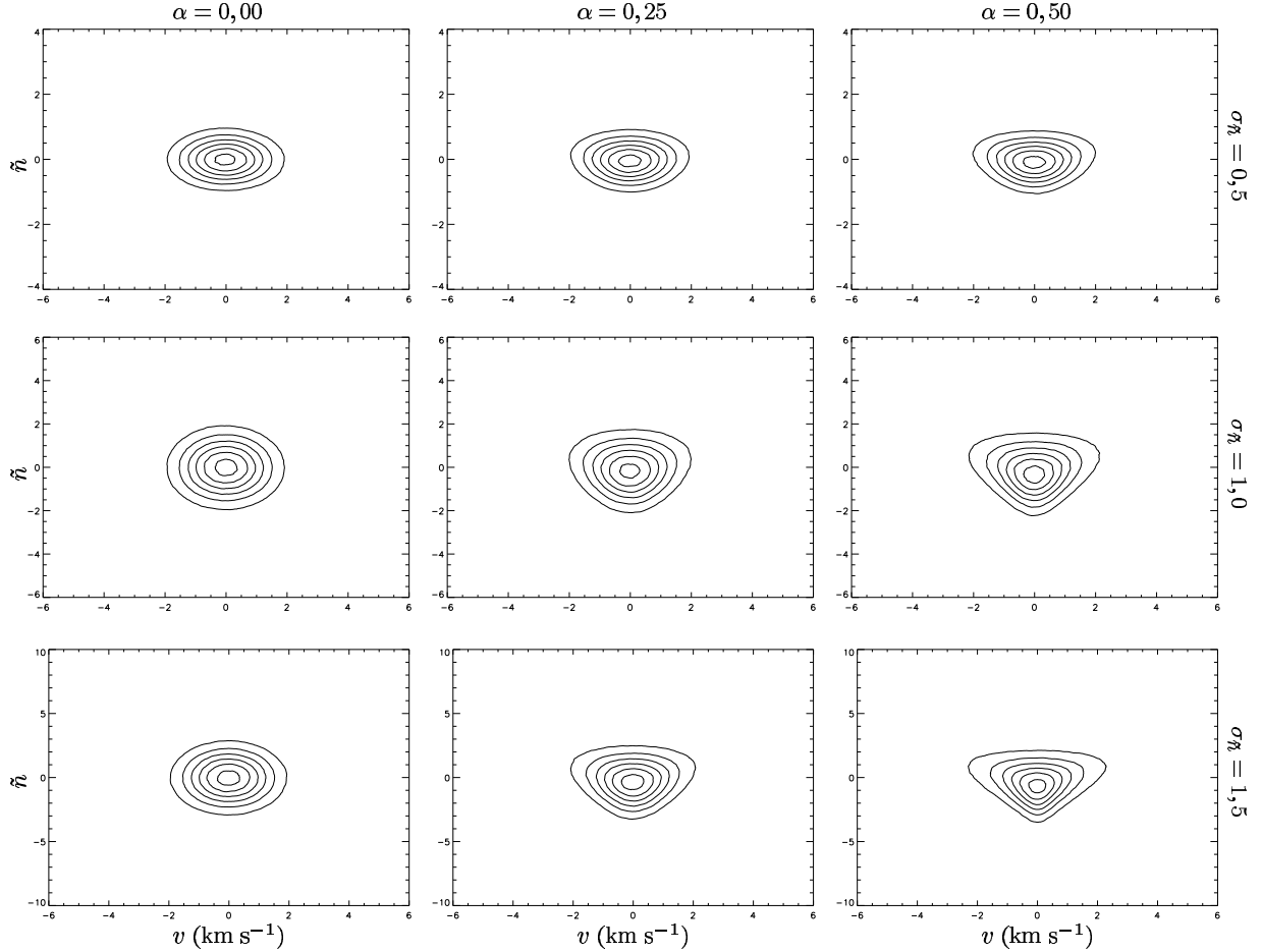
FIG. XX.5 – Distributions jointes W(v, \tilde{n}) obtenues pour les mêmes valeurs des paramètres que celles utilisées sur la figure XX.4 . La disposition des sous-figures est également la même.
