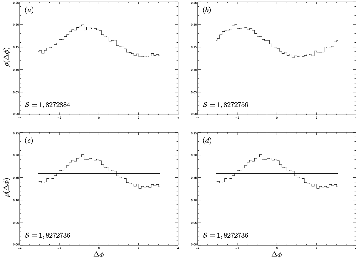
FIG. XVII.7 – Illustration des effets des transformations élémentaires. La figure (a) représente l'histogramme des incréments de phase de la densité de colonne de la figure XVII.6 , pour \delta = \mathbf{e}_x - \mathbf{e}_y , et constitue la référence. La figure (b) représente l'histogramme des incréments de phase, pour le même déplacement \delta , d'une image obtenue par translation de vecteur 100\mathbf{e}_x . On remarque que l'histogramme est déplacé en bloc, sans modification sensible de sa forme. Les figures (c) et (d) correspondent quant à elles respectivement aux cas d'une rotation d'angle \pi/2 , et d'une symétrie par rapport à l'axe Ox , et ce pour un déplacement \delta = \mathbf{e}_x + \mathbf{e}_y dans les deux cas. Les histogrammes sont sensiblement identiques à celui de référence, comme le prévoit la théorie. Les entropies correspondantes sont indiquées dans le coin inférieur gauche de chaque figure et sont toutes égales, à 10^{-5} près.
