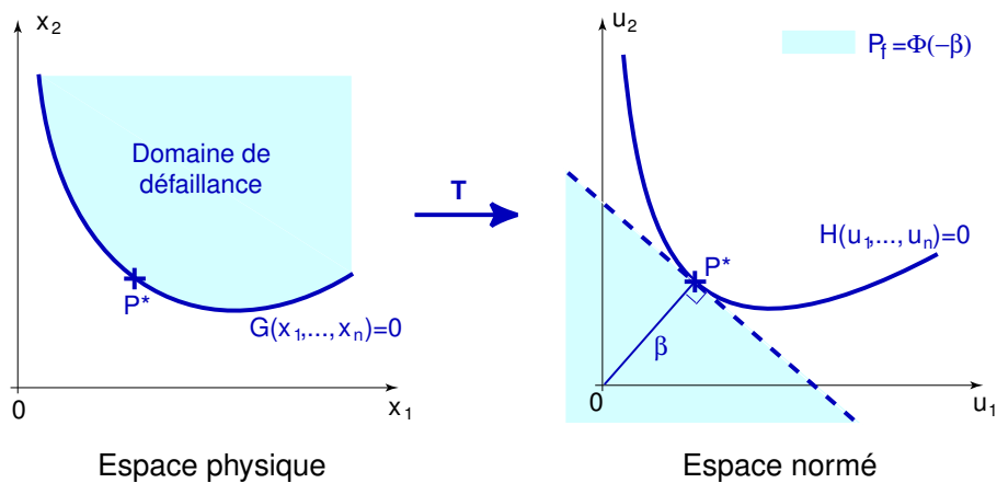
FIG. 1.2 – Principe des méthodes fiabilistes : exemple de l'approximation FORM
