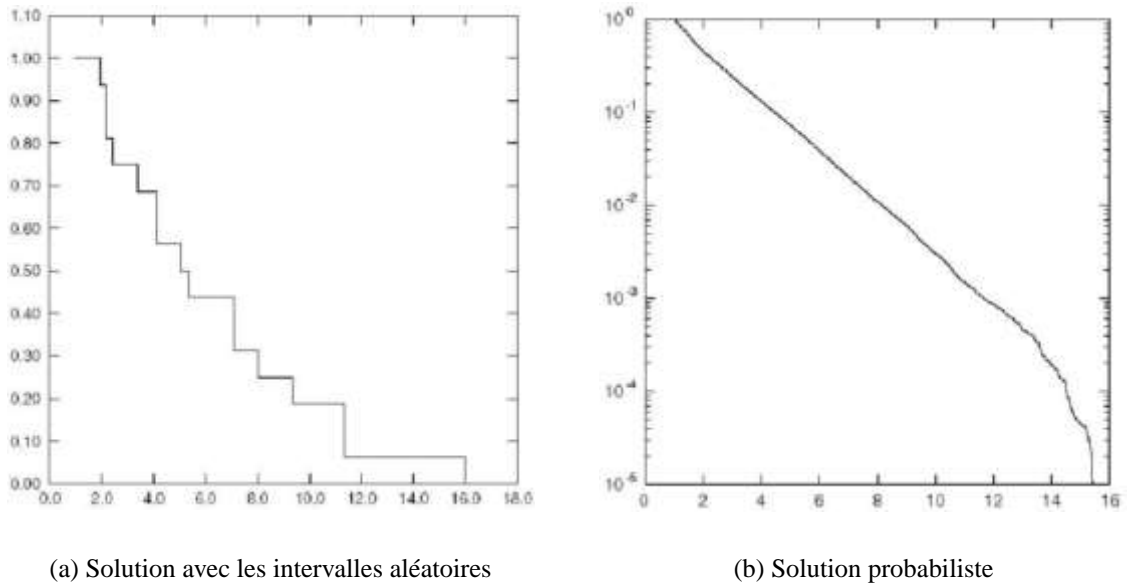
FIG. 2.1 – Comparaison des résultats obtenus sur un exemple simple par une représentation par intervalles aléatoires et une modélisation probabiliste, d’après [Oberkampff et al. 2001]
