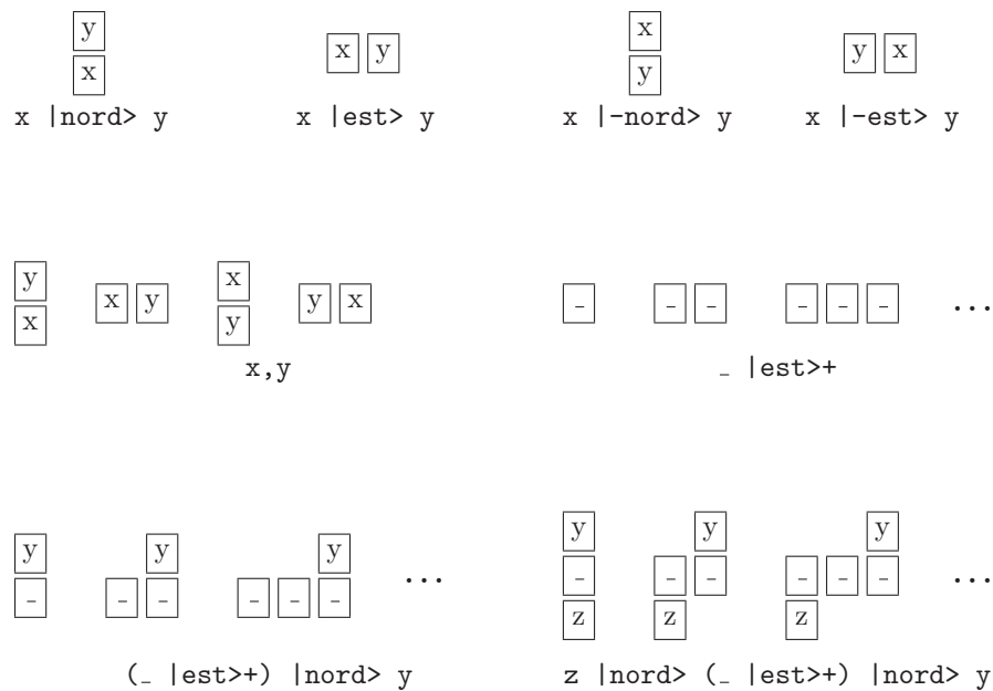
FIG. 5 – Exemples de motifs sur le GBF grille et parties filtrées correspondantes.
