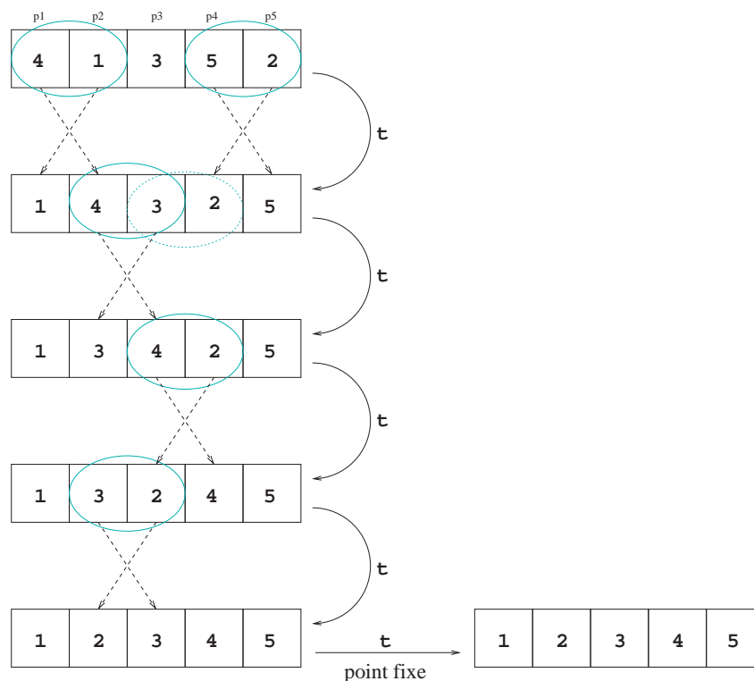
FIG. 2 – Une trace possible du tri d'une séquence.
