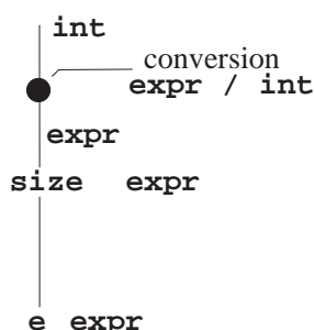
FIG. 4 – Termes étiquetés par leur implémentation (2).
