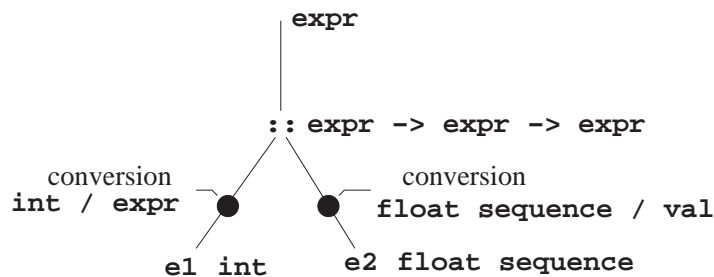
FIG. 2 – Termes étiquetés par leur mode d'implémentation.
