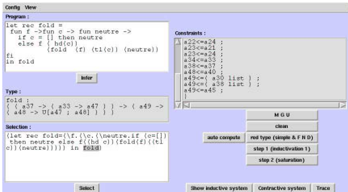
FIG. 6 – Version visuelle du module d'inférence de types.
