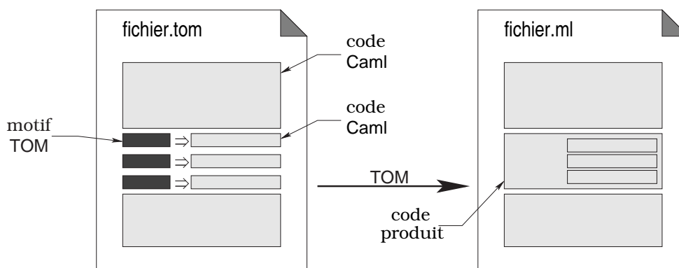
FIG. 11 – TOM est non intrusif : il transforme un motif en algorithme de filtrage.
