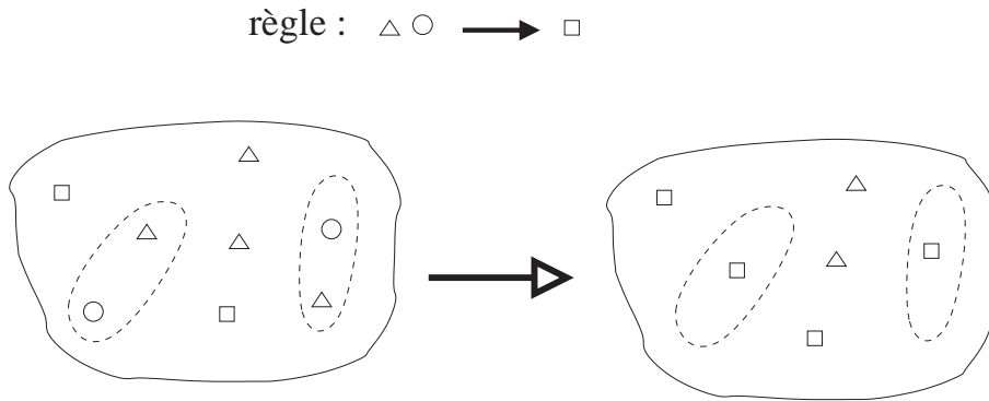
FIG. 1 – Transformation d’une collection. Une règle spécifie qu’une sous-collection A doit être remplacée par la sous-collection A' calculée à partir de A . La collection calculée dans la partie droite de la règle dépend de la sous-collection filtrée dans sa partie gauche et éventuellement de son voisinage.
