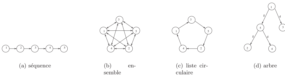
FIG. 1 – Collections topologiques vues comme des graphes
