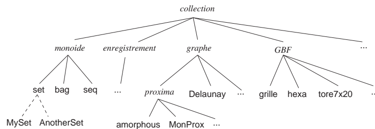
FIG. 2 – Hiérarchie sur les types de collections. MySet et AnotherSet sont des types de collections définis par l'utilisateur. Les types collection et monoïde ne correspondent pas à des structures de données concrètes. Formellement, un enregistrement est un ensemble de paires \langle \text{nom-du-champ}, \text{valeur-du-champ} \rangle mais son utilisation nécessite des opérateurs particuliers.
