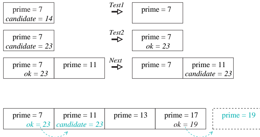
FIG. 3 – Le programme Erato . Quelques instanciations de règles et un fragment de séquence construit par la transformation Erato .
