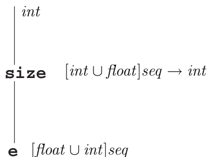
FIG. 3 – Termes étiquetés par leur type (2).
