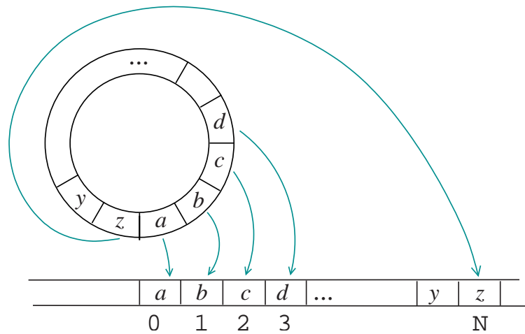
FIG. 5 – Codage d’une topologie d’anneau sur un champ de données de dimension 1. Chaque point d’indice i pour 0 \leq i \leq n dans le champ de données correspond à un élément de l’anneau. L’opération qui permet de calculer l’indice j du voisin de droite d’un élément d’indice i est alors définie par : j = i + 1 \text{ mod } n .
