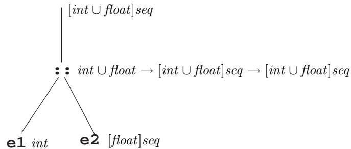
FIG. 1 – Termes étiquetés par leur type.
