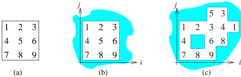
FIG. 4 – Notion de tableau et de champ de données. (a) : un tableau. (b) : le même tableau vu comme un champ de données : c’est une fonction qui associe à chaque indice (i, j) une valeur. Cette fonction est partielle : la plupart des indices (il y en a une infinité) ne sont associés à aucune valeur. Le domaine de définition du champ de données est symboliquement représenté par une région blanche sur le fond grisé. (c) : un champ de données permet de représenter simplement des régions arbitraires qui généralisent les régions rectangulaires des tableaux.
