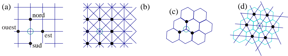
FIG. 3 – Exemples de treillis discrétisant de manière homogène un espace plan. (a) : treillis rectangulaire à 4 voisins appelé voisinage de Von Neuman . (b) : treillis rectangulaire à 8 voisins appelé Voisinage de Moore . (c) : treillis triangulaire : chaque point possède trois voisins. (d) : treillis hexagonal : chaque point possède 6 voisins. Si on représente chaque point de l'espace par une cellule hexagonale, et que la connexion entre deux points est représentée par le partage d'une face de la cellule, on obtient un pavage hexagonal.
