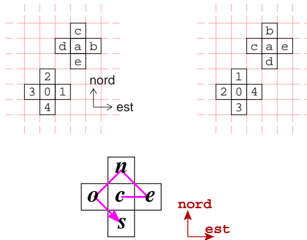
FIG. 6 – Rotation d'un motif sur une grille carrée. nord et est sont les deux générateurs.
