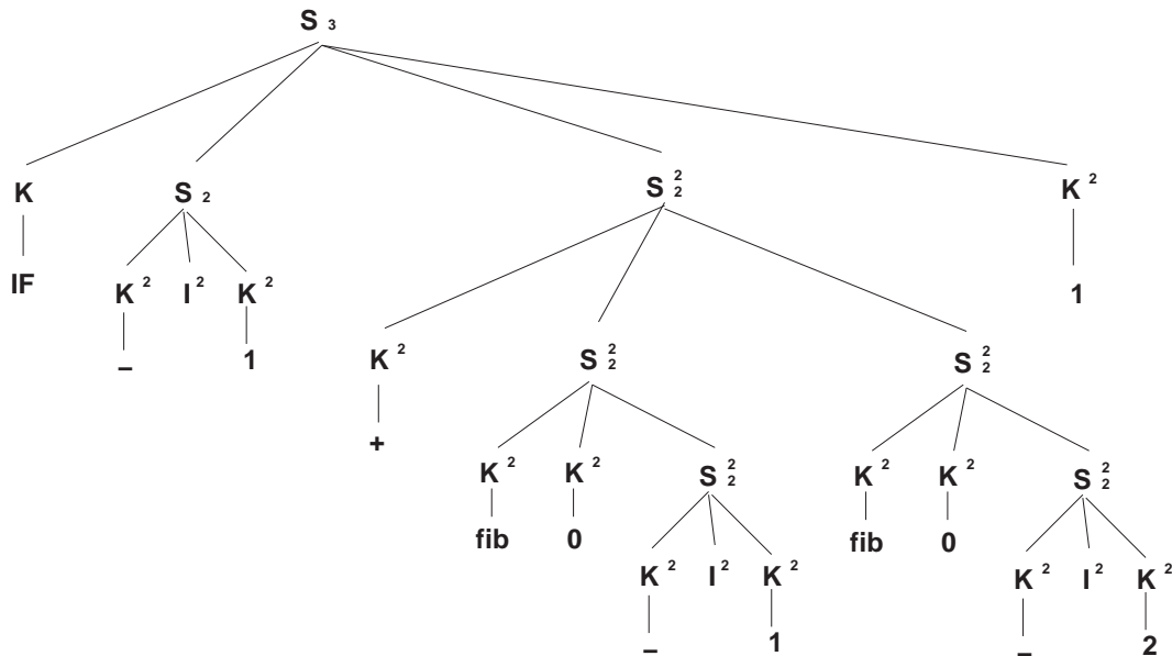
FIG. 1 – Représentation sous forme arborescente de l'expression de fib.
