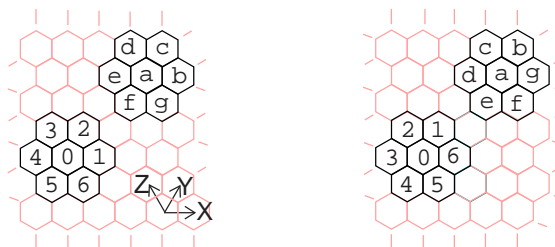
FIG. 7 – Rotation d'un motif sur un pavage hexagonal. X , Y et Z sont les générateurs.
