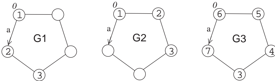
FIG. 7 – Trois instances de GBF de type A5 construit avec l'opérateur following .
