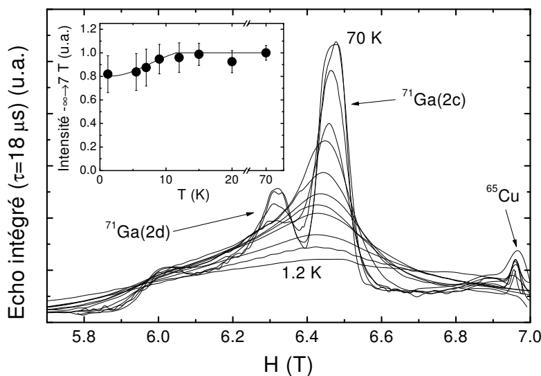
FIG. 7.1 – Série de spectres entre 70 K (largeur minimale, amplitude maximale) et 1.2 K (largeur maximale, amplitude minimale). L'intensité correspondante (l'aire d'une raie, proportionnelle au nombre de spins dont la résonance est mesurée) est donnée en encart. La perte d'intensité en dessous de \sim 10 K est compatible avec la perte des \frac{2}{3} des sites ^{71}\text{Ga}(2d) dans la signal.
