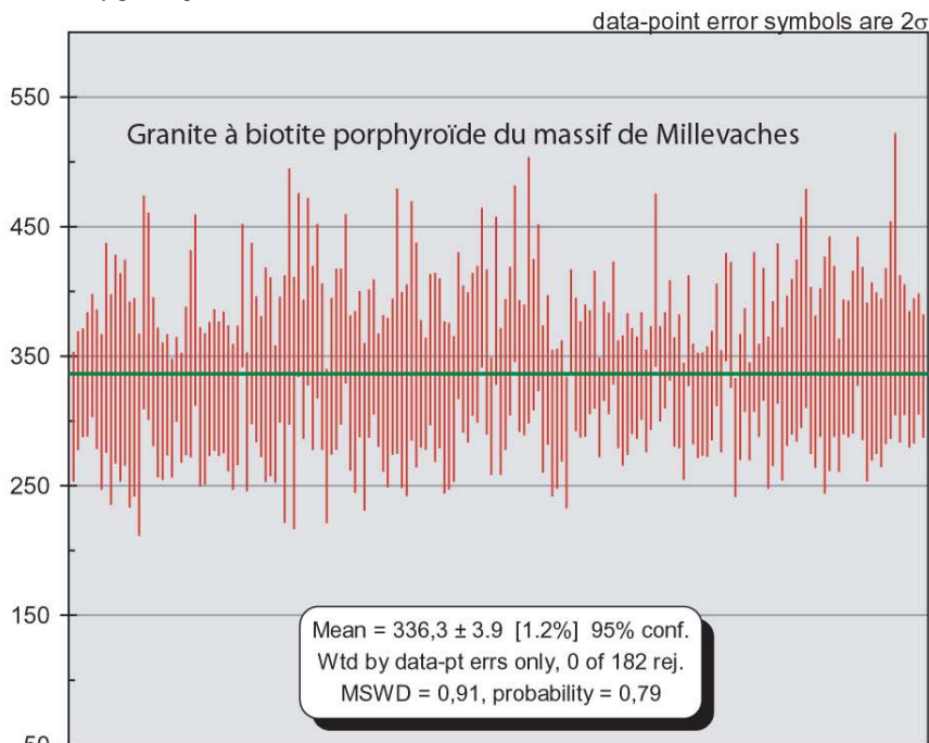
Fig. IV-32a : Moyenne pondérée des âges individuels et barres d'erreur de l'échantillon MVG4.
