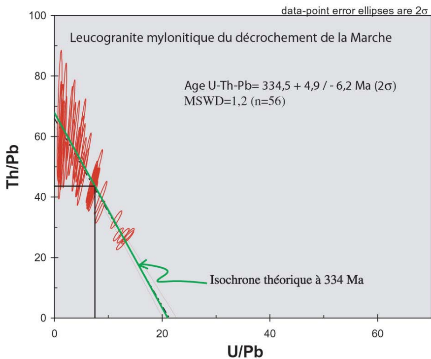
Fig. III-12b : Diagramme isochrone Th/Pb=f(U/Pb). Echantillon 284
