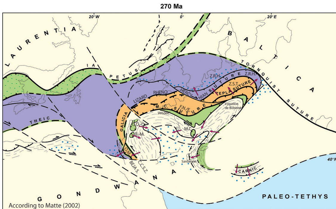
FIG. I-6 – Chaîne Varisque d'Europe de l'ouest et du nord de l'Afrique au Permien d'après MATTE (2002) laissant apparaître les zones de suture principales et l'extension des microplaques Avalonia et Armorica. En vert et pointillés : Suture Calédonienne Iapetus. En violet : Avalonia. En orange : Armorica. En vert : Nappes ophiolitiques enracinées dans la suture Galicia-Massif Central. Tiretés : Nappes de la zone méridionale. Pointillés bleus : Bassins externes Carbonifères. Flèches rouges : Vergence des nappes. C.C.S.Z. : Coïmbra-Cordoba shear zone. Beja S. : Beja suture. O.M. : Ossa Morena. B.-M. : Bragança et Morais. C.O.-O. : Cabo Ortega et Ordennes. Z.S.T : Zone Saxo-Thuringienne. Z.R.H. : Zone Rheno-Hercynienne. M.C. : Massif Central. F.N./E. : Faille Nord sur Etre.
