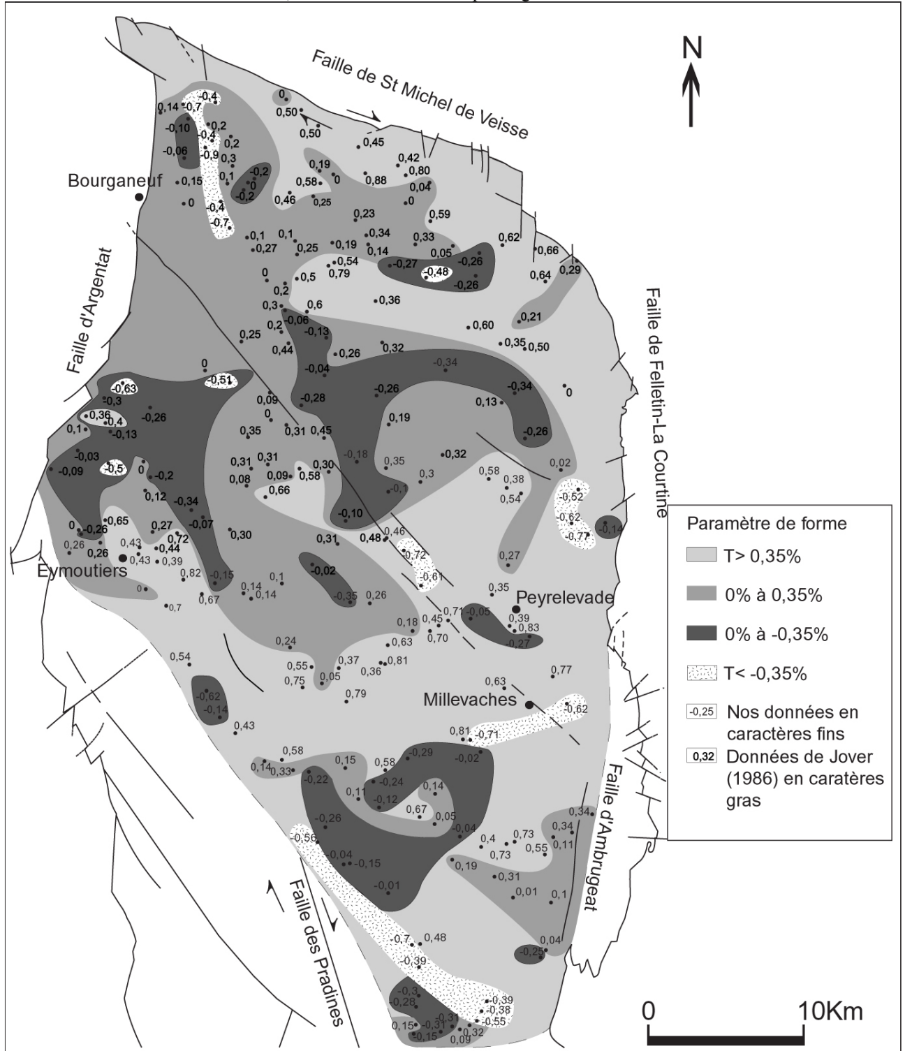
FIG. IV-22 – Répartition géographique du paramètre de forme T
