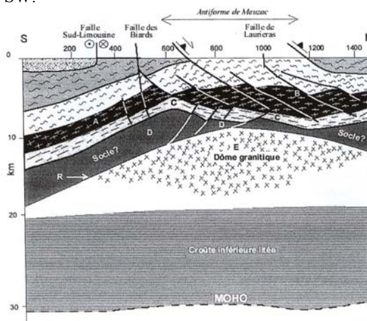
FIG. IV-4 – Interprétation du profil sismique Laurières. A et B: Unités gneissiques. C: Unités para-autochtone. D: Unité discordante (socle ?). E: Zone sismiquement transparente. R: Réflecteur au toit de la zone sismiquement transparente.
