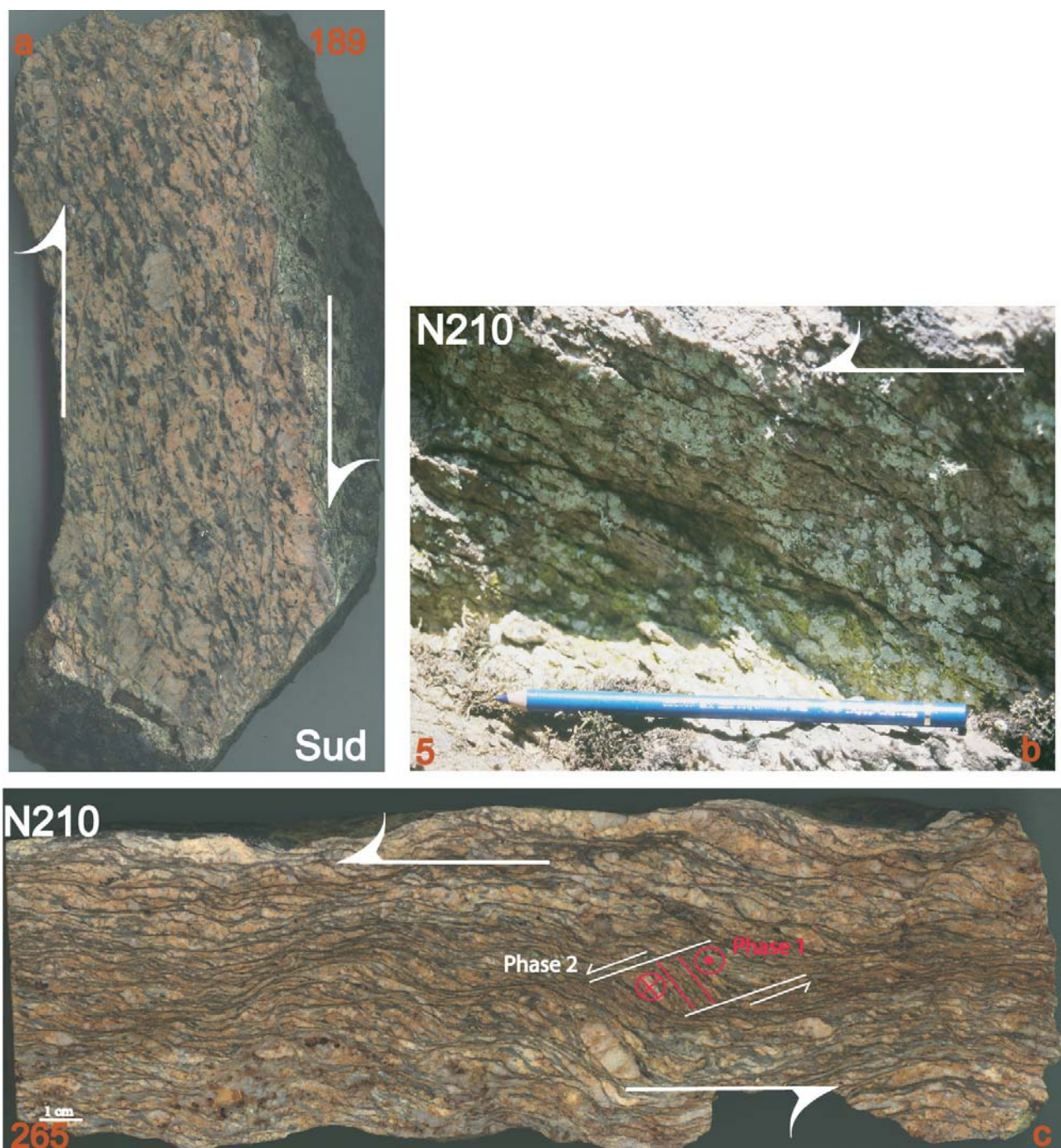
PLANCHE I- Microstructures dans les leucogranites de bordure du massif de Millevaches à l'échelle du macroéchantillon. a : Echantillon 189. Microstructure C-S indiquant un mouvement décrochement dextre avec abaissement du compartiment Est. b : Echantillon 5. Bandes de cisaillement mettant en évidence le mouvement inverse vers le SW. c : Echantillon 265. Echantillon ayant enregistré les deux phases. La première en décrochement dextre, la seconde en mouvement inverse vers le SW.
