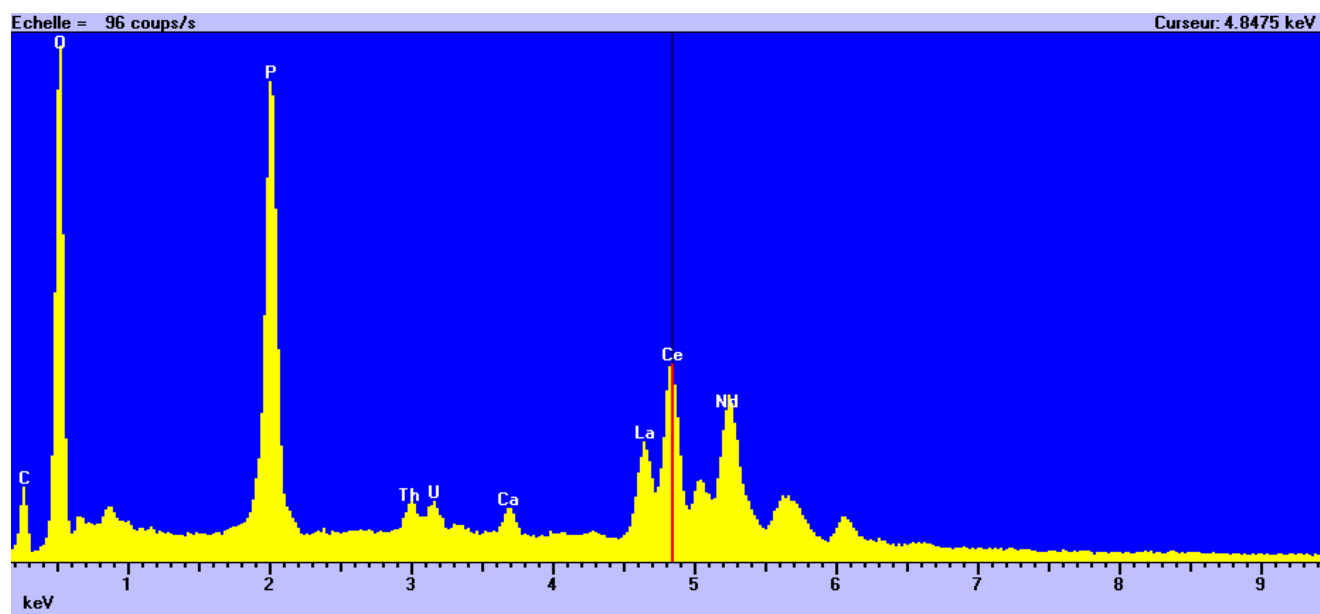
FIG. II-8 – Spectre EDS (Système à dispersion d'énergie) caractéristique de la monazite.
