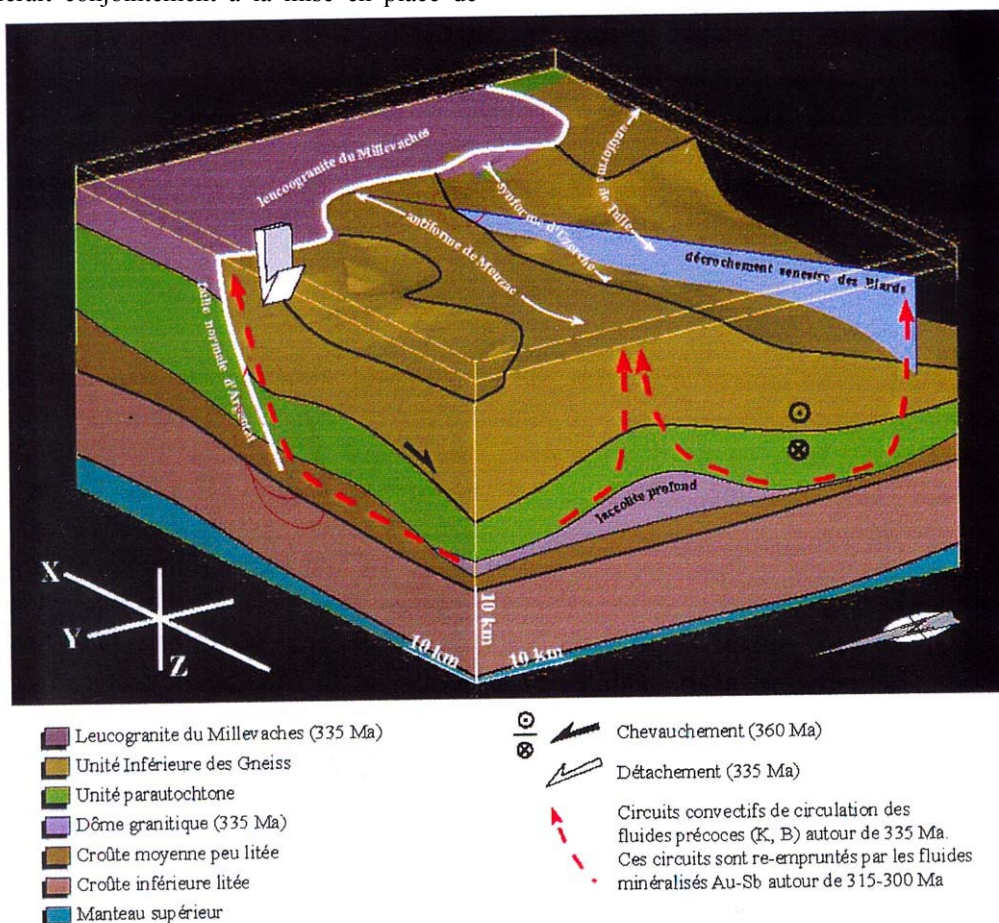
FIG. IV-6 – Modèle géométrique 3D obtenu pour le Sud-Limousin d'après BELLOT (2001)
