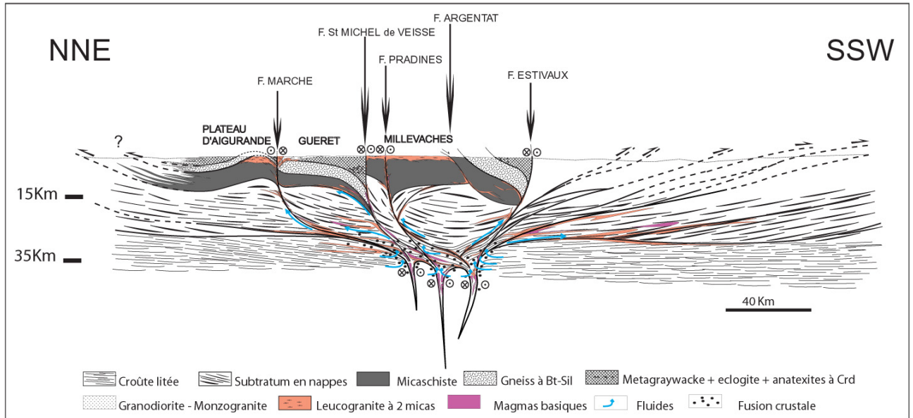
FIG. V-7 : Schéma simplifié de la « pop-up structure » vers 300 Ma en coupe.
