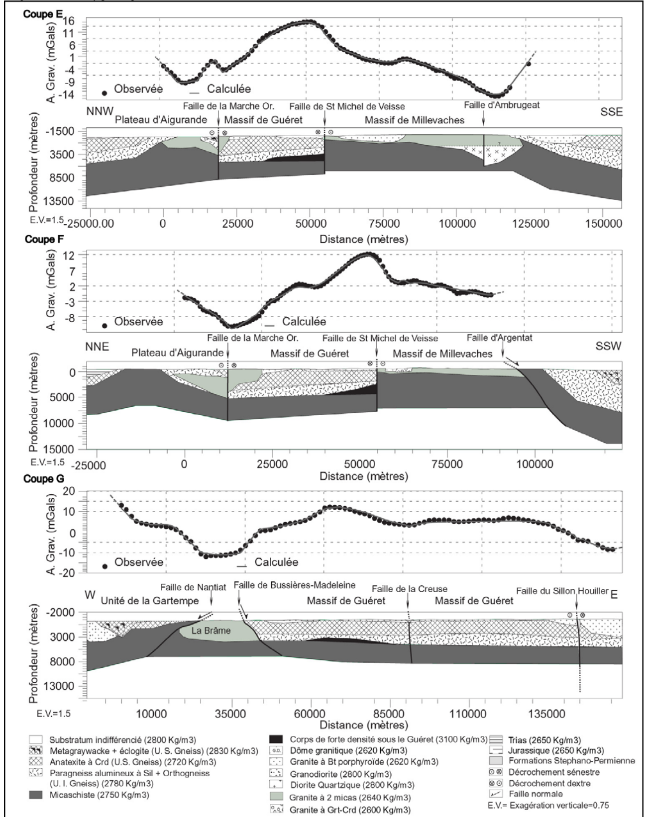
FIG. IV-15- Modélisations gravimétriques à l'échelle régionale.
