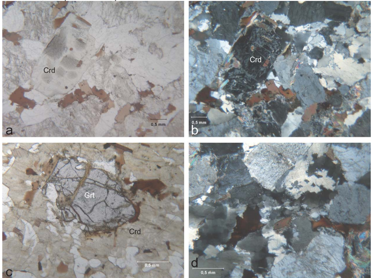
PLANCHE VI - Microstructures observées dans les anatexites à cordiérite de la bordure Est du massif de Millevalches. a : Cordiérite pinitisée en lumière naturelle. b : Cordiérite pinitisée en lumière polarisée. c : Grenat en inclusion dans une cordiérite pinitisée. d : Texture du quartz mettant en évidence des quartz en échiquier (en bas à gauche) et de quartz en mosaïque (joints de grains à 90°).
