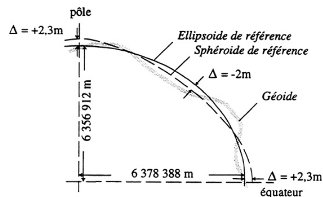
FIG. II-6 – Représentation schématique du système de référence de la Terre : Sphéroïde, Ellipsoïde et Géoïde d'après VAN DEN BOSCH (1981).
