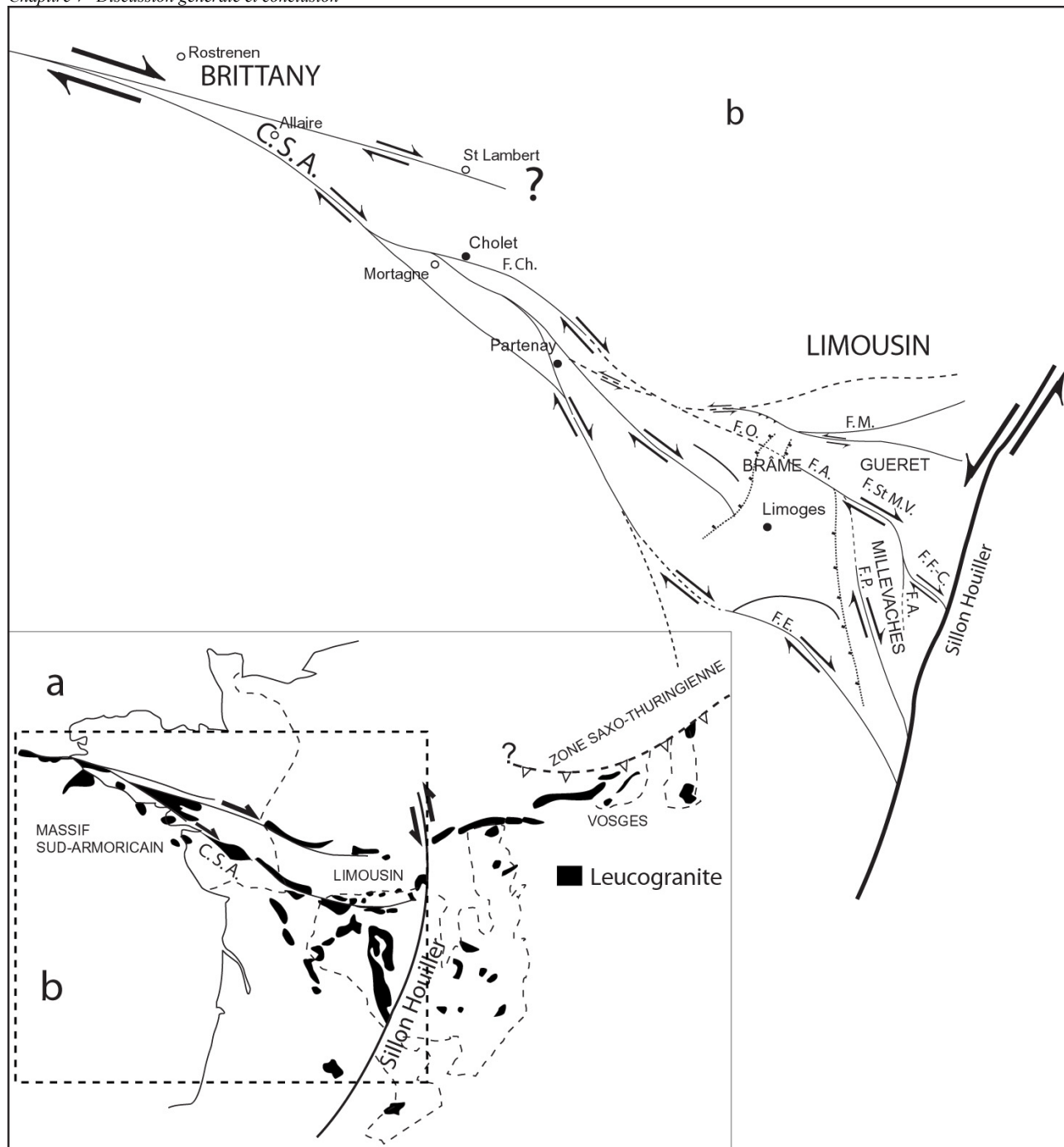
FIG. V-5 – a : Carte des leucogranites de la France associés aux zones de cisaillements ductiles d'après AUTRAN et LAMEYRE (1980). C.S.A. : Cisaillement Sud Armoricain. b : Raccord entre les décrochements du Limousin et le cisaillement Sud-Armoricain. F. Ch. : Faille de Cholet. F. M. : Faille de la Marche. F. O. : Faille d'Ouzilly. F.A. : Faille d'Arrènes. F. St M. V. : Faille de St Michel de Veisse. F.F.C. : Faille de Felletin-La Courtine. F. P. : Faille des Pradines. F. A. : Faille d'Ambrugeat. F. E. : Faille d'Estivaux.
