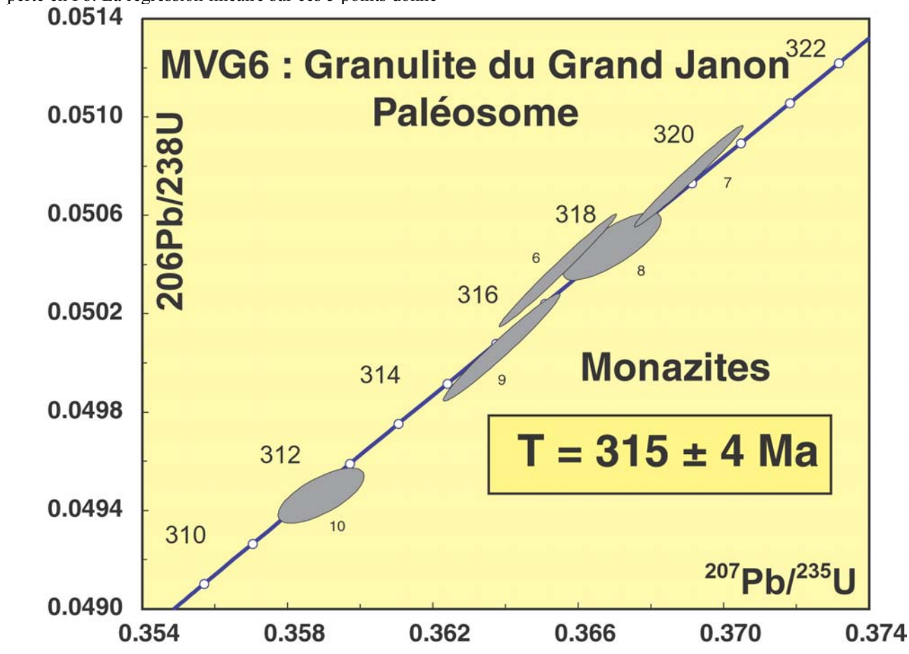
FIG. IV-28- Diagramme concordia du paléosome des granulites du Grand Janon.
