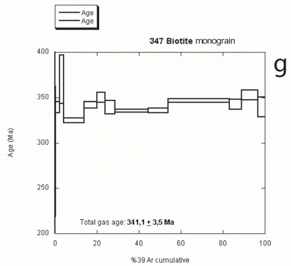
PLANCHE XII – Résultats 40 Ar/ 39 Ar effectués sur les gneiss à biotite-sillimanite (échantillon 241, 40 et 347) de la zone de cisaillement de St Michel de Veisse Felletin-La Courtine.
