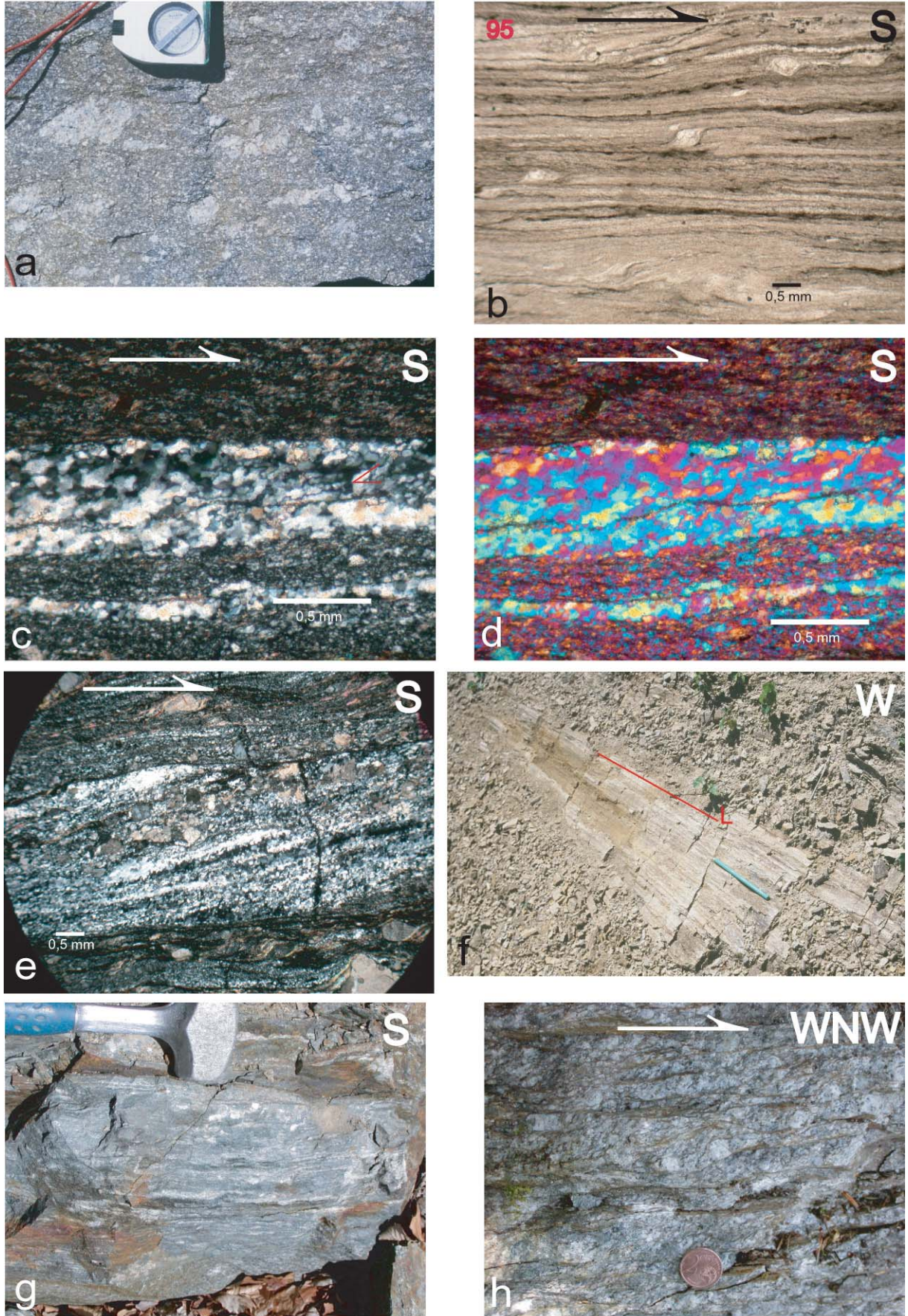
PLANCHE III - Microstructures observées dans les granites à biotite (type Guéret) au sein de la zone de cisaillement de Felletin-La Courtine à l'échelle du macroéchantillon et de la lame mince. a : Phénocristaux de feldspath potassique centimétriques. b : Echantillon 95. Faciès ultramylonitique. c : Echantillon 95. Rubans de quartz en lumière naturelle avec fabrique de forme oblique de 35 à 40° par rapport au plan de cisaillement. d : Echantillon 95. Rubans de quartz à grains obliques montrant une fabrique par ajout de la lame onde. e : Echantillon 95. Microplis d'entraînement formés par les rubans de quartz. f : Linéation horizontale bien exprimée dans les faciès mylonitiques. g : Faciès des granites à proximité de la carrière de Clairavaux. h : Echantillon 375. Microstructures C-S mettant en évidence le mouvement décrochant dextre.
