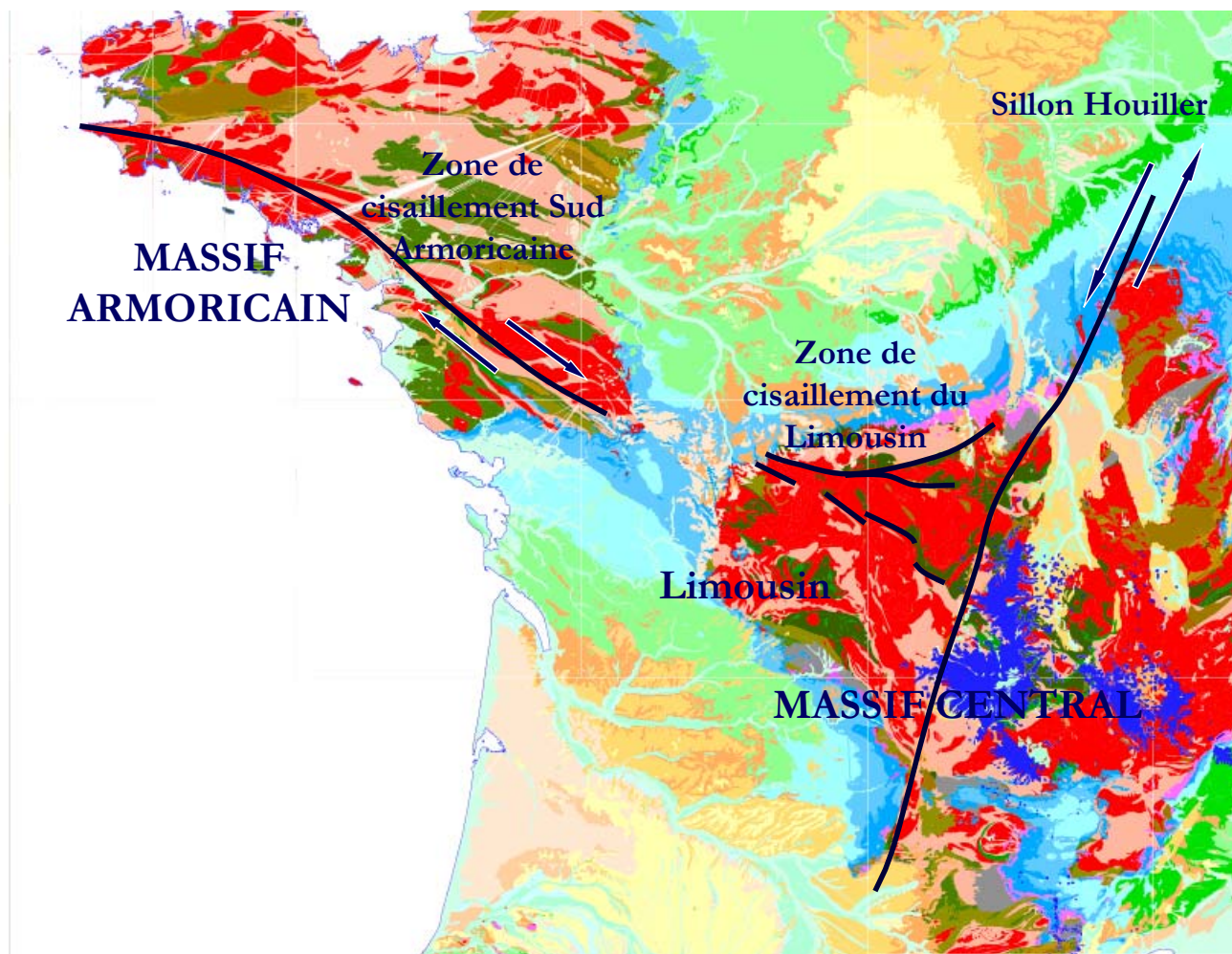
FIG. III-1 – Carte géologique de la France au 1 : 1 000 000 (BRGM) mettant en évidence les relations entre les zones de cisaillements du Limousin et la zone de cisaillement Sud Armoricaïne.
