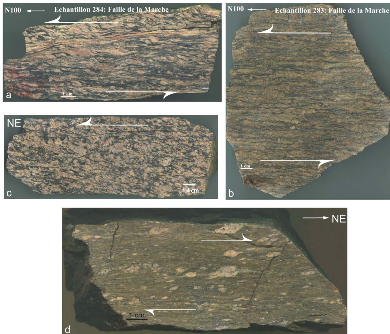
PLANCHE XIX – Photographies montrant les microstructures des leucogranites et des gneiss à biotite-sillimanite affectés par l'accident de la Marche à l'échelle du macro échantillon. a : Échantillon 284. Leucogranites mylonitiques avec passées ultramytonitiques prélevés au sud de Dun-le-Palestel sur la D5. La déformation est très pénétrative et les critères de cisaillement sont sénestres. F : N100-90°, L : N100-0° b : Échantillon 283. Leucogranites situés à 500m au nord du précédent. La déformation est moins intense et les critères de cisaillement sont moins significatifs F : N080-65SE, L : N100-30°. c : Échantillon 334. Leucogranites provenant de la Marche occidentale, vers Cromac (Moulin de Réculais). Les microstructures C-S indiquent un mouvement en faille inverse vers le NE. d : Échantillon 333. Gneiss à biotite-sillimanite indiquant un mouvement en faille inverse vers le NE (Cromac).
