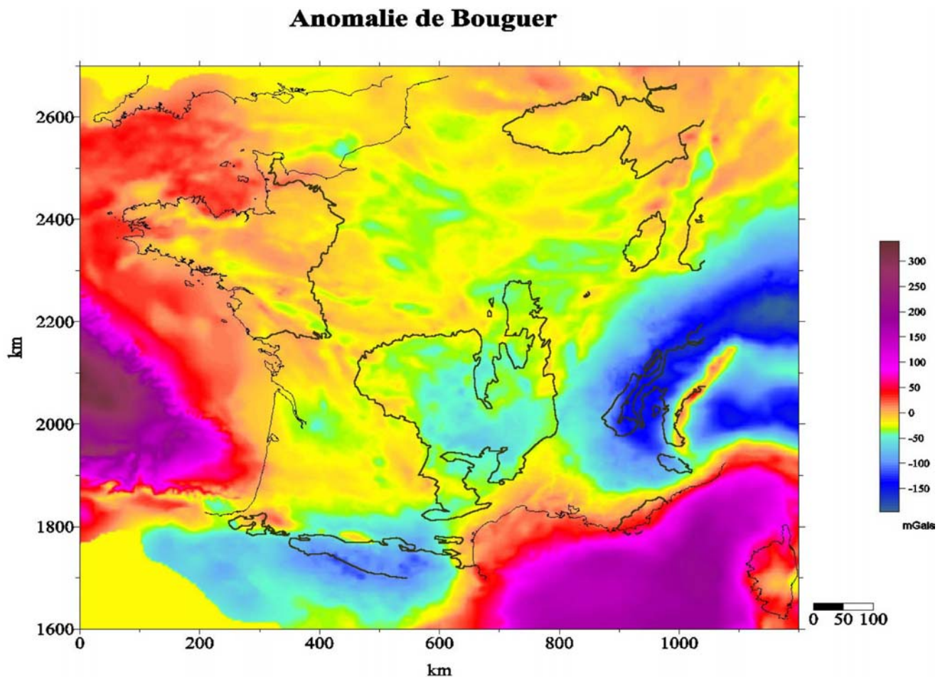
FIG. II-7 – Carte d'anomalie de Bouguer à l'échelle de la France d'après GRANJEAN et al. , 1998.
