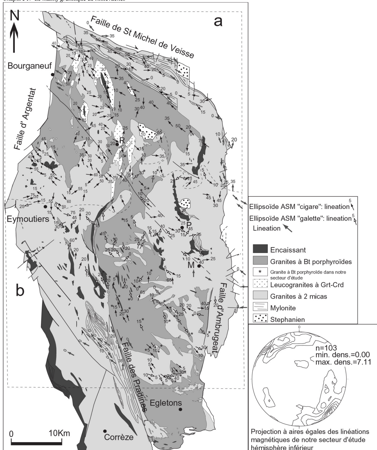
FIG. IV-25 – Carte des linéations magnétiques du massif de Millevaches. a) Données de Jover (1986). b) Notre secteur d'étude
