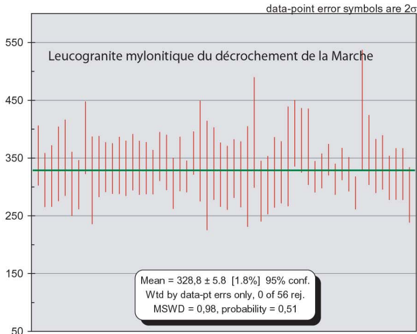
Fig. III-12a : Moyenne pondérée des âges individuels et barres d'erreur de l'échantillon 284.
