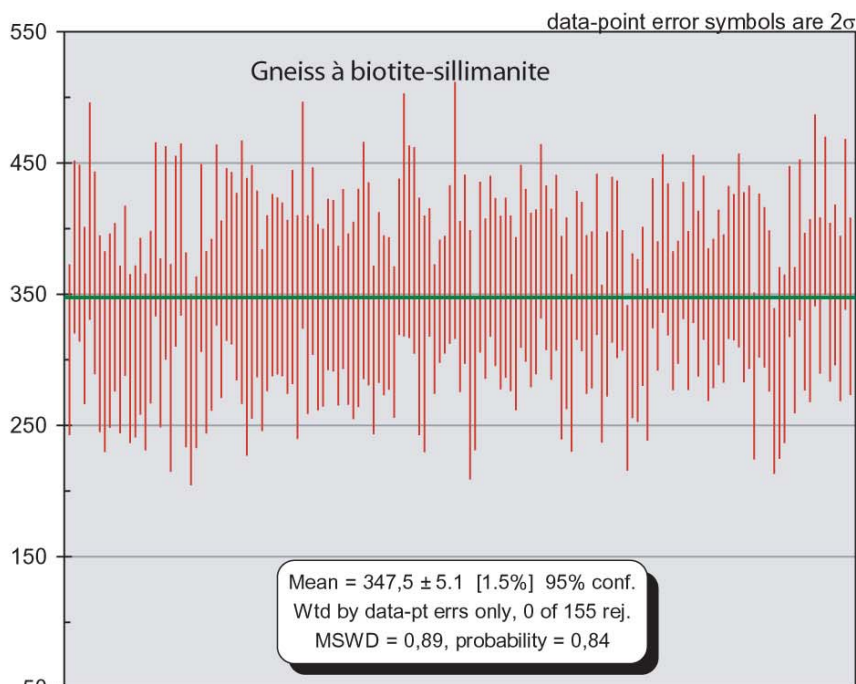
Fig. III-6 a : Moyenne pondérée des âges individuels et barres d'erreur de l'échantillon 381.
