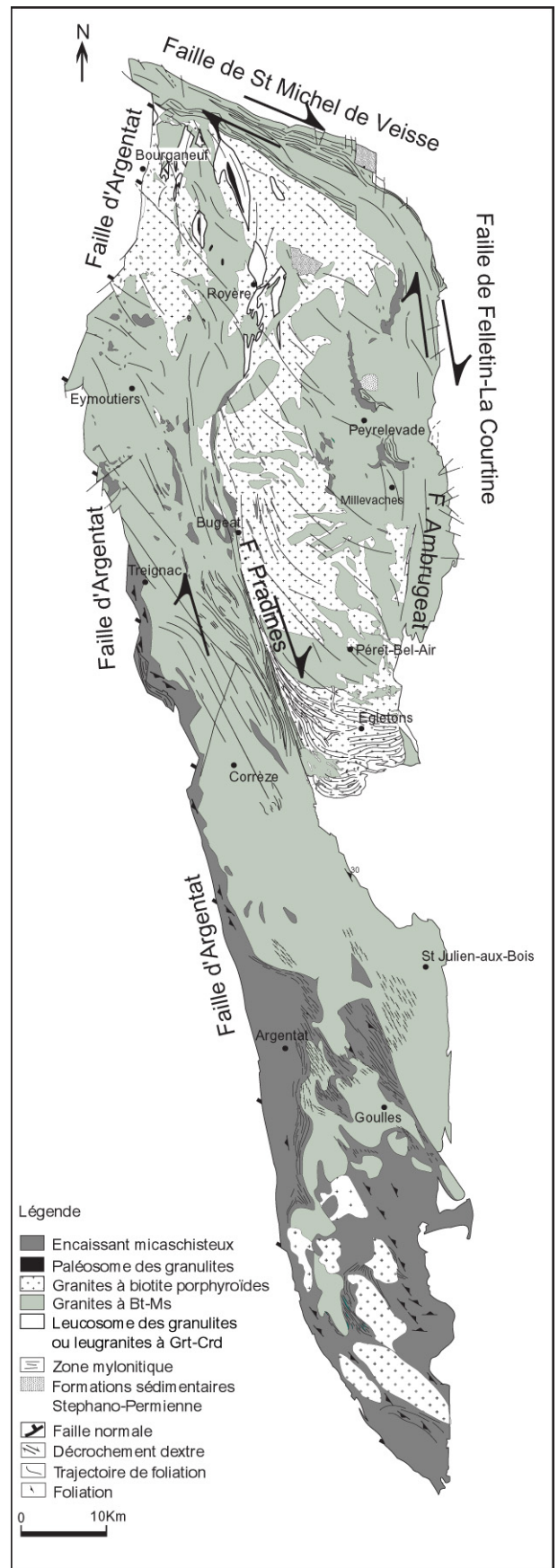
FIG. V-1 – Carte pétrostructurale du massif de Millevaches.
