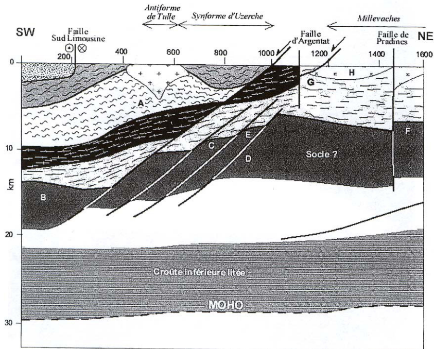
FIG. III-11 – Interprétation du profil sismique d'Argentat d'après BITRI et al. (1999). A: Unités gneissiques. B, C, D, E, F, G: Unités discordantes. G: Micaschistes. H: Leucogranites du Millevaches.
