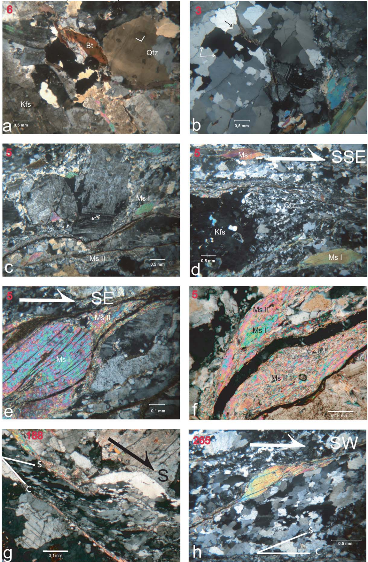
PLANCHE II - Microstructures dans les leucogranites de bordure du massif de Millevaches à l'échelle de la lame mince. a : Quartz en « échiquier ». b : Quartz en mosaïque (joints de grain à 90°). c : Fracturation et déformation plastique des feldspaths. d : Recrystallisation intense du quartz et du feldspath dans les ombres de pression des feldspaths potassiques. e : Développement de muscovites secondaires syncisaillement dans les queues de recrystallisation des muscovites primaires. f : Phénomène de recrystallisation de muscovites secondaires généralisé à partir des muscovites primaires magmatiques. g : Micro zone de cisaillement avec développement des grains de quartz à 40°C du plan de cisaillement. h : Migration intense aux joints de grain des quartz avec micafish dextre indiquant un mécanisme en faille inverse vers le SW..
