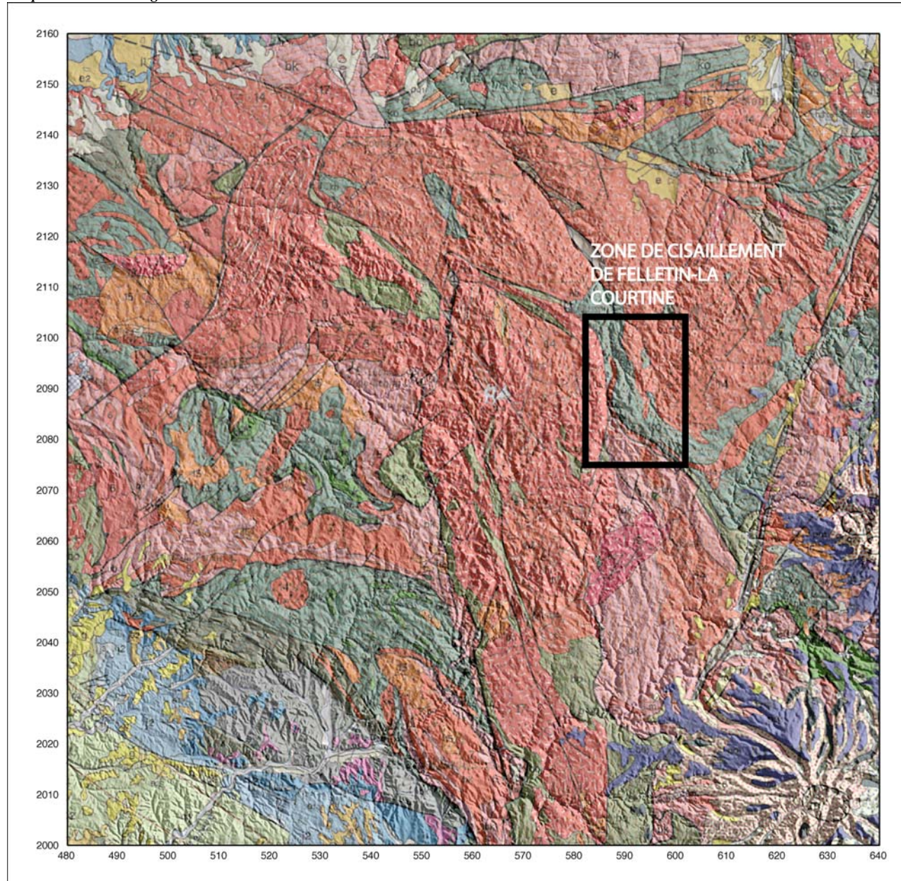
FIG. II-1 – Modèle Numérique de Terrain au 1 : 1 000 000 (BRGM) montrant la localisation de la zone de cisaillement de Felletin-La Courtine cartographiée.
