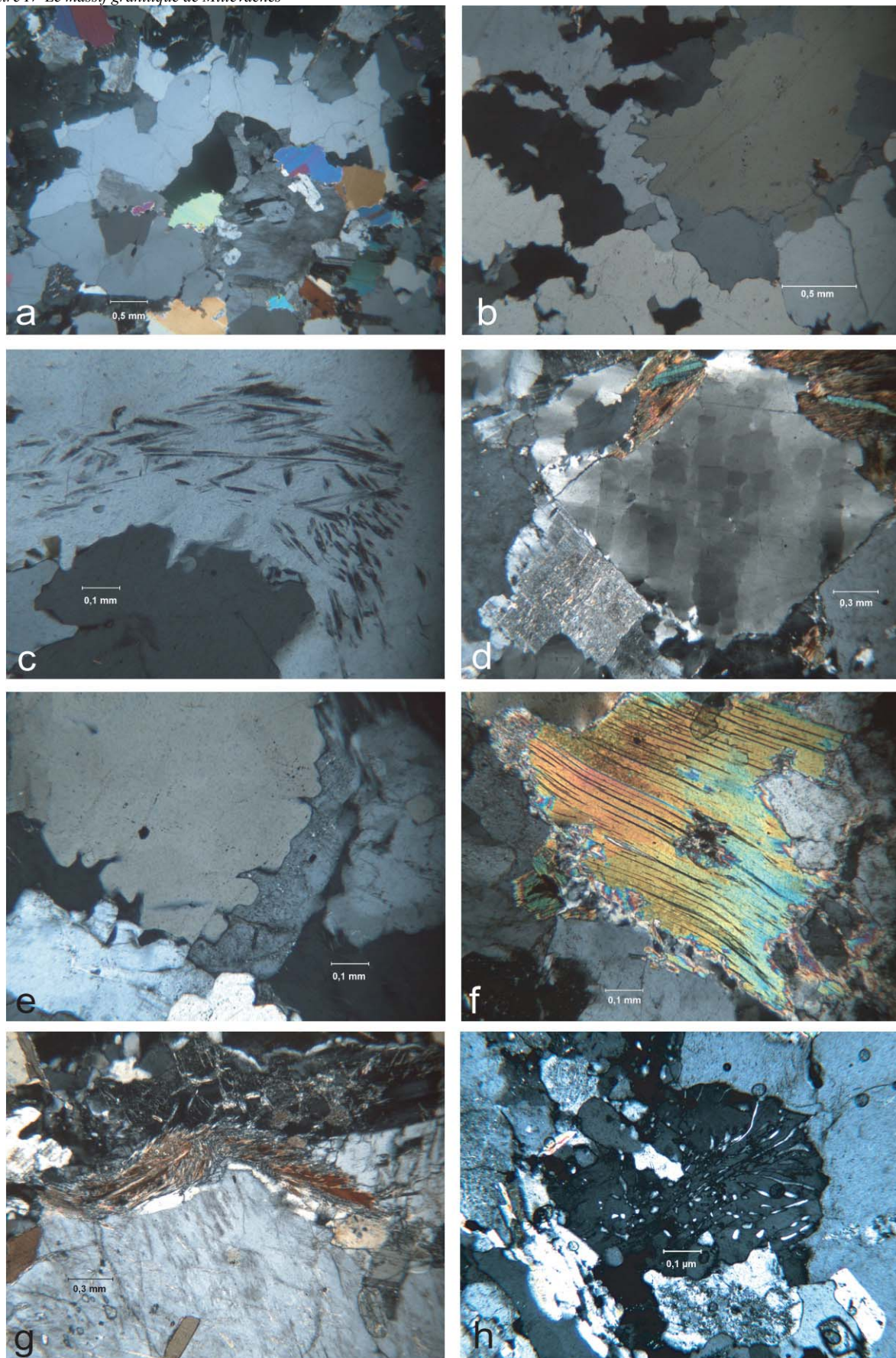
PLANCHE XXVIII- Microstructures des granites à deux micas observées parallèlement à la linéation magnétique. a :Microstructures magmatiques montrant des grains de quartz à extinction franche. b : Migration au joints de grain de quartz. c : Sillimanites prismatiques en inclusion dans les quartz. d : Quartz en échiquier où les sous joints basaux et prismatiques \langle c \rangle sont bien mis en évidence. e : Géométrie curviligne entre quartz et feldspath se développant dans des conditions de haute température (650°C-750°C). f : Muscovite froissée qui s'effectue dans le continuum magmatique. g : Association sillimanite-biotite dans les plans de cisaillement entre les feldspaths potassiques. h : Présence fréquente de myrmékites.
