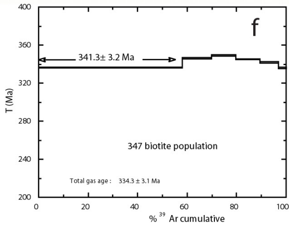
PLANCHE XII – Résultats 40 Ar/ 39 Ar effectués sur les gneiss à biotite-sillimanite (échantillon 241, 40 et 347) de la zone de cisaillement de St Michel de Veisse Felletin-La Courtine.
