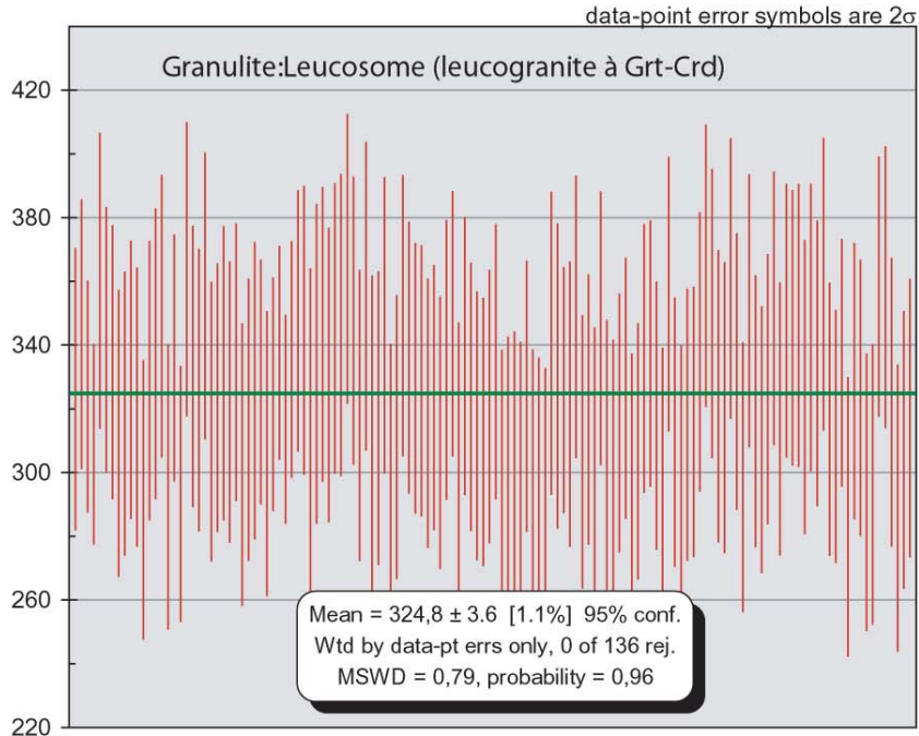
Fig. IV-33a : Moyenne pondérée des âges individuels et barres d'erreur de l'échantillon 487.
