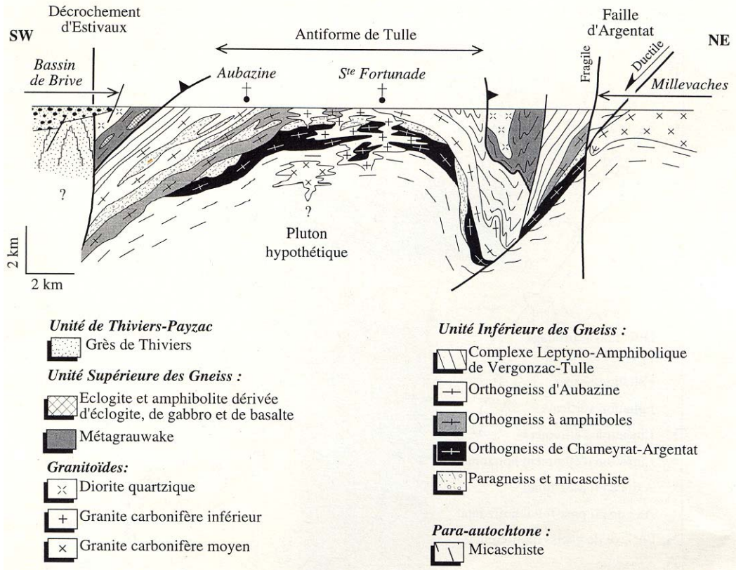
FIG. III-10 – Coupe à travers l'antiforme de Tulle et l'ouest du massif granitique de Millevaches mettant en évidence le jeu normal de la faille d'Argentat d'après ROIG et FAURE (2000).
