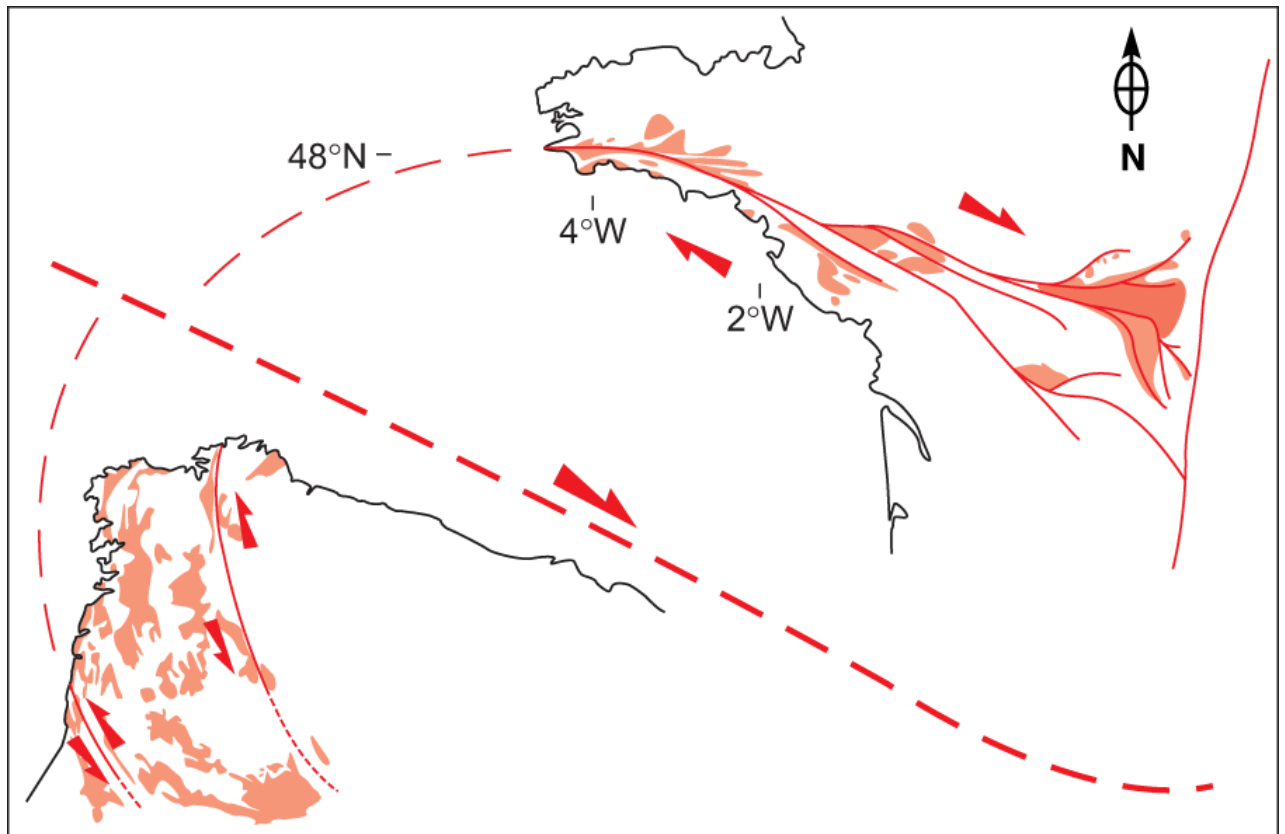
FIG. V-8 : Prolongement possible de la « pop-up structure » en Galice.
