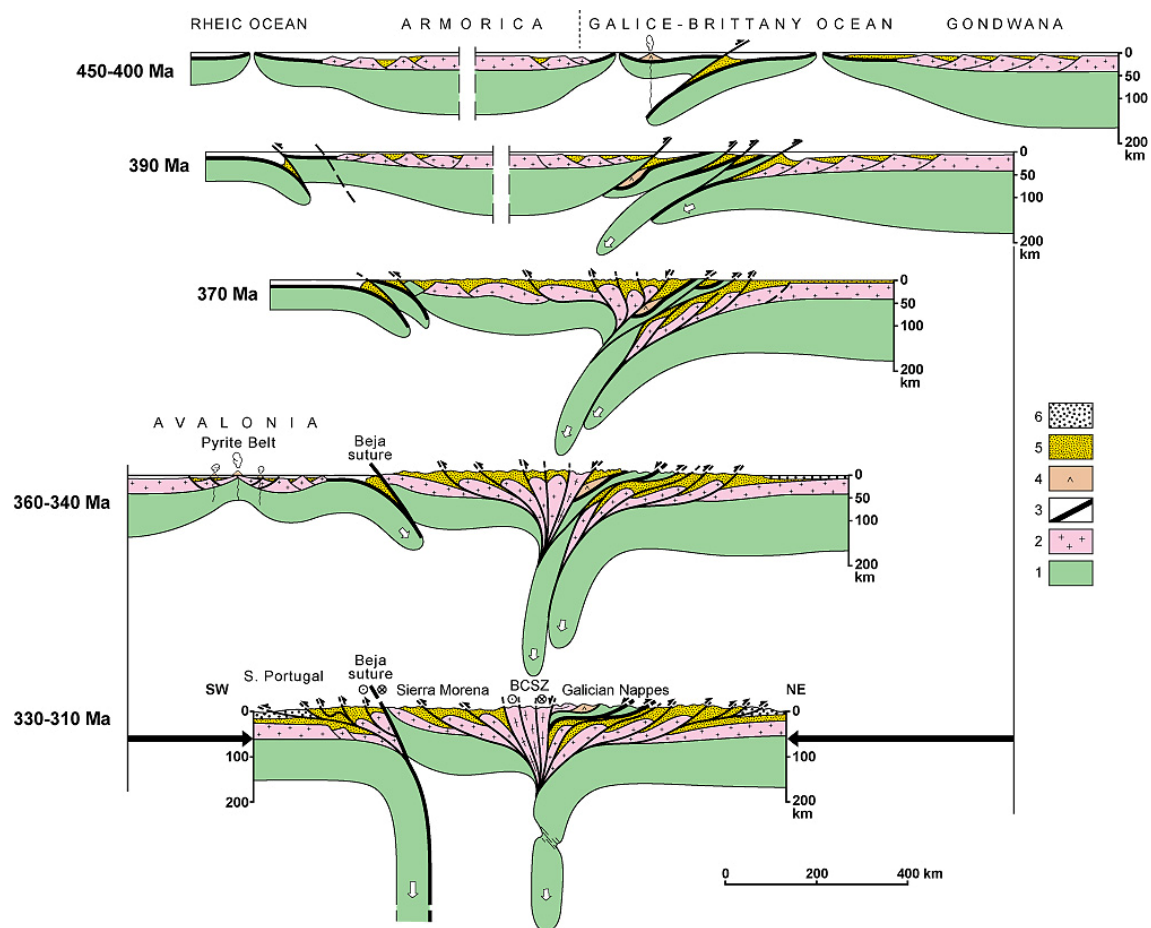
FIG. I-8– Modèle d'évolution monphasé de la Chaîne Varisque d'Europe sur la transversale Ibérique depuis l'ordovicien jusqu'au Carbonifère, d'après MATTE (2002). 1 : Manteau. 2 : Croûte continentale. 3 : Croûte océanique. 4 : Croûte d'arc possible. 5 : Sédiments Paléozoïques. 6 : Bassins Carbonifères.
