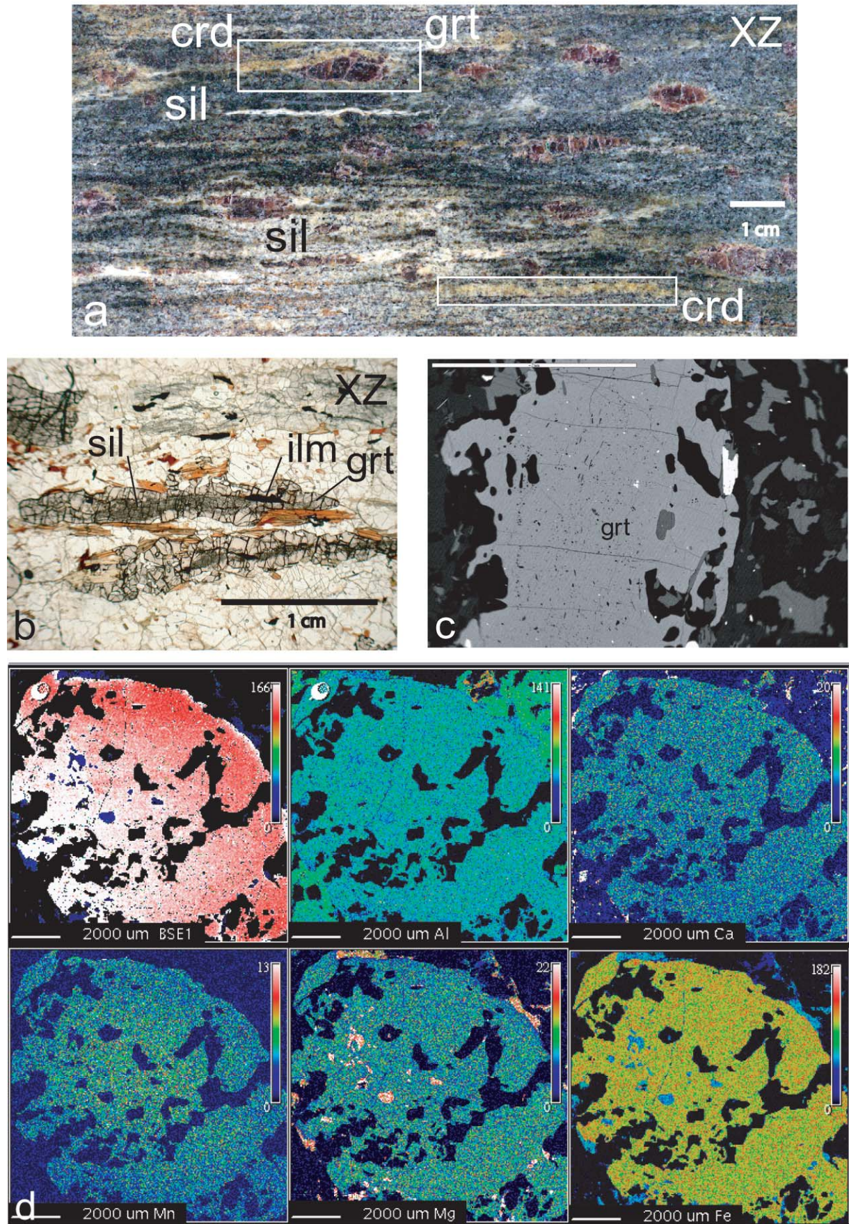
PLANCHE XXV -Les formations granulitiques du hameau du Grand Janon à proximité de St Pierre-Bellevue (Nord du Millevaches). a. Aspect macroscopique des granulites sur un échantillon scié. Les grenats, les cordiérites et les sillimanites forment des rubans. b. Rubans de grenats en lame mince. Notons que les inclusions de sillimanite (halo gris sombre à l'intérieur du grenat) sont plus nombreuses au cœur qu'à la périphérie. La sillimanite est également observée dans la trame de la roche. c. Bordure du grenat curviligne au MEB. Croissance dendritique suggérant une croissance rapide. d. Cartographie d'éléments faite à la microsonde électronique SX 100 de Montpellier d'un grenat ne montrant aucune zonation significative. Léger enrichissement du cœur en manganèse lié à sa croissance (d).
