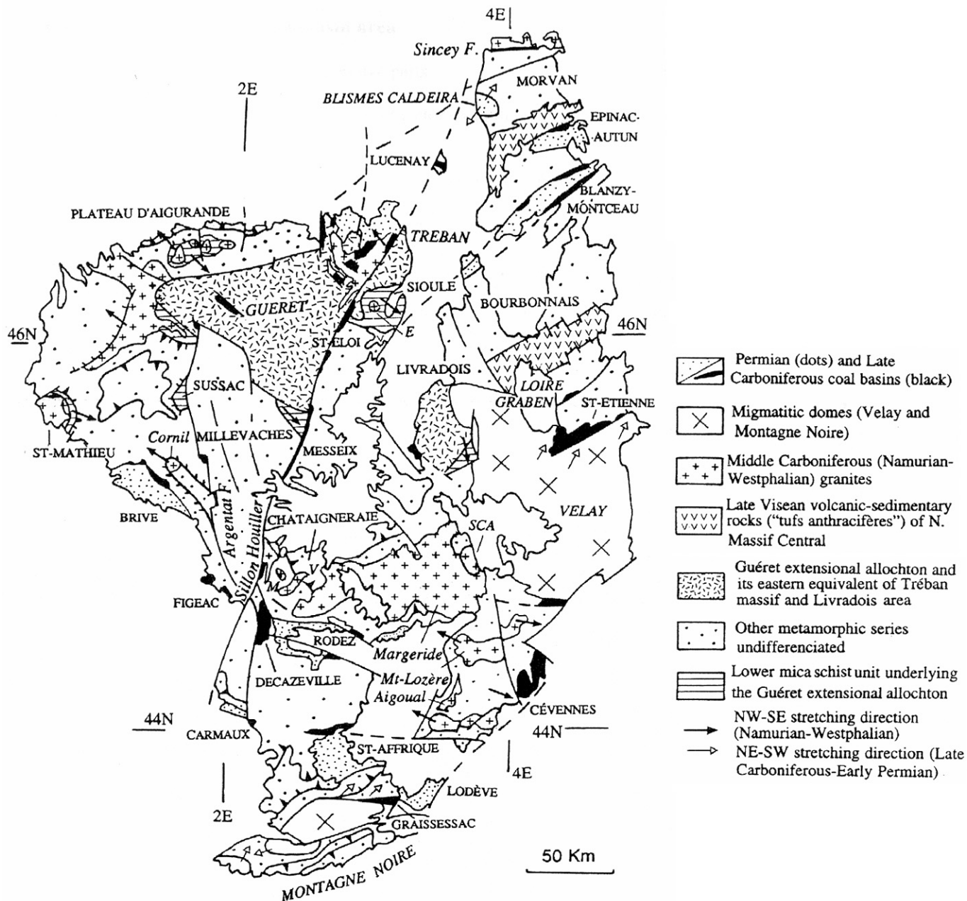
FIG. I-16- Carte générale des structures extensives Carbonifère dans le Massif Central d'après FAURE (1995).
