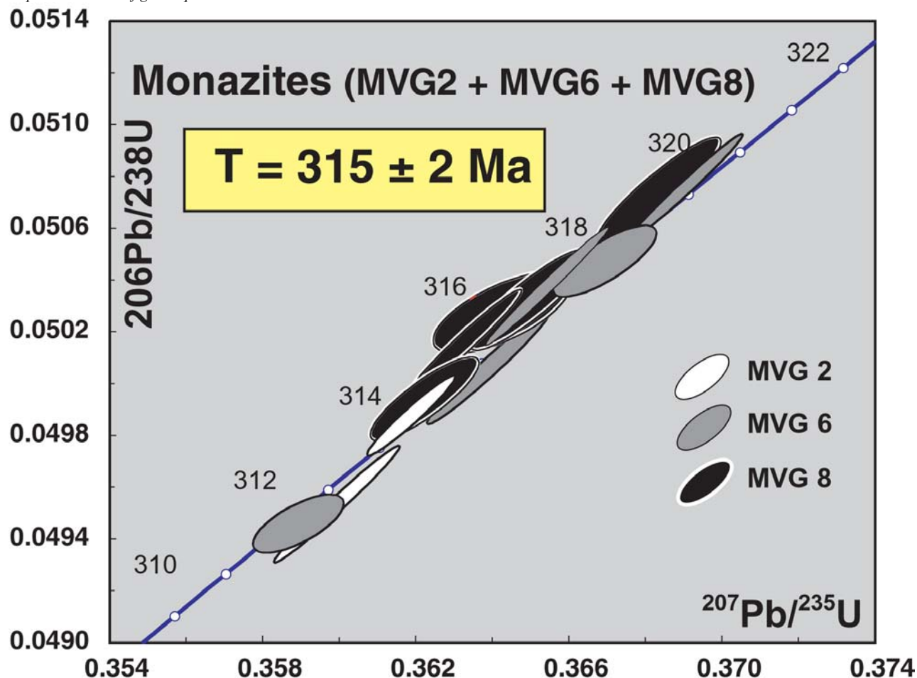
FIG. IV-30– Diagramme concordia récapitulatif
