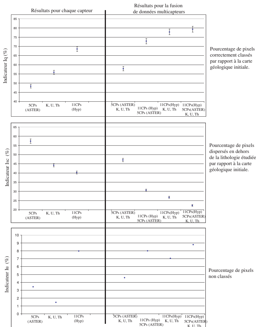
FIG. 4.23 – Indicateurs de qualité I_q , I_{sc} et I_u dans le cas de zones d'apprentissage aléatoires et utilisant : les 5 CPs ASTER, les 3 données de radioéléments, les 11 CPs Hyperion; la fusion des 3 données de radioéléments et des 5 CPs ASTER, la fusion des 5 CPs ASTER et les 11 CPs Hyperion, la fusion des 3 données de radioéléments et des 11 CPs Hyperion, et enfin la fusion des 3 données de radioéléments, des 5 CPs ASTER et des 11 CPs Hyperion.
