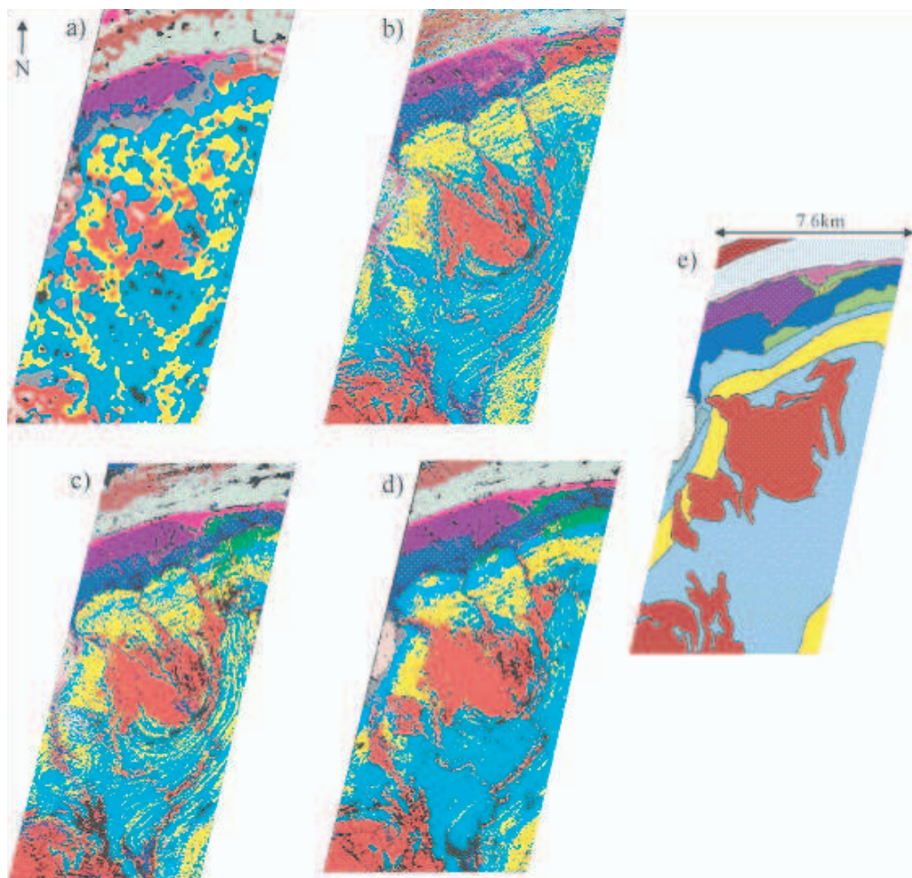
FIG. 4.24 – Résultats de la classification initialisée avec des zones d'apprentissage aléatoires et utilisant : a) les 11 données de radioéléments, b) les 5 CPs ASTER, c) les 11 CPs HYPERION, et d) la fusion des 3 données de radioéléments, des 5 CPs ASTER et des 11 CPs HYPERION. e) Carte géologique initiale. Les surfaces en noir correspondent aux pixels classés dans aucune des 12 lithologies composant la carte géologique.
