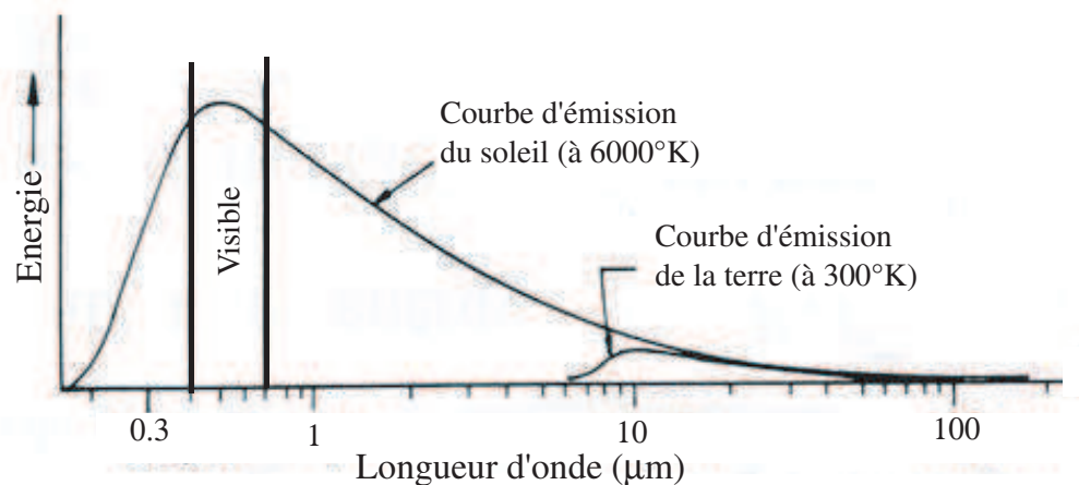
FIG. 2.3 – Courbe d’émission spectrale du REM du soleil (à 6000^\circ\text{K} ) et de la surface de la terre (à 300^\circ\text{K} ).
