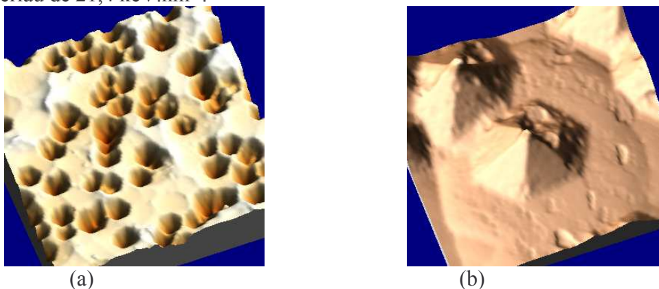
Figure III-11 : Vue du dessus d'une zone de 10\mu\text{m}^2 (a) et représentation tridimensionnelle inversée de la morphologie d'une trace révélée (b) dans une fluoroapatite de Durango irradiée avec des ions Xe ( 21,4 \text{ keV.nm}^{-1} ) et révélée 60 secondes dans \text{HNO}_3 1%.
