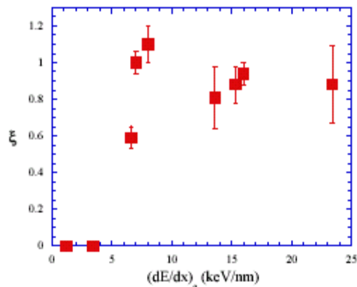
Figure III-17 : Evolution de l'efficacité chimique \xi en fonction du pouvoir d'arrêt électronique dans SiO_2 irradiée avec différents ions lourds et révélée dans HF (d'après Rotaru 04).
