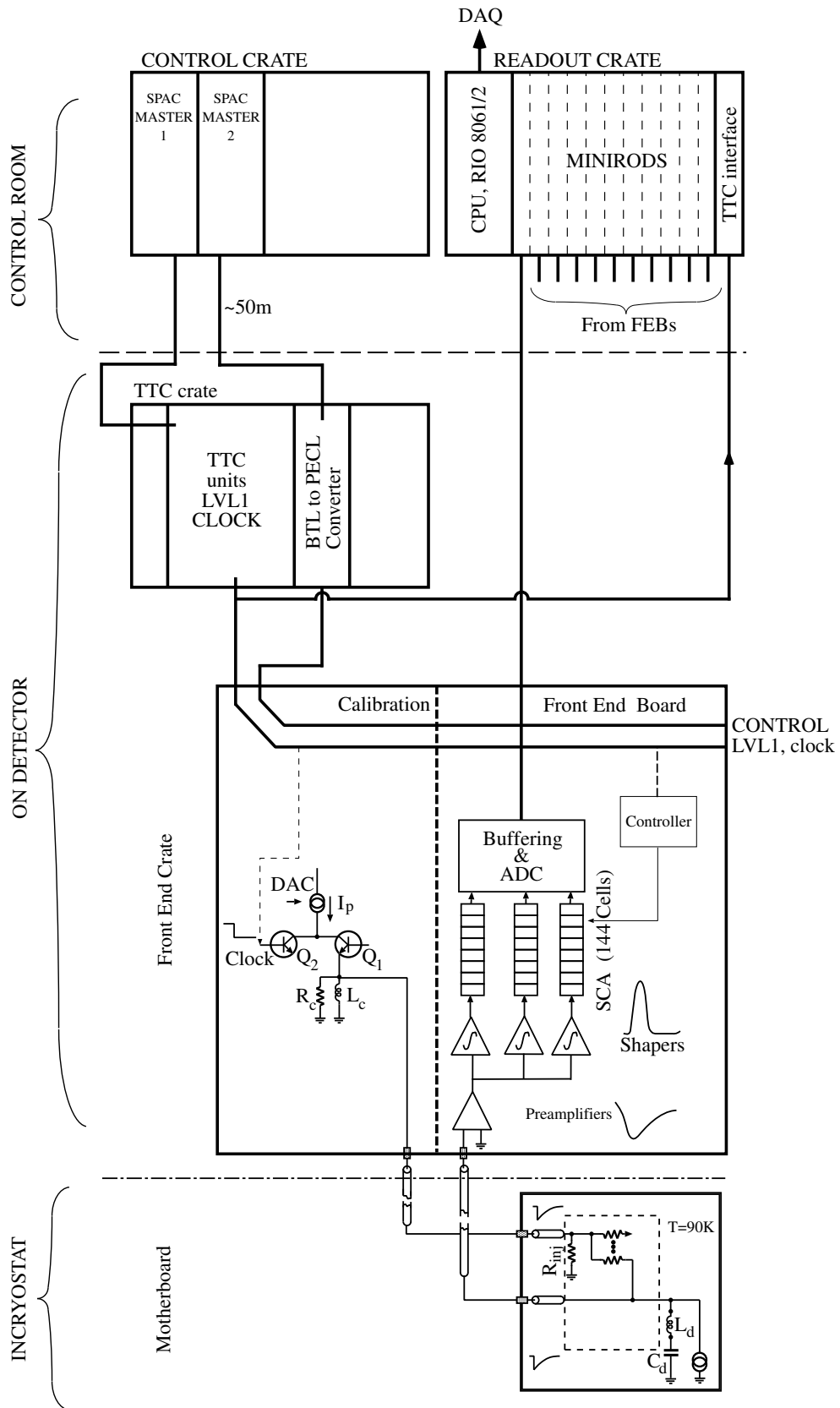
FIG. 4.5 – Schéma de la chaîne de lecture et du système d'étalonnage du calorimètre dans le cadre des tests en faisceau.
