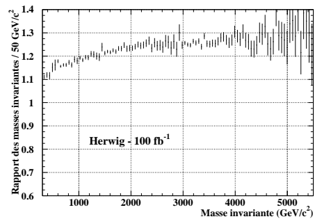
FIG. 6.22 – Rapport des distributions sans et avec radiation de photons, pour HERWIG.
