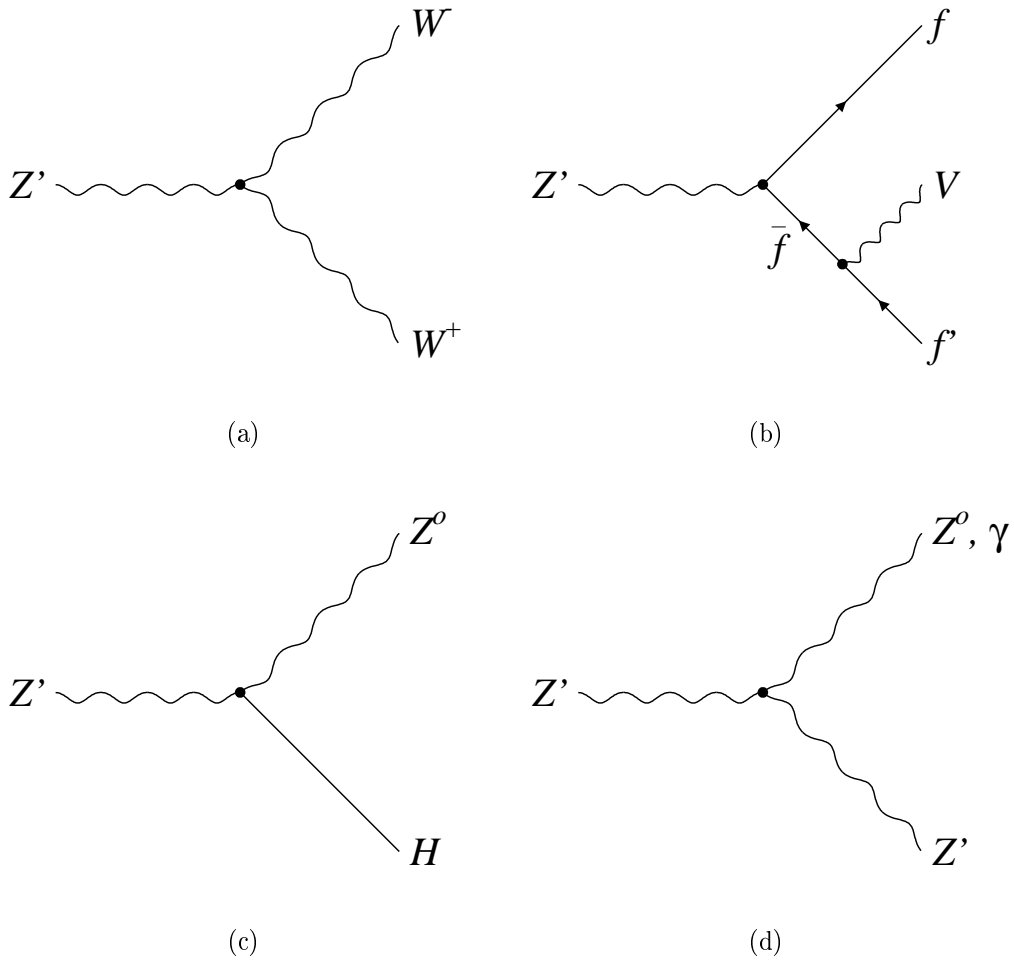
FIG. 1.3 – Modes de désintégration du Z' : (a) Z' \rightarrow W^+ W^- . (b) Z' \rightarrow f \bar{f} V . (c) Z' \rightarrow Z^0 H . (d) Z' \rightarrow Z \gamma .
