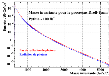
FIG. 6.19 – Distribution de la masse invariante du processus Drell-Yann sans (rouge) et avec (bleu) radiation de photons dans l'état final avec PYTHIA ( 100 \text{ fb}^{-1} ).
