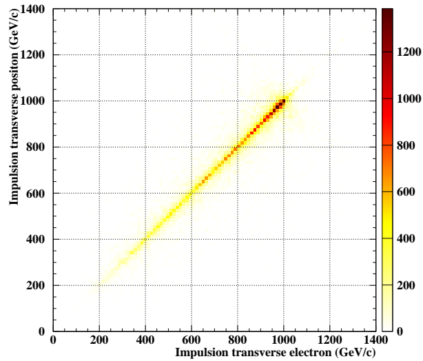
FIG. 6.5 – Impulsion transverse du positon en fonction de l'impulsion transverse de l'électron dans la désintégration électronique d'un Z' de 2 TeV au niveau de la génération.
