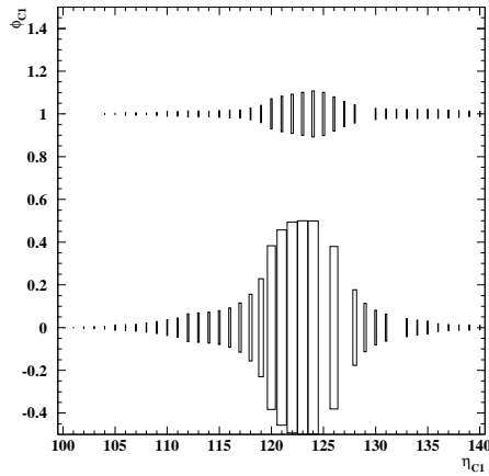
FIG. 5.11 – Distribution de la position du barycentre en \varphi en fonction de \eta dans le compartiment avant. La taille des boites dépend du nombre d'événements pour chaque position.
