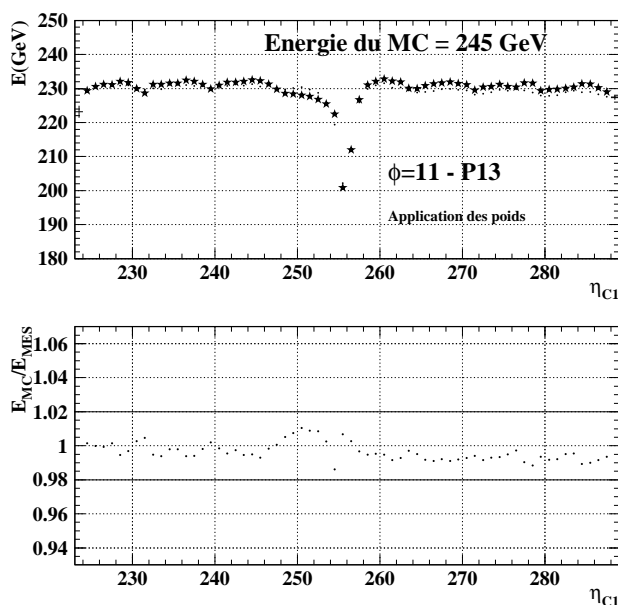
FIG. 5.31 – Figure du haut : profil de l'énergie en fonction de \eta (en unité de cellule du compartiment avant), pour les données (étoiles) et la simulation d'électrons de 245 GeV. Figure du bas : rapport entre les profils de la figure du haut.
