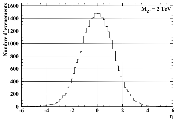
FIG. 6.6 – Distribution en \eta de l'électron issu de la désintégration du Z' .
