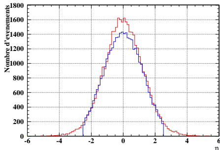
FIG. 6.10 – Distribution en \eta du positon généré par PYTHIA (rouge) et après sa simulation dans le détecteur (bleu). Les coupures d'isolation sur \Delta R_3 et E_{max} sont inhibées.
