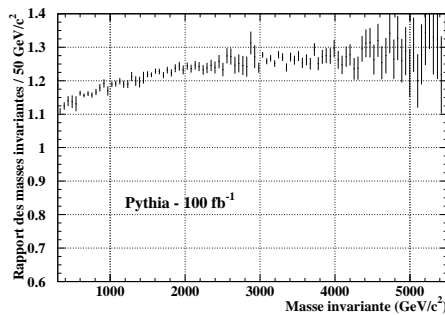
FIG. 6.21 – Rapport des distributions sans et avec radiation de photons, pour PYTHIA.
