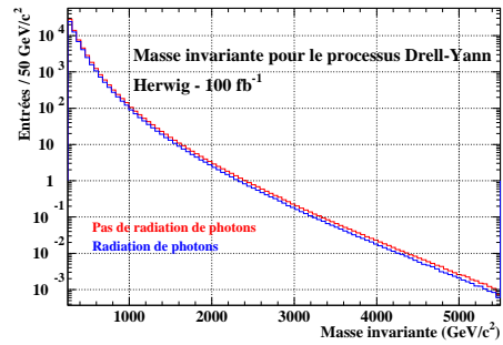
FIG. 6.20 – Distribution de la masse invariante du processus Drell-Yann sans radiation (rouge) et avec (bleu) de photons dans l'état final avec HERWIG ( 100 \text{ fb}^{-1} ).
