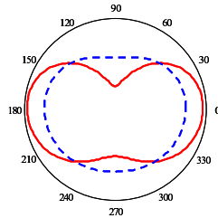
FIG. 4.10 – Projections dans le plan ( \mathbf{X}, \mathbf{Y} ) des fonctions de distributions photoinduites en l'absence de transfert (trait plein) et pour une efficacité de transfert de 50% dans ( \mathbf{X}, \mathbf{Y} ) (pointillés) avec p_1 = p_3 = 0, 3 et p_2 = 0, 15 .
