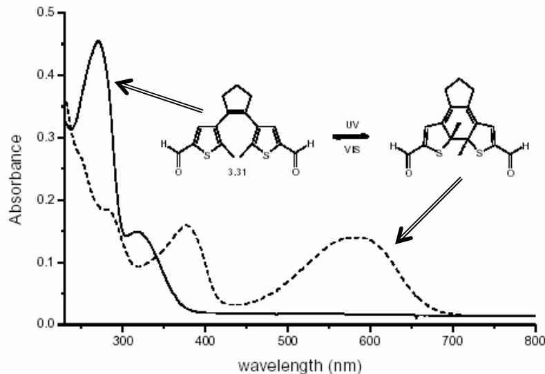
FIG. 2.2 – Spectres d'absorption d'un dérivé du diaryléthène avant (forme ouverte) et après (forme fermée) irradiation à 313nm [68]
