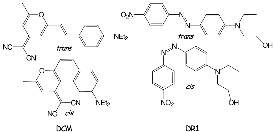
FIG. 2.1 – Exemple de deux molécules photoisomérisables possédant des liaisons doubles C=C ou N=N dans leurs formes cis et trans .
