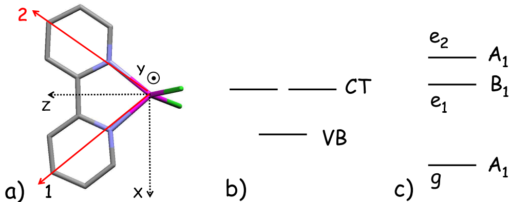
FIG. 7.9 – Représentations schématiques d'une molécule C_{2v} plane présentant deux transferts de charge (dirigés selon les vecteurs 1 et 2) séparés d'un angle de 60^\circ dans le plan (x, z) (a). Niveaux d'énergie de la base du modèle VB-2CT (b) et énergies propres de la molécule indexées selon leurs représentations irréductibles (c).
