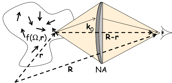
FIG. 1.9 – Représentation schématique du dispositif optique ( NA ) servant à collecter en \mathbf{R} la lumière rayonnée par f(\Omega, \mathbf{r}) . Les cônes dessinés correspondent aux directions d'observations \mathbf{k}_0 collectées. Les photons émis hors de ces cônes n'interviennent pas.
