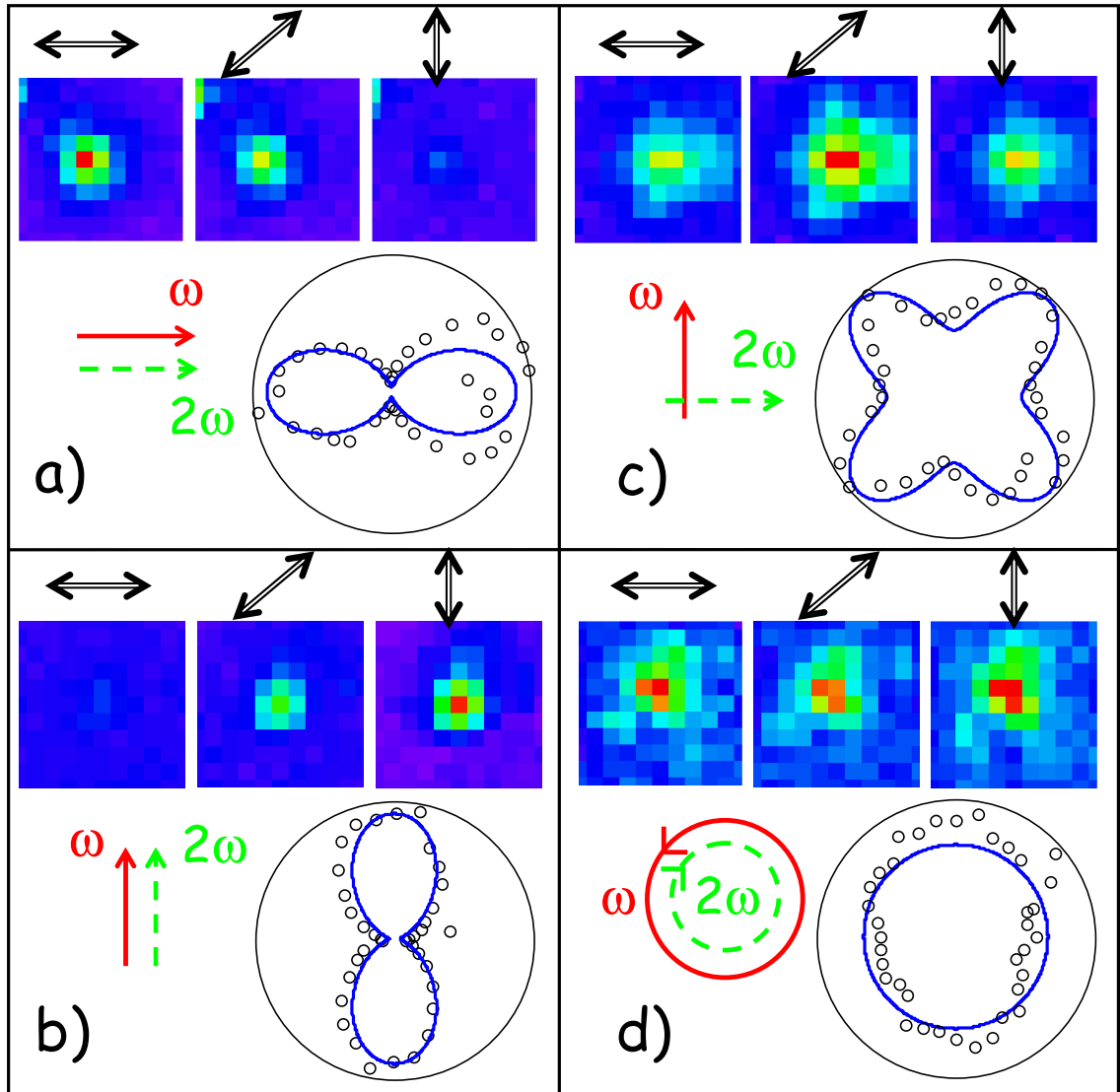
FIG. 6.6 – a) et b) : Réponses en polarisation de l'intensité de SH généré par des zones orientées sur un échantillon de DR1(5%)/PMMA pour des champs linéaires parallèles avec respectivement \hat{\phi}=0^\circ et 90^\circ ( I^\omega = 1,5 J/cm^2 pendant 2 minutes). Les images des intensités de SHG mesurées avec \phi=0^\circ, 40^\circ et 90^\circ permettent d'estimer la résolution spatiale de l'orientation sur l'échantillon de DR1 à 1,5 \mu m (signaux intégrés sur 5s). c) : Réponse en polarisation de l'intensité de SH généré par une zone orientée sur un échantillon de DCM(5%)/PC avec des champs linéaires perpendiculaires ( I^\omega = 2 J/cm^2 pendant 2 minutes). d) : Réponse en polarisation de l'intensité de SH généré par une zone orientée sur un échantillon de DCM(5%)/PC avec des champs contra-circulaires ( I^\omega = 2,5 J/cm^2 pendant 5 minutes). Les images des intensités de SHG mesurées avec \phi=0^\circ, 40^\circ et 90^\circ permettent d'estimer la résolution spatiale de l'orientation sur l'échantillon de DCM à 3 \mu m (signaux intégrés sur 10s).
