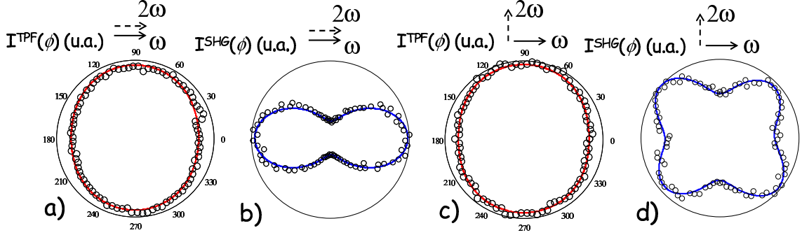
FIG. 6.7 – a) : Réponse en polarisation de l'intensité de TPF d'un échantillon de DCM(5%)/PC après orientation avec des champs linéaires parallèles pour (I^\omega = 0, 2J/cm^2; I^{2\omega} = 0, 4mJ/cm^2) . b) : Réponse en polarisation de l'intensité de SHG d'un échantillon de DCM(5%)/PMMA après orientation avec des champs linéaires parallèles pour I^\omega = 0, 4J/cm^2 . c) : Réponse en polarisation de l'intensité de TPF d'un échantillon de DCM(0, 4%)/PC après orientation avec des champs linéaires perpendiculaires pour (I^\omega = 0, 6J/cm^2; I^{2\omega} = 0, 3mJ/cm^2) . d) : Réponse en polarisation de l'intensité de SHG d'un échantillon de DCM(5%)/PMMA après orientation avec des champs linéaires perpendiculaires pour I^\omega = 0, 6J/cm^2 .
