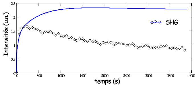
FIG. 5.15 – Dynamique d'évolution des signaux expérimentaux de SHG (losanges) et courbe théorique obtenue en supposant le blanchiment nul (trait continu).
