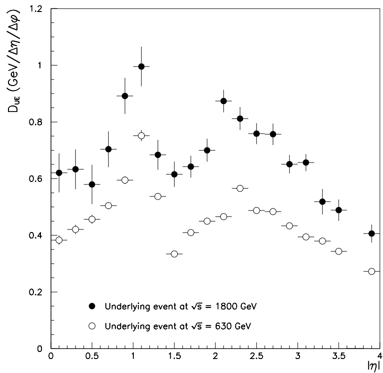
FIG. 5.1 – Densité d'énergie transverse associée aux interactions des partons spectateurs ( D_{UE} ) en fonction de \eta_{det} pour différentes valeurs de l'énergie dans le centre de masse ( \sqrt{s} ) pendant le Run I
