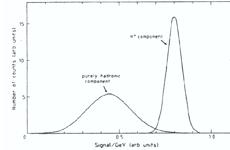
FIG. 2.11 – Réponse du calorimètre pour les composantes électromagnétique ( \pi^0 ) et non-électromagnétique d'une gerbe hadronique.
