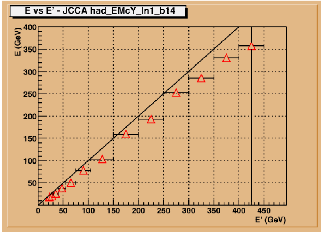
FIG. 6.8 – Corrélation entre E_{jet} et E' pour des événements photon + bjet
