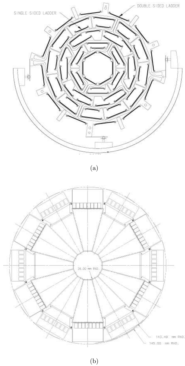
FIG. 2.4 – Coupe transverse d'un segment cylindrique (a) et d'un disque F du SMT (b).
