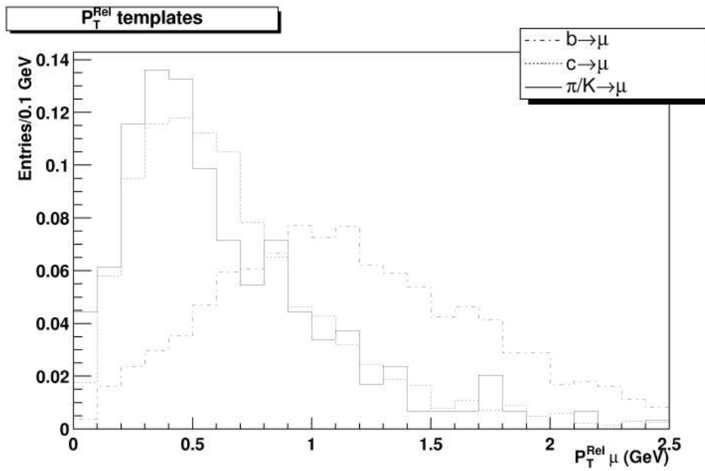
FIG. 4.11 – Distribution du P_{Trel} pour le muon dans 3 jeux événements Monte-Carlo
