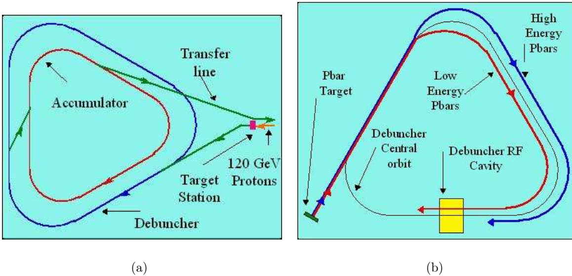
FIG. 1.8 – Principe de fonctionnement du Debuncher et de l'Accumulateur(a) et différentes trajectoires dans le Debuncher en fonction de l'impulsion (b).
