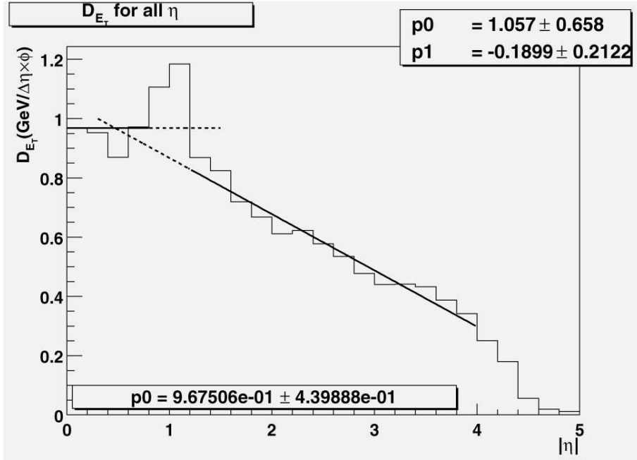
FIG. 5.4 – Ajustement de la distribution d'énergie transverse en fonction de \eta_{det} implémentée dans JetCorr 2.0 pour les données.
