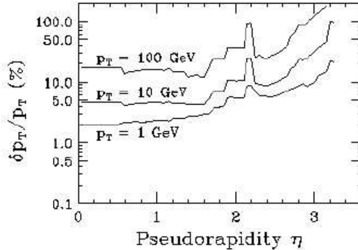
FIG. 2.7 – Résolution en P_T du détecteur interne (SMT + CFT) en fonction de \eta pour 3 valeurs de P_T (1, 10 et 100 GeV ).
