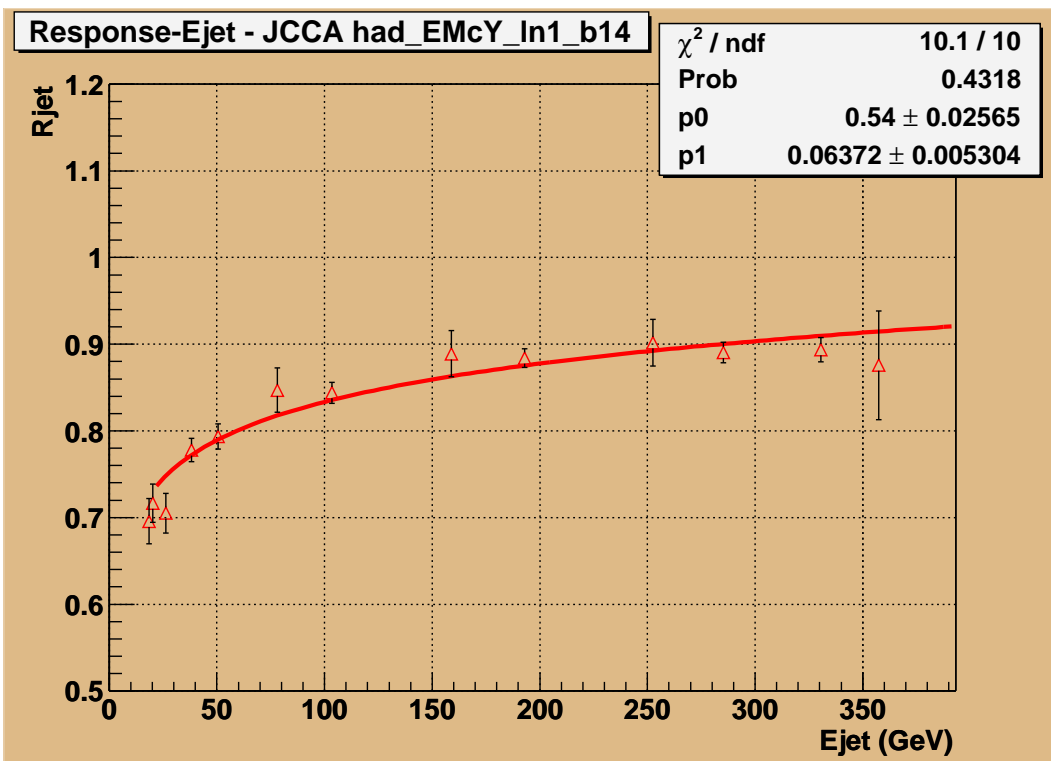
FIG. 6.9 – Réponse en fonction de l'énergie mesurée du jet pour la partie centrale et sur l'avant dans des événements photon + bjet (mode hadronique).
