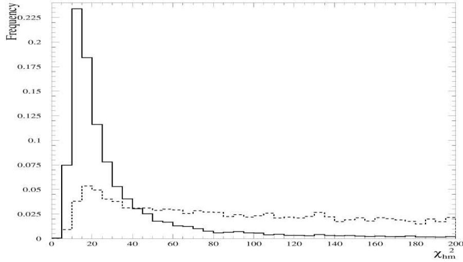
FIG. 4.5 – Distributions du \chi_{hm}^2 pour des électrons dans des événements candidats Z \rightarrow e^+e^- (trait plein) et pour des faux électrons reconstruits dans des données sélectionnées en ligne avec plusieurs jets (pointillés) (pour la partie centrale du calorimètre).
