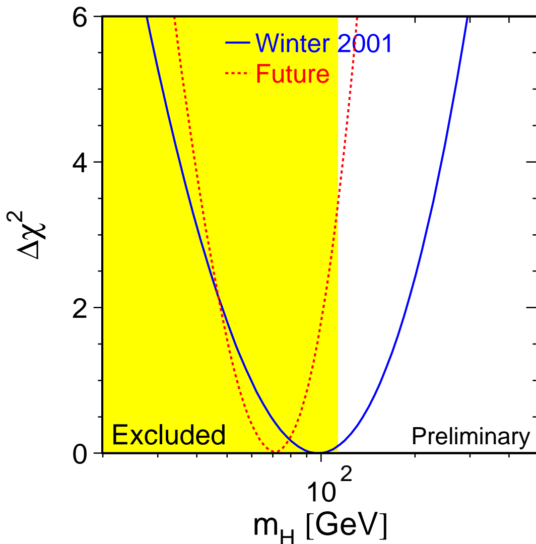
FIG. 1.11 – Prédiction actuelle de la masse du Higgs dans le cadre du modèle standard obtenue à partir des masses mesurées du quark top et du boson W comparé avec la prédiction obtenue en supposant une luminosité de 15 \text{ fb}^{-1} . L'amélioration attendue de la précision sur la masse de ces particules conduit à une diminution d'environ la moitié de la largeur de cette courbe [12].
