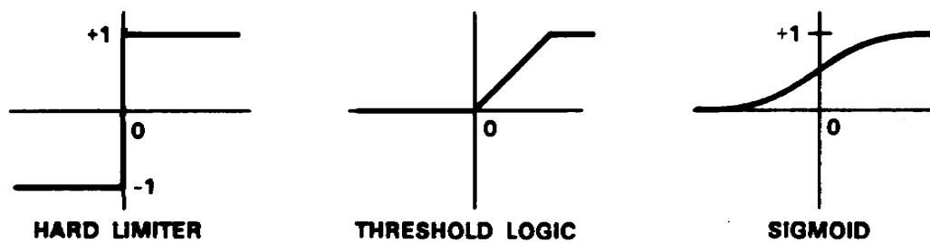
FIG. 1.16 – Quelques fonctions de seuils.
