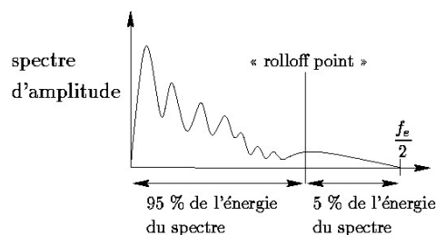
FIG. 1.7 – Définition du « Spectral Rolloff Point ».
