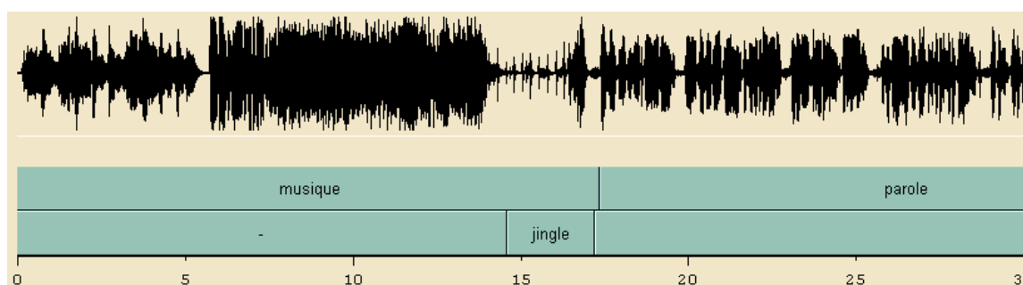
FIG. 4.8 – Exemple de partitionnement bas niveau : (a) classification parole/musique, (b) détection de jingle.
