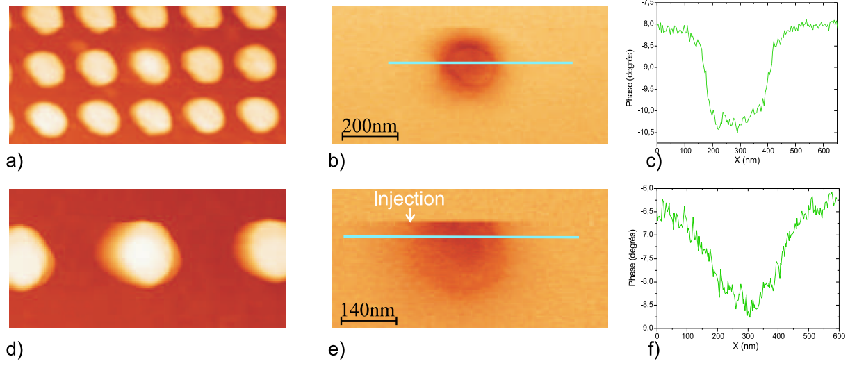
FIG. 4.4: Influence de l'épaisseur d'oxyde sur le chargement des nanostructures lithographiées. Les paramètres d'injection sont -8 \text{ V}/5 \text{ s} . Figures du haut : échantillon avec un oxyde mince de 7 \text{ nm} . a) : Signal AFM, topographie. b) : Signal EFM. c) : Profil EFM sur le diamètre de la tache EFM. Figures du bas : échantillon avec un oxyde épais de 400 \text{ nm} . d) : Signal AFM, topographie. e) : Signal EFM. f) : Profil EFM sur le diamètre de la tache EFM. Les deux échantillons présentent les mêmes caractéristiques de chargement avec une variation de phase au maximum de 2 degrés environ.
