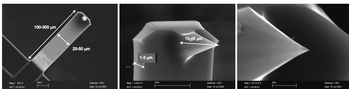
FIG. 1.5: Images MEB d'une sonde AFM utilisée dans le cadre de ce travail, avec agrandissements successifs. Les dimensions caractéristiques des leviers sont indiquées sur la figure. Pour ce levier, les dimensions L \times w \times e = 130 \times 35 \times 1 sont telles que la raideur est de l'ordre de 0,7 \text{ N.m}^{-1} et la fréquence de résonance de l'ordre de 83 kHz.
