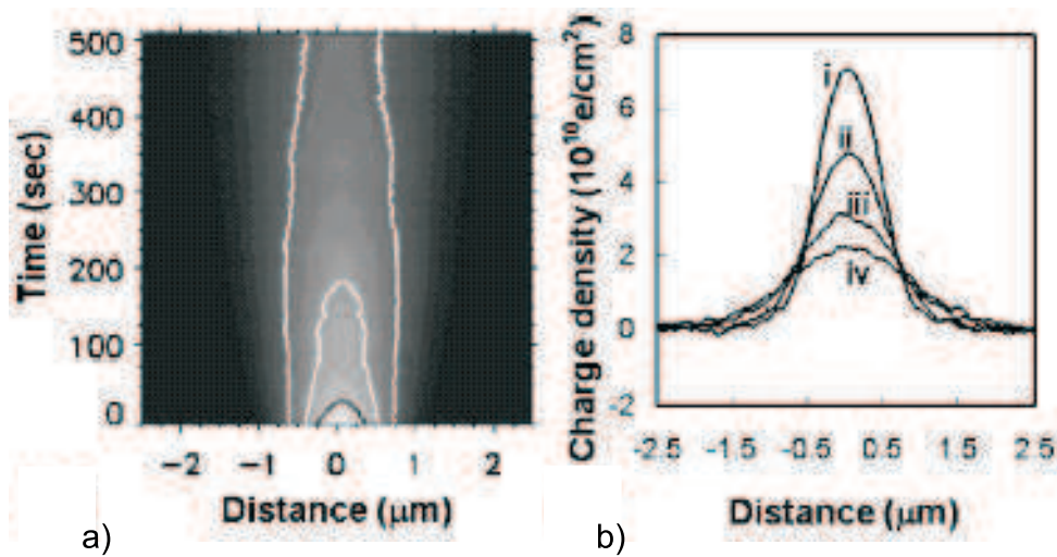
FIG. 4.1: Evolution temporelle d'un paquet de charges sur SiO 2 . Les conditions d'injection sont +10 V/10 s. a) : Evolution du diamètre de la tache de charge. Les contours représentent les 25%, 50% et 75% du maximum du signal. b) : Profils du signal EFM après 0(i), 50(ii), 256(iii) et 512(iv) secondes. D'après [127].
