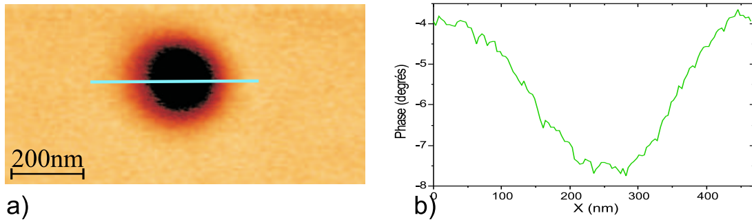
FIG. 4.14: Comportement au chargement de l'échantillon E3. Les conditions de chargement sont -8\text{ V}/0,5\text{ s} . a) : Image de signal EFM. La tache de charge est un disque centré sur le point d'injection. b) : Profil de l'image EFM montrant la distribution homogène des charges.
