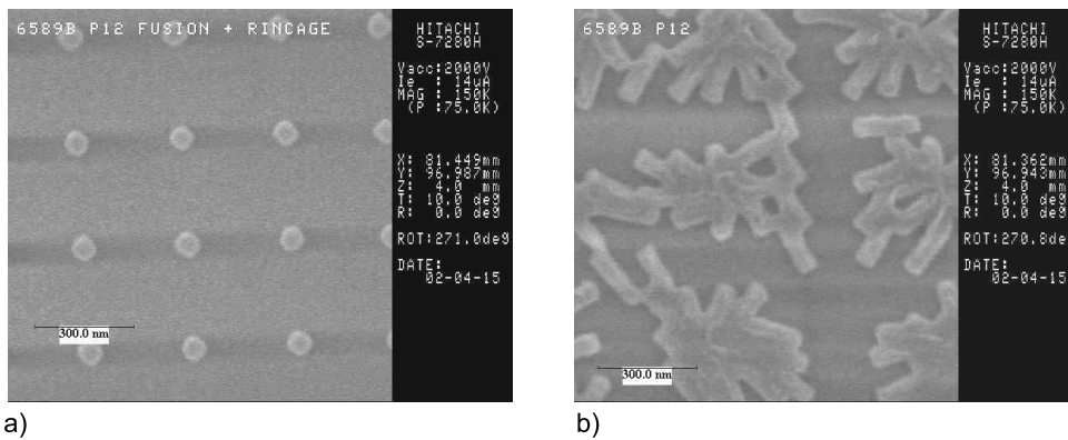
FIG. 3.10: Clichés de microscopie à balayage des plots fabriqués par lithographie à faisceau d'électron. a) : Image MEB des plots de 75 nm espacés de 225 nm. b) : Image MEB des plots de 50 nm espacés de 75 nm : les motifs ne sont pas reconnaissables. On attribue cette configuration en bâtonnets de 200 nm de long agglutinés par amas à la résine qui s'est couchée lors du développement.
