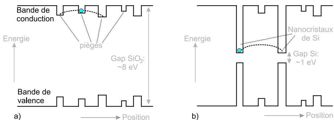
FIG. 4.21: Diagrammes énergétiques de 2 types d'échantillon. a) : Échantillon de référence. Les électrons injectés sont piégés dans des défauts de l'oxyde. La faible profondeur du puits énergétique ainsi que la forte densité de ces pièges permet aux charges de s'évacuer rapidement, soit par la bande de conduction soit par effet tunnel d'un piège vers son voisin. b) : Échantillon de nanocristaux de silicium. Les électrons injectés, même s'ils sont d'abord piégés par les défauts de l'oxyde, rejoignent les sites de nanocristaux qui leur sont énergétiquement plus favorables. De là ils ne peuvent plus rejoindre la bande de conduction. Le passage par effet tunnel au nanocristal voisin dépend de la densité de nanocristaux.
