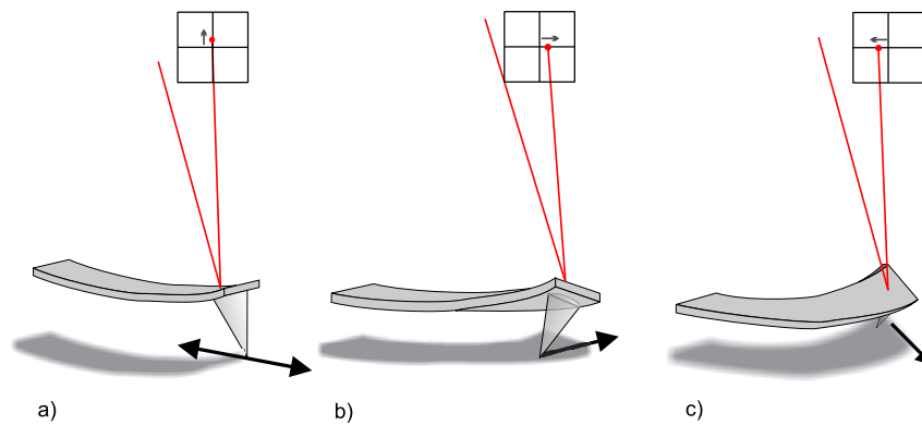
FIG. 1.8: a) : En mode contact normal, le cantilever balaye la surface parallèlement à son grand axe. La déflexion sur la photodiode est verticale. b) et c) : En mode friction, le cantilever balaye perpendiculairement à son grand axe, il se tord, provoquant une déflexion horizontale (A+C)-(B+D) sur la photodiode. La différence entre l'aller et le retour constitue le signal de friction.
