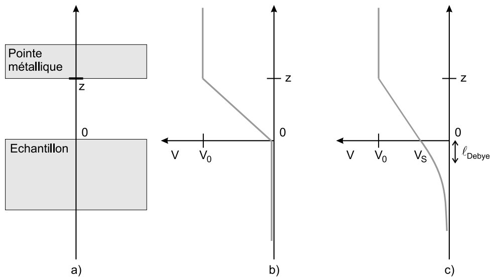
FIG. 3.2: Influence de l'écrantage sur la chute de potentiel. a) : Géométrie pointe-surface modélisée par deux plaques séparées d'une distance z . b) : Cas de deux métaux. La chute de potentiel s'effectue uniquement dans l'intervalle de diélectrique. c) : Cas d'une pointe en métal et d'un échantillon semiconducteur non-dégénéré. La chute de potentiel s'effectue dans l'intervalle de diélectrique, mais aussi dans le semiconducteur.
