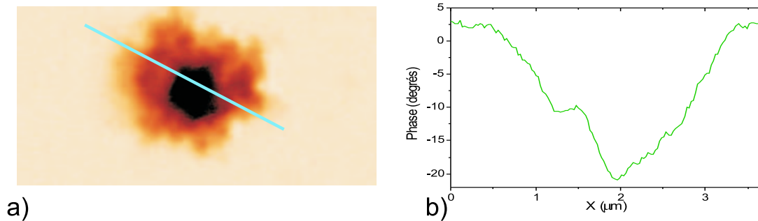
FIG. 4.13: Comportement au chargement de l'échantillon E2. Les conditions de chargement sont -10 V/10 s. a) : Image de signal EFM. La tache de charge est rugueuse. b) : Profil de l'image EFM montrant l'inhomogénéité des régions chargées.
