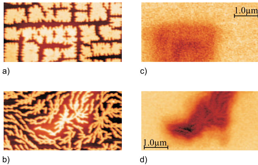
FIG. 4.6: Propagation de la charge dans une nanostructure ramifiée déposée sur oxyde mince. Les conditions d'injection sont -10\text{ V}/10\text{ s} . Images du haut : 1 er type de structure ramifiée. Images du bas : 2 e type de structure ramifiée. a) et c) : Images de topographie : la nanostructure chargée apparaît avec une hauteur apparente supérieure aux autres structures. b) et d) : Images du signal EFM, enregistrées à 100 nm de hauteur. Echelles respectives de 4 et 10 degrés. En d), la pointe est polarisée à +1\text{ V} . La charge s'est propagée à toute la nanostructure et de manière homogène. La nanostructure peut être considérée comme iso-potentielle.
