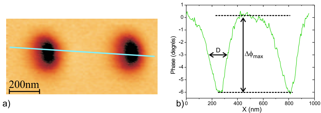
FIG. 4.17: Définitions des paramètres significatifs du nuage de charge sur l'échantillon E3. a) : Image EFM de deux chargements à -10 \text{ V}/3 \text{ s} . b) : Profil de chargement, et définitions de la variation de phase maximale \Delta\phi_{max} ainsi que de la largeur à mi-hauteur D .
