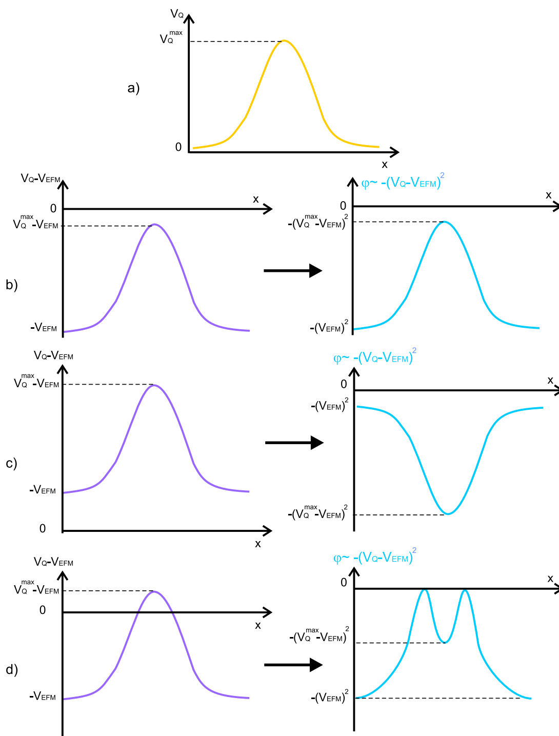
FIG. 1.15: Détermination du signe des charges injectées par la tension V_{EFM} appliquée sur la sonde. Exemple d'application à des charges positives. a) : Distribution surfacique du potentiel V_Q créé par des charges positives en excès. La phase étant proportionnelle à -(V_Q - V_{EFM})^2 , il en résulte que si V_{EFM} est également positif (cas b), il apparaît une bosse dans le signal de phase. Si V_{EFM} est négatif (cas c), il apparaît un creux. Dans le cas rare où V_Q et V_{EFM} sont de même signe, mais où |V_{EFM}| < |V_Q^{max}| (cas d), on obtient un profil plus complexe d'un creux avec une bosse au milieu.
