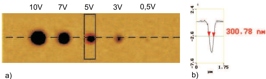
FIG. 2.1: Expériences d'injection de charges dans une fine couche de 7 nm de \text{SiO}_2 sur substrat de Si. Seule l'image de phase de 7 \times 1,75 \mu\text{m}^2 est représentée. a) : Injections successives de gauche à droite : 10 V, 7 V, 5 V, 3 V et 0,5 V, toutes de 5 secondes. Pour la détection, afin de discerner la tache à 0,5 V, une tension V_{EFM} de -4 V est appliquée. b) : Mesure de la valeur à mi-hauteur de la phase sur un profil de la tache à 5 V. Elle vaut environ 3^\circ .
