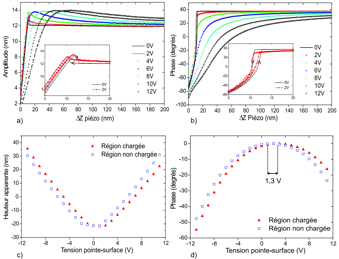
FIG. 2.14: Courbes d'approche-retrait expérimentales en mode non-contact avec couplage électrostatique. La position de la surface n'étant pas connue, seul le déplacement relatif du piézo vertical est donné. Les paramètres expérimentaux sont : f_0 = 136,708 kHz, u = 0,9988 , A_{libre} = 12 nm (amplitude loin de la surface à la fréquence d'excitation f = 0,9988f_0 ), Q = 150 . a) : Amplitude et b) : phase d'oscillation en fonction de la tension appliquée à la pointe. Les inserts sont des agrandissements de la zone d'hystérésis pour les courbes à 0 et 2 V. Le sens de déplacement de la pointe est indiqué. c) : Hauteur apparente et d) : décalage en phase en fonction de la tension appliquée sur la pointe, sur une région chargée et une région non chargée.
