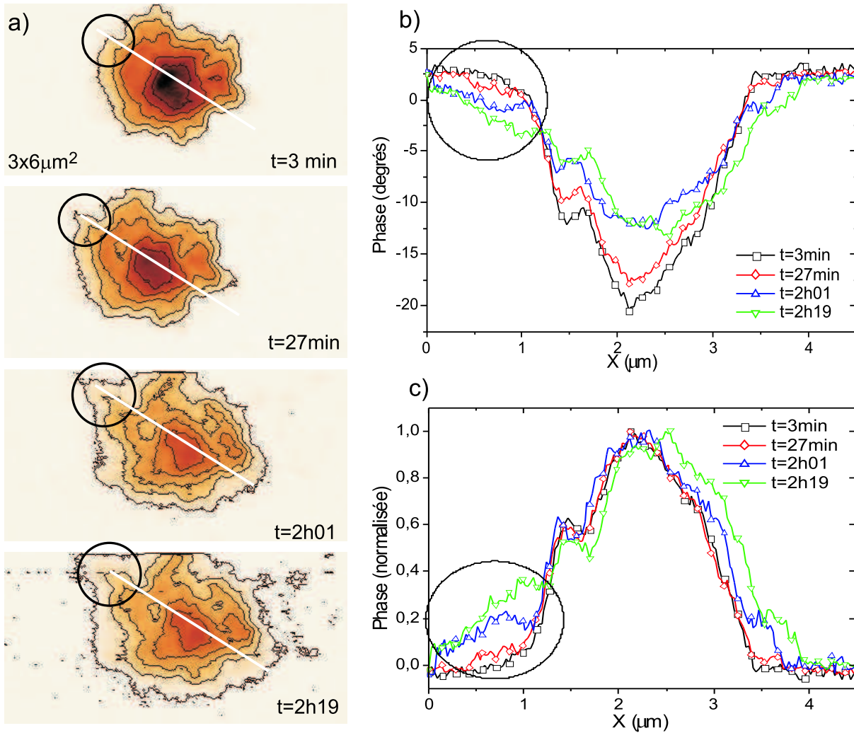
FIG. 4.23: Evolution temporelle du nuage de charges sur l'échantillon E2. Les conditions d'injection sont -10 \text{ V}/10 \text{ s} . a) : Images EFM ( 3 \times 6 \mu\text{m}^2 ) enregistrées sur 2h20 montrant l'étalement progressif et inhomogène du nuage de charges. Les contours du nuage sont mis en évidence. b) : Evolution temporelle d'une coupe du nuage. c) : Mêmes profils, normés. La région encerclée souligne le remplissage par des charges de certaines zones de l'échantillon au détriment d'autres.
