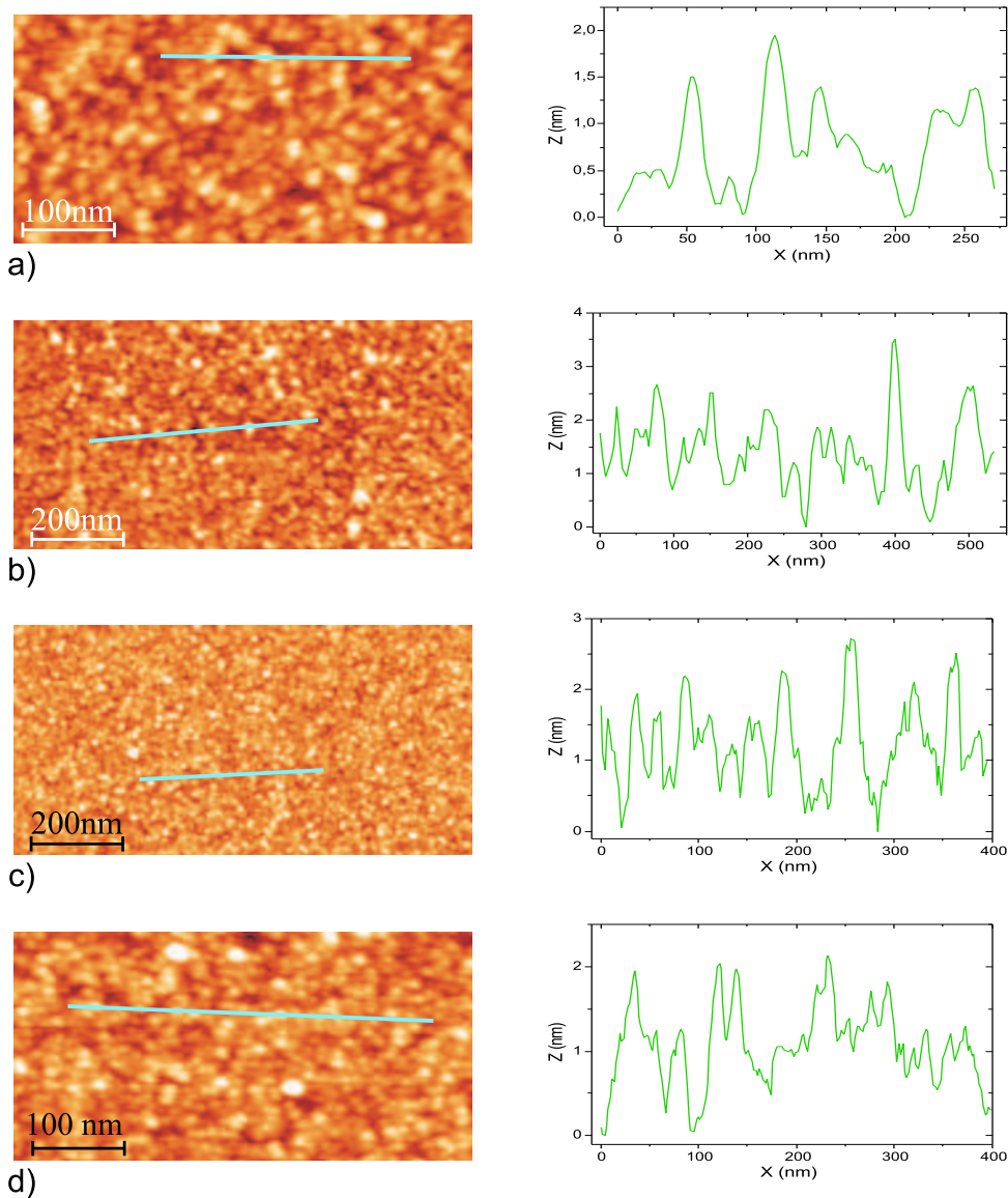
FIG. 3.15: Images de topographie AFM des nanocristaux de Si enfouis dans du \text{SiO}_2 (à gauche), et profils de hauteur (à droite). a) : Echantillon E1, rugosité RMS : 3,7 \text{ \AA} . b) : Echantillon E2, rugosité 6,5 \text{ \AA} . c) : Echantillon E3, rugosité 6,0 \text{ \AA} . d) : Echantillon E4, rugosité 6,1 \text{ \AA} . Toutes les rugosités sont comparables et faibles, en particulier même lorsqu'il n'y a pas de nanocristaux (Echantillon E4, non recuit). Ceci indique que les nanocristaux sont bien enfouis dans le \text{SiO}_2 , et ne contribuent donc pas à la rugosité de la surface.
