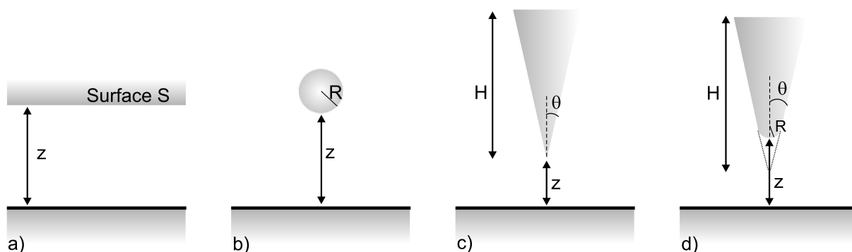
FIG. 1.17: Géométries pointe-surface pour la modélisation des forces capacitatives. a) : Géométrie plan-plan de surface S . On néglige les effets de bords dûs à la surface infinie en regard de la pointe. b) : Géométrie sphère-plan pour une sphère de rayon R . c) : Géométrie cône-plan pour un cône de hauteur H et de demi-angle d'ouverture \theta . d) : Géométrie cône tronqué-plan. Le cône tronqué est constitué d'un cône de hauteur H et de demi-angle d'ouverture \theta tronqué à son apex par une sphère de rayon R .
