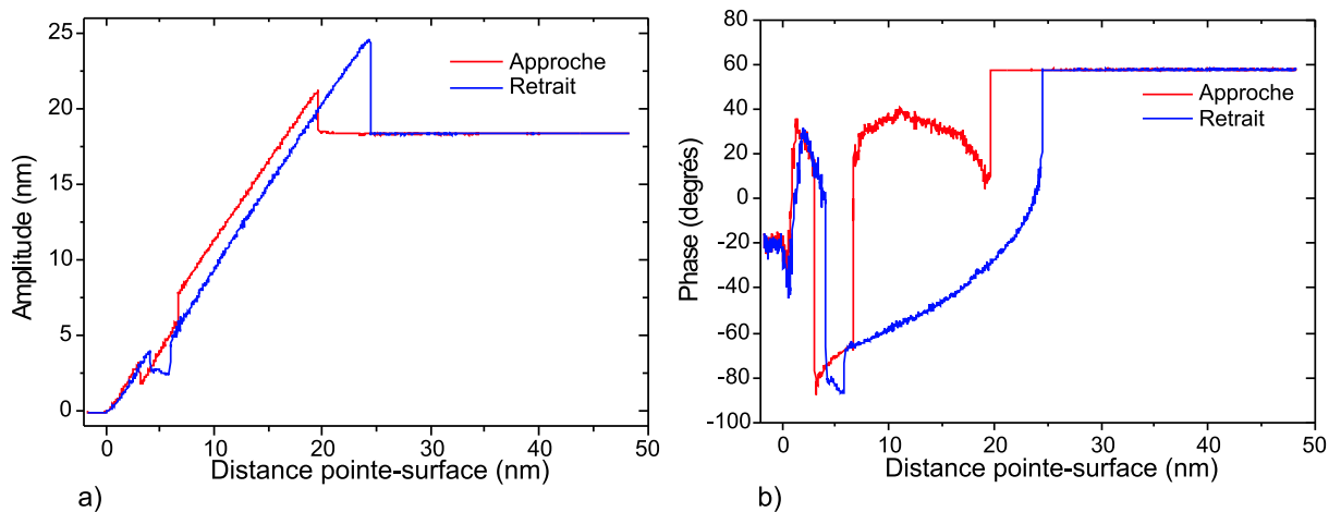
FIG. 2.12: Mise en évidence expérimentale de la pollution de la pointe ou de la surface. a) Amplitude. b) : Phase. Le système passe continuellement entre les modes non-contact et contact intermittent, à l'approche comme au retrait.
