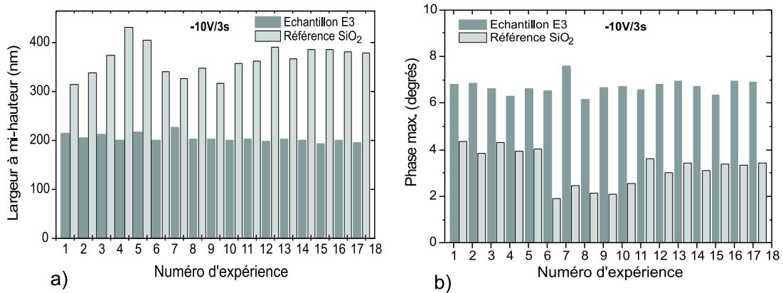
FIG. 4.18: Reproductibilité de l'injection de charges sur l'échantillon E3 et sur l'échantillon référence. La même pointe a été employée pour les deux échantillons, avec des conditions de chargement de -10 \text{ V}/3 \text{ s} . a) : Largeur à mi-hauteur du nuage de charges. b) : Variation maximale de phase, mesurée au centre du nuage de charges. La reproductibilité est excellente sur E3, correcte sur l'échantillon de référence.
