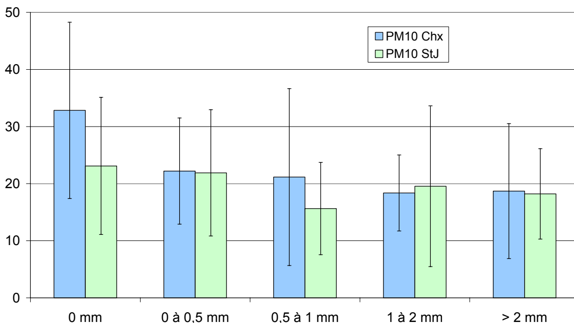
figure IV-23 : Evolution de la concentration des PM_{10} en fonction des précipitations.
