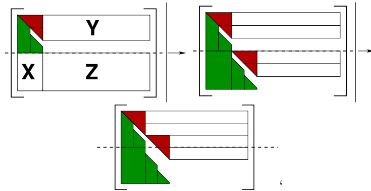
FIG. 3.4 – Principe de la factorisation LQUP
