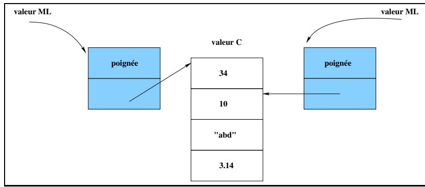
FIG. 3.1 – Représentations de la même donnée C en ML
