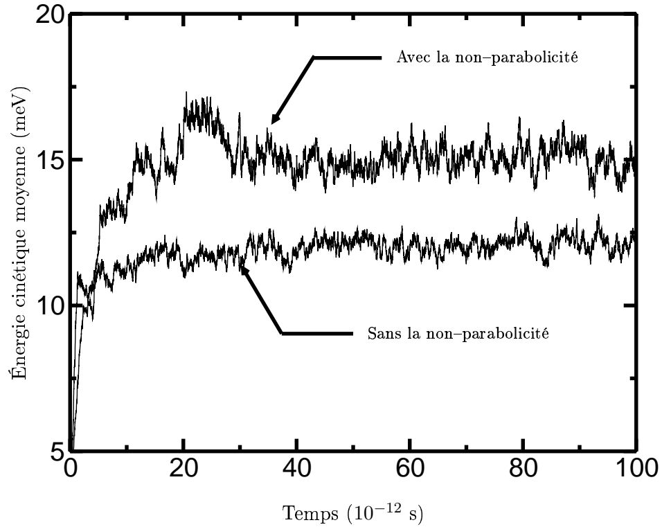
FIG. F.5 – Évolution temporelle de la moyenne d'ensemble de l'énergie cinétique du LCQ de la figure 7.1 en traitant ou non la non-parabolicité dans l'interaction électron-électron.
