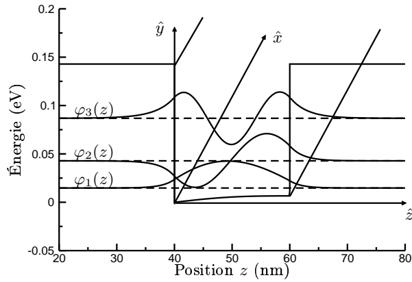
FIG. 1.8 – États quantifiés de la bande de conduction d'une double hétérostructure en GaAs/ \text{Al}_{0,18}\text{Ga}_{0,82}\text{As} . Les traits pointillés symbolisent les énergies propres \{E_\nu, \nu = 1, 2, 3\} correspondants aux fonctions d'onde \varphi_\nu(z) . L'unité des fonctions d'onde \varphi_\nu(z) , qui est le mètre ^{-1/2} , n'est généralement pas indiquée, car elles sont définies à une constante de normalisation près.
