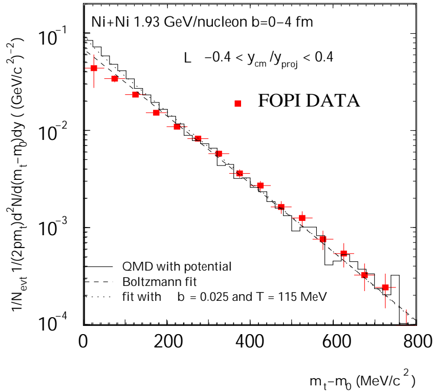
FIG. 6.5 – Spectres en masse transverse expérimentaux des \Lambda (carrés) pour des collisions centrales ( b < 4 fm) Ni+Ni à 1,93 AGeV et une rapidité comprise entre -0,4 < y_{\text{cm}}/y_{\text{proj}} < 0,4 . Les prédictions du modèle QMD [105] avec potentiel \Lambda -nucléon (lignes) sont ajustées par les distributions thermiques de type Boltzmann (tirets) et de type Siemens et Rasmussen (pointillés).
