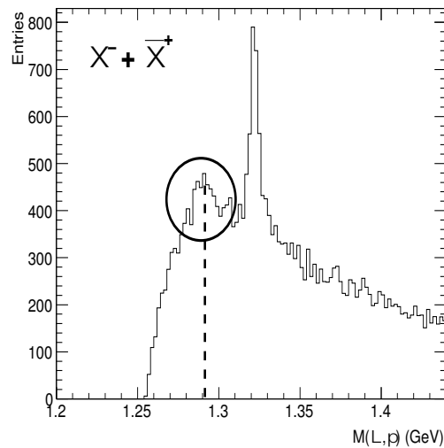
FIG. 5.7 – Spectre en masse invariante des \Xi^- + \Xi^+ mesuré par la collaboration NA49 pour des collisions \text{Pb}+\text{Pb} à 30 \text{A GeV} [171]. Nous avons entouré le “faux” pic centré sur la masse de 1,29 \text{GeV}/c^2 .
