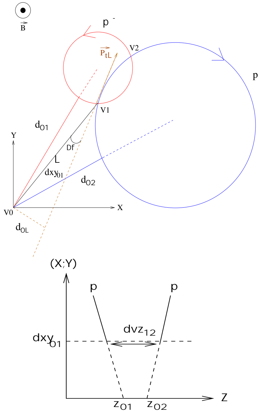
FIG. 4.9 – Schéma de reconstruction du \Lambda dans le plan transverse de la CDC (haut), et variables utilisées dans le plan longitudinal (bas).
