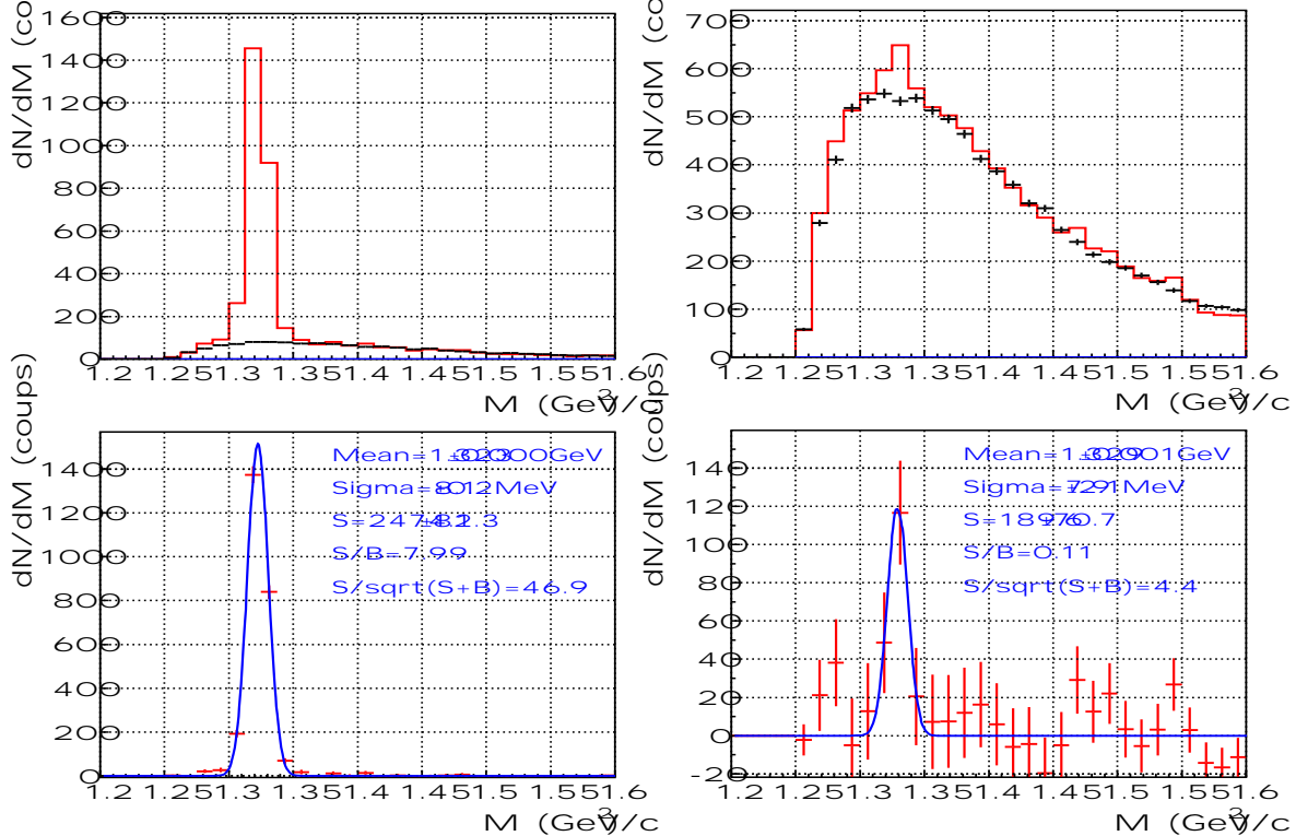
FIG. 5.8 – Spectres en masse invariante des \Xi^- obtenus avec la simulation (gauche) et avec les données expérimentales (droite) pour des collisions centrales Ni+Ni à 1,93 AGeV et avec le lot de coupures du tableau 5.2. La combinatoire est représentée par les histogrammes en traits pleins, le bruit de fond par les tirets. La distribution du signal pur après soustraction du bruit de fond (bas) est ajustée par une gaussienne.
