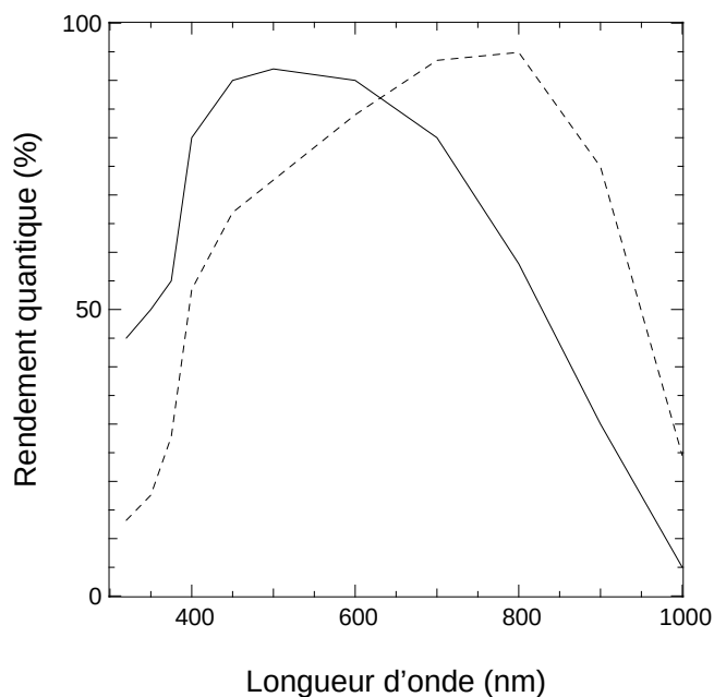
FIG. 6.8 – Rendement quantique dans le domaine visible en fonction de la longueur d'onde (en nm) du détecteur de l'ASO visible NAOS (trait plein) et du détecteur utilisé sur FORS-2 (en pointillés).
