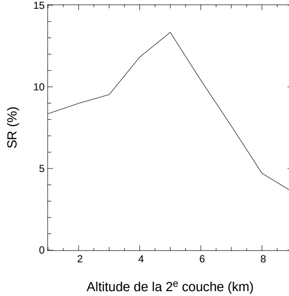
FIG. 5.9 – Evolution du rapport de Strehl en fonction de l'altitude de la deuxième couche. La matrice de reconstruction suppose une altitude h_2 = 5 kilomètres. Analyse et correction des polynômes de Zernike 2 à 120.
