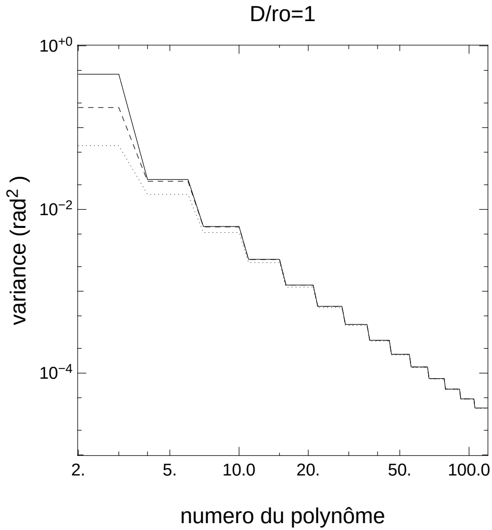
FIG. 2.5 – Variance théorique des 120 premiers coefficients de Zernike (échelle logarithmique) et pour des échelles externes \mathcal{L}_0 = \infty (trait plein), \mathcal{L}_0 = 100\text{m} (trait) et \mathcal{L}_0 = 24\text{m} (points, valeur médiane au Cerro-Paranal). La pupille considérée a un diamètre D = 8 mètres.
