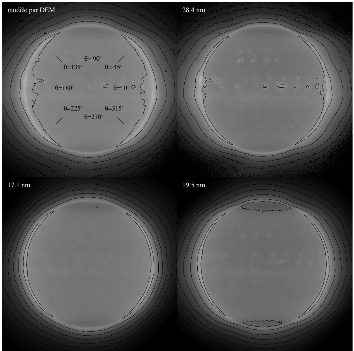
FIG. 4.3 – Comparaison des deux méthodes utilisées pour mesurer l'intensité de la raie de résonance de l' \text{He}^+ à partir des images enregistrées à 30.4 nm par EIT. En haut à gauche, le résultats de l'analyse par DEM. Les trois autres panneaux sont les images correspondantes à 17.1 nm, 19.5 nm et 28.4 nm. L'image à 28.4 nm est remarquablement semblable à la carte des contaminants obtenue par DEM. Les deux autres images à 17.1 nm et 19.5 nm sont nettement différentes, avec en particulier des gradients bien plus forts au-dessus du limbe. Ceci confirme que la réponse en température de la bande passante à 30.4 nm est proche de la celle de la bande passante à 28.4 nm pour les hautes températures, et justifie le choix de la bande passante à 28.4 nm comme modèle des contaminants.
