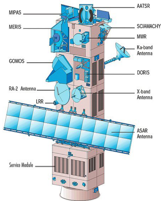
Figure III.25 : Satellite ENVIAT et ses différents instruments (source : http://envisat.esa.int/ ).
