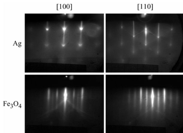
Fig.IV.7 : Clichés RHEED obtenus sur une couche de 7nm de Ag déposée à 200°C sur Fe 3 O 4 (001).
