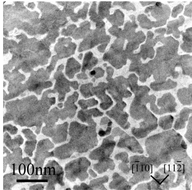
Fig.IV.36 : Cliché MET en vue plane de 7nm de Au déposé à 750°C sur \text{Fe}_3\text{O}_4(111) .
