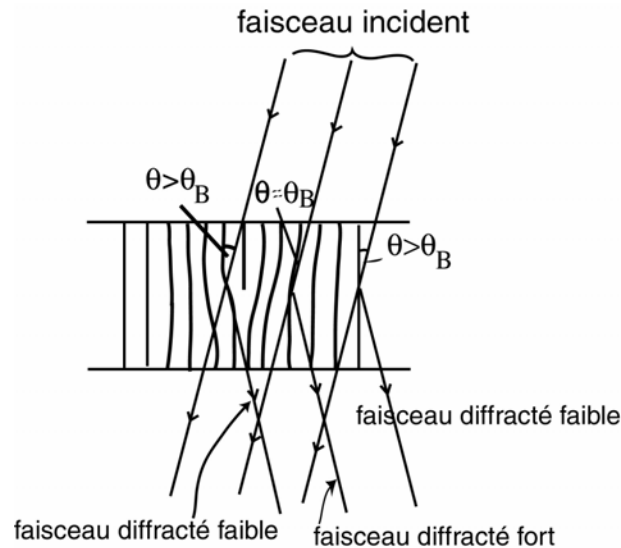
Fig.C.24 : Schéma de la diffraction et de la transmission des faisceaux électroniques au travers de l'objet.
