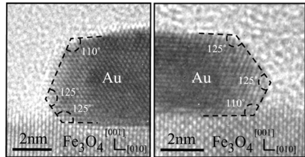
Fig.IV.24 : Clichés MEHR en section transverse de grains Au déposés à 400^\circ C sur Fe_3O_4(001) .
