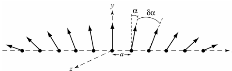
Fig.I.7 : Rotation des moments magnétiques le long de l'axe x.
