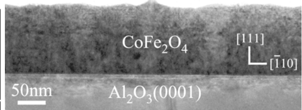
Fig.II.64 : Cliché MET en section transverse d'une couche de 120nm de CoFe_2O_4 déposée sans O_2 à 400°C sur Al_2O_3(0001) .
