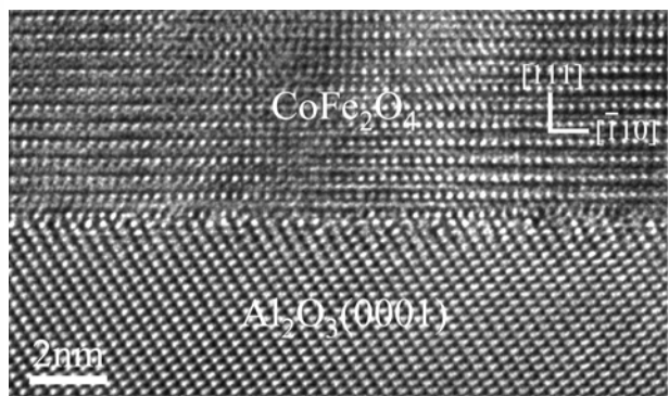
Fig.II.75 : Cliché MEHR en section transverse de l'interface entre une couche de \text{CoFe}_2\text{O}_4 déposée avec 10% d' \text{O}_2 à 600^\circ\text{C} et \text{Al}_2\text{O}_3(0001) .
