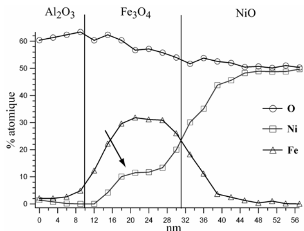
Fig.III.14 : Profil chimique en % atomique déduit des spectres EELS réalisés sur la bicouche NiO(66nm)/Fe 3 O 4 (20nm) épitaxiée sur Al 2 O 3 (0001). La flèche pointe la large diffusion du Ni dans la couche de Fe 3 O 4 .
