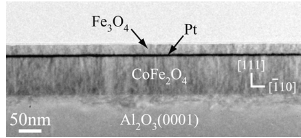
Fig. V.16 : Cliché MET en section transverse de la tricouche \text{Fe}_3\text{O}_4(40\text{nm})/\text{Pt}(5\text{nm})/\text{CoFe}_2\text{O}_4(120\text{nm}) épitaxiée sur \text{Al}_2\text{O}_3(0001) .
