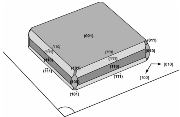
Fig.IV.45 : Schéma représentant la structure adoptée par les grains de Pt [001] déposés à 400°C et 750°C sur \text{Fe}_3\text{O}_4(001) .
