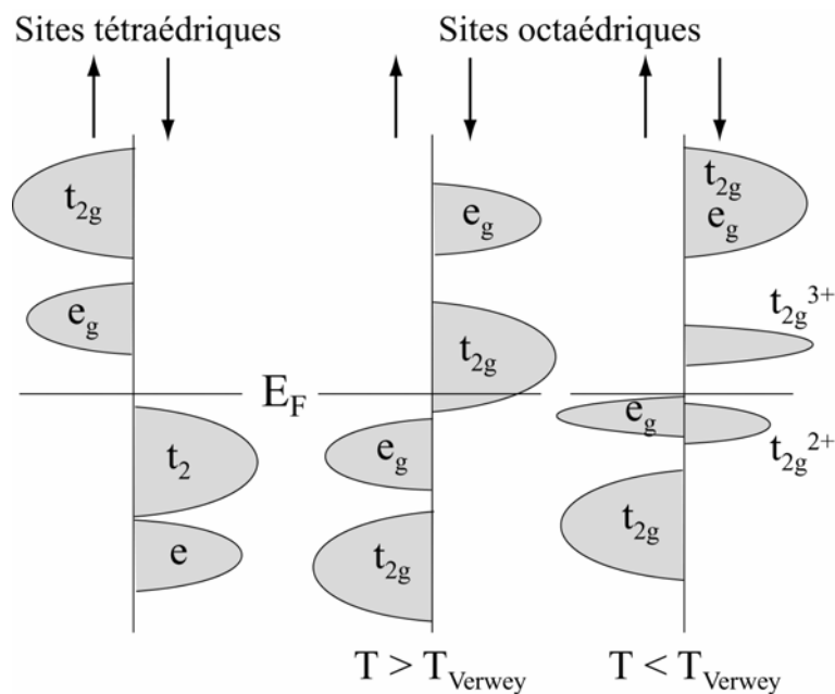
Fig.II.19 : Densité d'états de \text{Fe}_3\text{O}_4 . Pour les cations en sites octaédriques sont donnés les diagrammes de bandes à T < T_V et à T > T_V .
