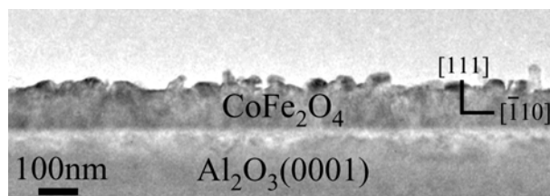
Fig.II.65 : Cliché MET en section transverse d'une couche de 120nm de \text{CoFe}_2\text{O}_4 déposée sans \text{O}_2 à 600°C sur \text{Al}_2\text{O}_3(0001) .
