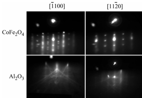
Fig.II.63 : Clichés RHEED d'une couche de 120nm de \text{CoFe}_2\text{O}_4 déposée sans \text{O}_2 à 600°C sur \text{Al}_2\text{O}_3(0001) .
