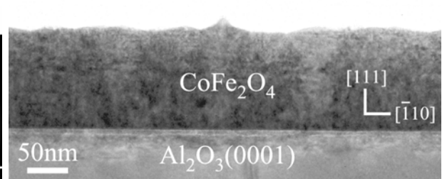
Fig.II.64 : Cliché MET en section transverse d'une couche de 120nm de \text{CoFe}_2\text{O}_4 déposée sans \text{O}_2 à 400°C sur \text{Al}_2\text{O}_3(0001) .
