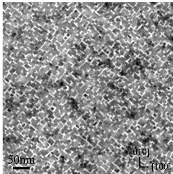
Fig.IV.46 : Cliché MET en vue plane de 5nm de Pt déposé à 750°C sur \text{Fe}_3\text{O}_4(001) .
