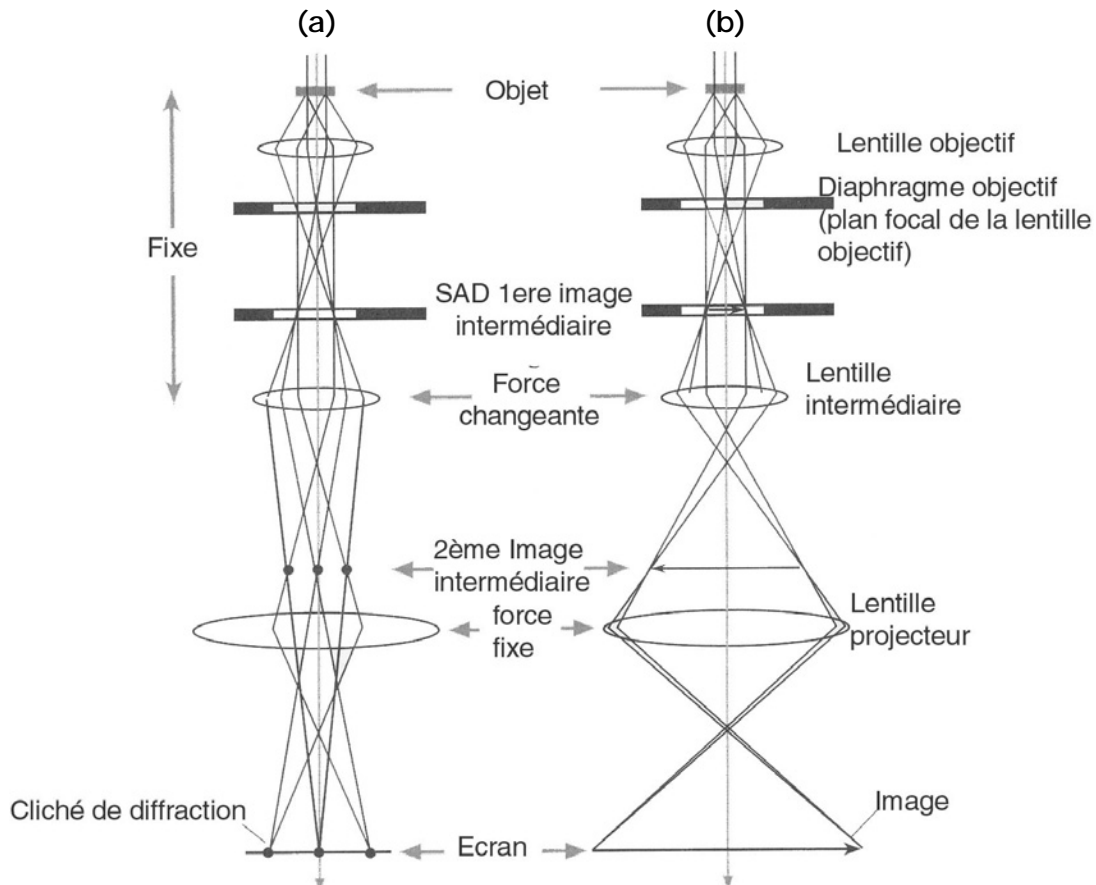
Fig.C.13 : Schémas optiques du mode diffraction (a) et du mode image (b) selon l'excitation de la première lentille intermédiaire.
