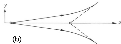
Fig.C.21: Action des quadripôles sur la trajectoire des électrons en 3D (a) et dans chaque plan de symétrie (b).
