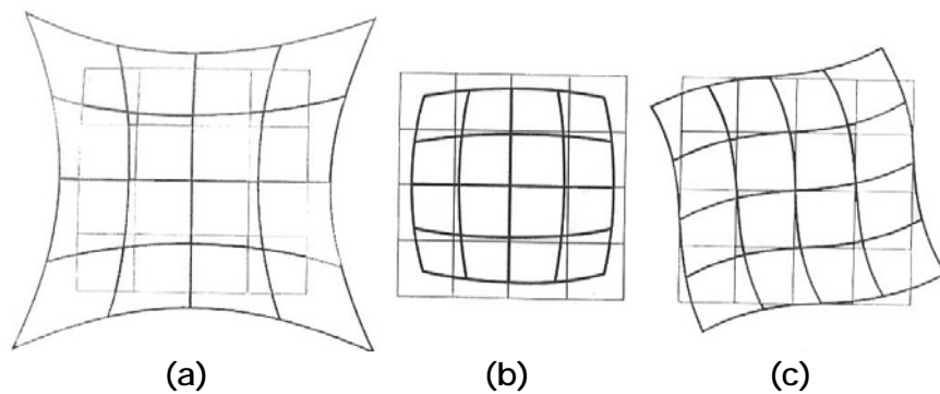
Fig.C.17 : Schémas représentant les différentes distorsions de l'image : en croissant (a), en barillet (b) et anisotrope (c).
