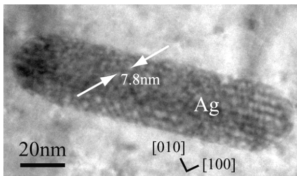
Fig.IV.16 : Cliché MET en vue plane d'un « bâtonnet » de Ag déposé à 750°C sur Fe_3O_4(001) .
