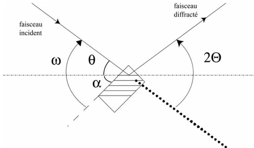
Fig.B.5 : Schéma du réglage en asymétrie.
