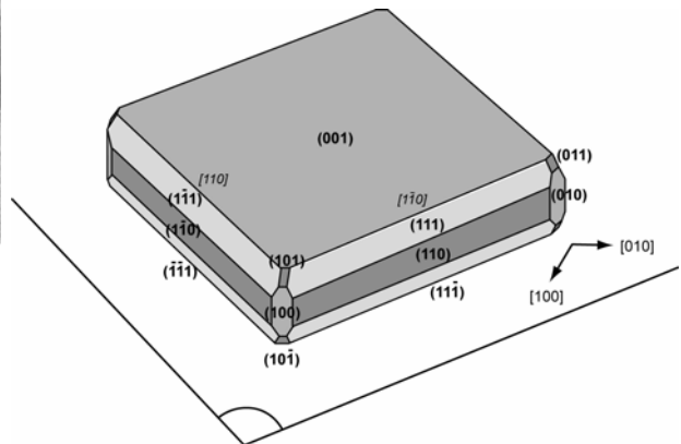
Fig.IV.45 : Schéma représentant la structure adoptée par les grains de Pt [001] déposés à 400°C et 750°C sur Fe_3O_4(001) .
