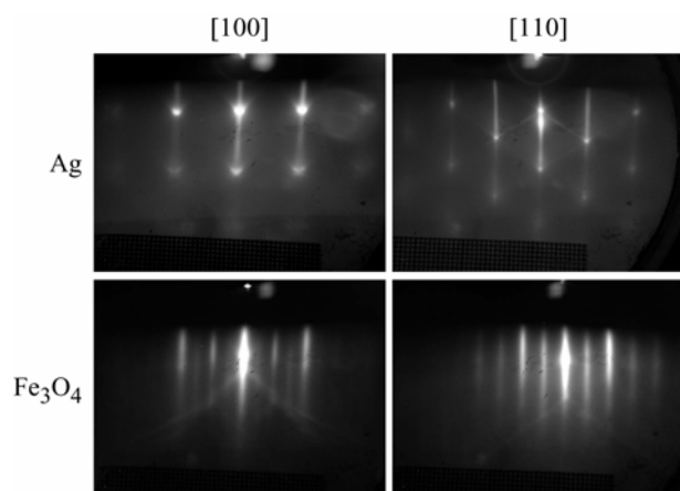
Fig.IV.7 : Clichés RHEED obtenus sur une couche de 7nm de Ag déposée à 200°C sur \text{Fe}_3\text{O}_4(001) .
