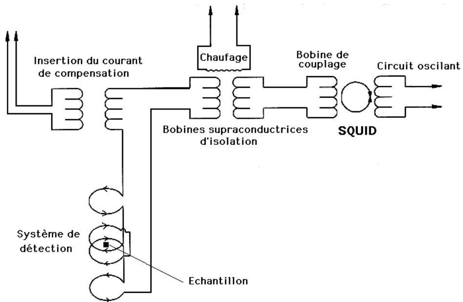
Fig.E.1 : Schéma de détection du magnétomètre utilisé : le flux détecté est transmis au SQUID via deux bobines supraconductrices permettant d'isoler le SQUID des fortes variations de flux engendrées par la variation du champ magnétique appliqué sur l'échantillon.
