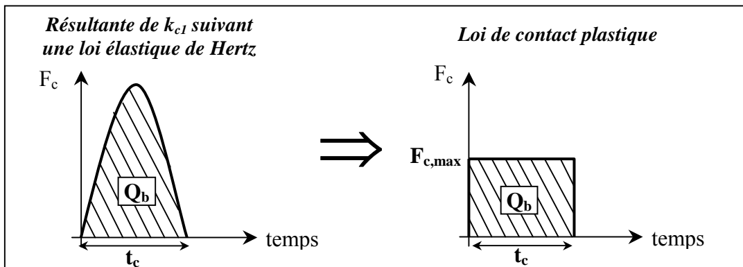
figure V.30 : détermination de l'effort de contact pour le modèle simplifié « contact »
