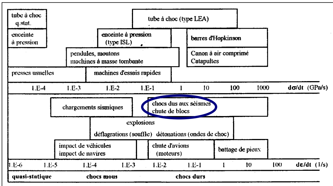
figure II.7 : vitesses de déformation en fonction du type de choc [TOU, 95]
