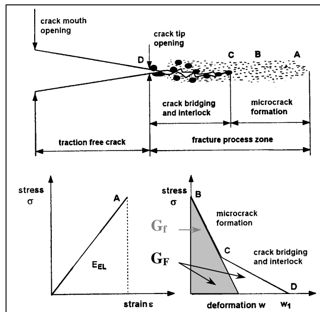
figure IV.18 : structure générale d'une FPZ dans le béton [MOM, 03]
