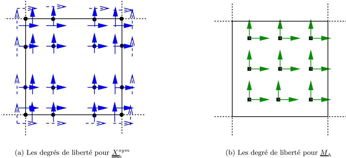
FIG. 3.2.5 – Degrés de liberté pour l'élément Q_3 - Q_2
