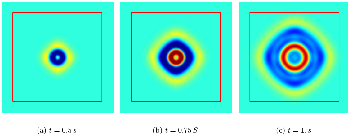
FIG. 8.3.1 – La pression dans un milieu anisotrope
