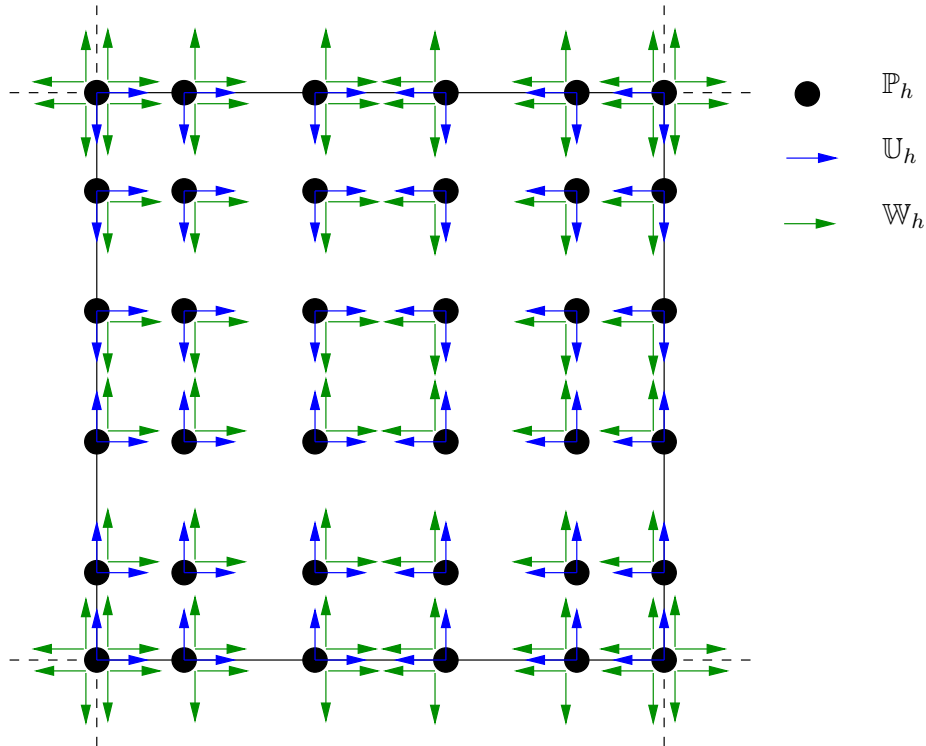
FIG. 7.3.3 – Les degrés de libertés associées à P_h , U_h et W_h pour r = 5
