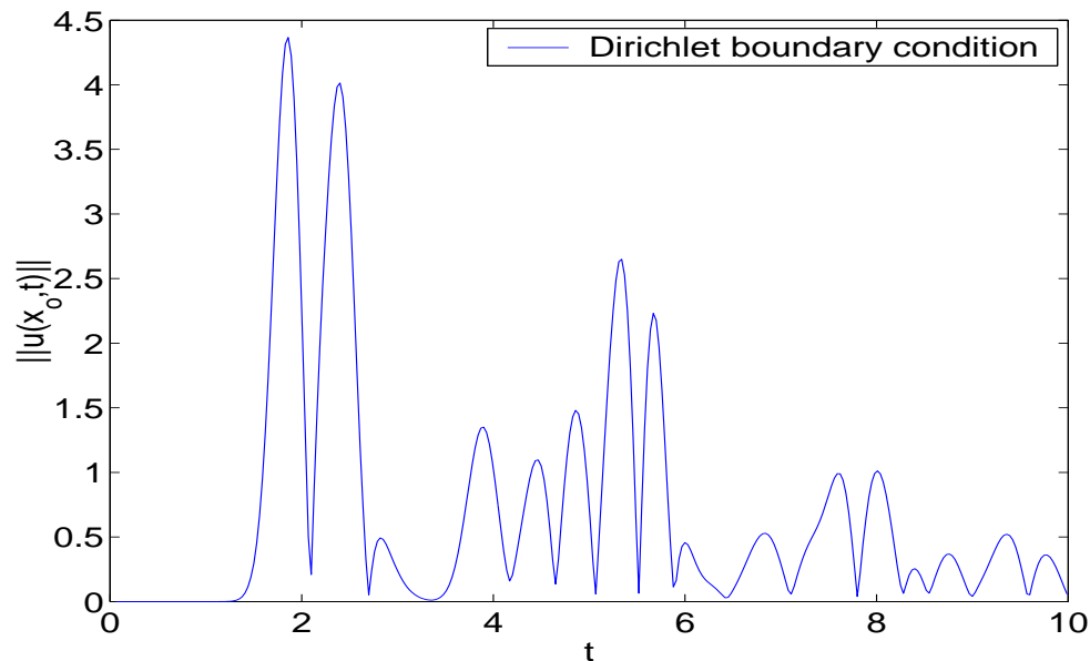
FIG. 4.2.10 – Sismogramme dans un milieu borné sans PML
