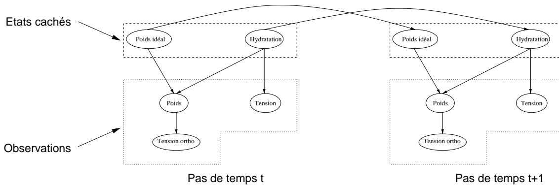
FIG. 4.9 – Modèle d'évolution du système Diatelic™v3. Les nœuds représentant les états cachés sont reliés d'un pas de temps à l'autre pour modéliser la relation markovienne d'ordre un qui existe entre eux.
