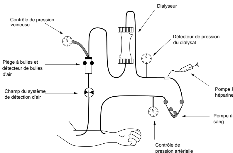
FIG. 1.1 – Circuit d'hémodialyse
