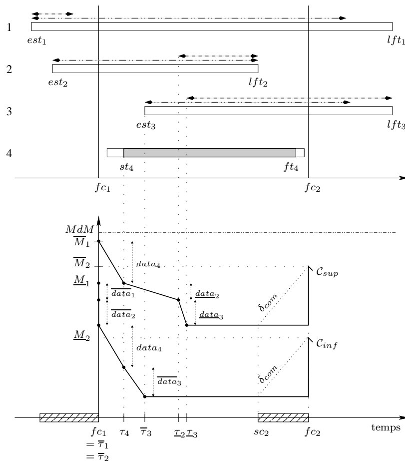
FIG. 6.6 – Exemple de construction des courbes \mathcal{C}_{inf} et \mathcal{C}_{sup} sur un intervalle [fc_1, fc_2] pour un ensemble de quatre expériences élémentaires
