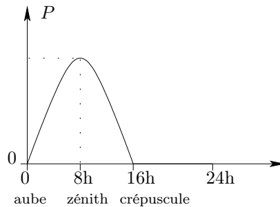
FIG. 6.11 – Profil de la puissance fournie pour l'exemple
