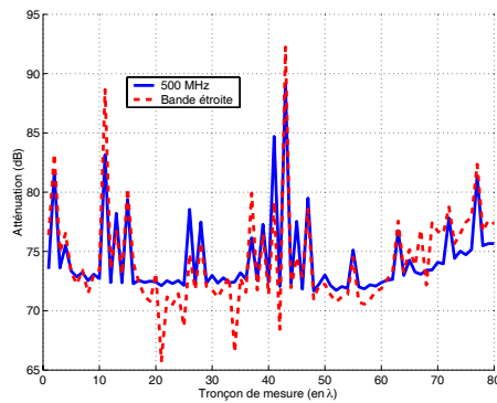
(e) Exemple 3 : A(d) et A_{BE}(d) - Pas : \lambda
