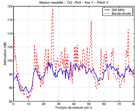
(a) Exemple 1 : A(d) et A_{BE}(d) - Pas : \lambda/2
