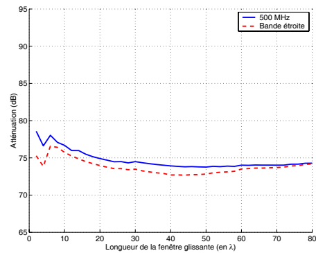
(f) Exemple 3 : Am_{n,\lambda} et Am_{BE n,\lambda} pour n = \{2, 4, \dots, 80\}
