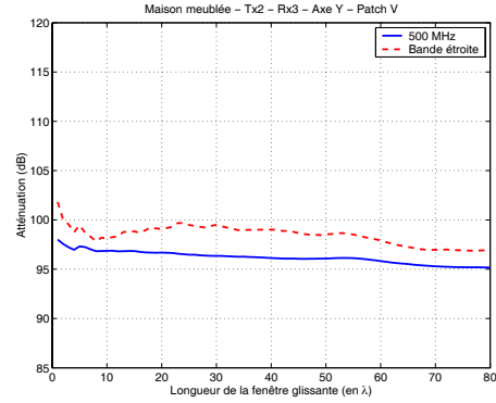
(b) Exemple 1 : Am_{n,\lambda/2} et Am_{BE n,\lambda/2} pour n = \{2, 4, \dots, 160\}
