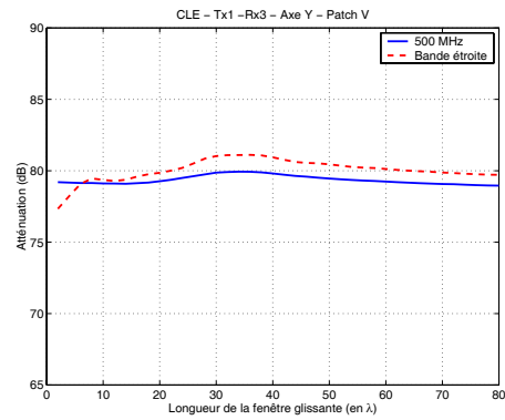
(d) Exemple 2 : Am_{n,\lambda} et Am_{BE n,\lambda} pour n = \{2, 4, \dots, 80\}
