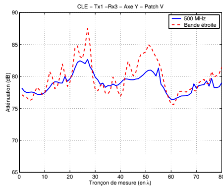
(c) Exemple 2 : A(d) et A_{BE}(d) - Pas : \lambda
