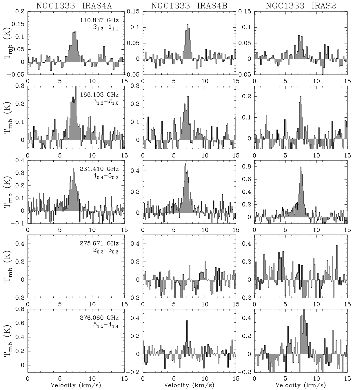
FIG. 4.3 – Transitions de \text{D}_2\text{CO} observées sur IRAS4A, IRAS4B et IRAS2.
