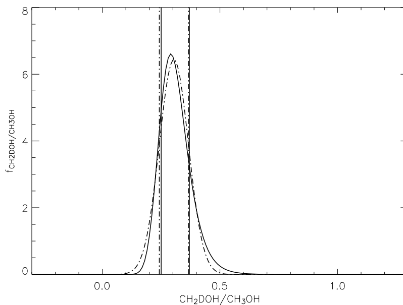
FIG. A.4 – Simulation de la fonction de répartition exacte du rapport isotopique CH 2 DOH/CH 3 OH (trait plein) pour le cas présenté en Fig. A.3. Approximation gaussienne (trait pointillé). Les barres verticales délimitent les intervalles de confiance à 68% pour chacune des distributions.
