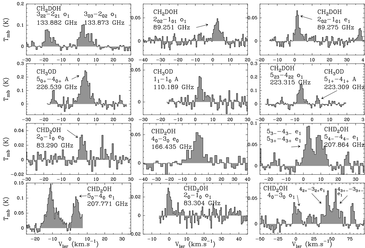
FIG. 3.3 – Exemples de transitions de CH 2 DOH, CH 3 OD et CHD 2 OH. Les intensités sont en température de lobe principal.
