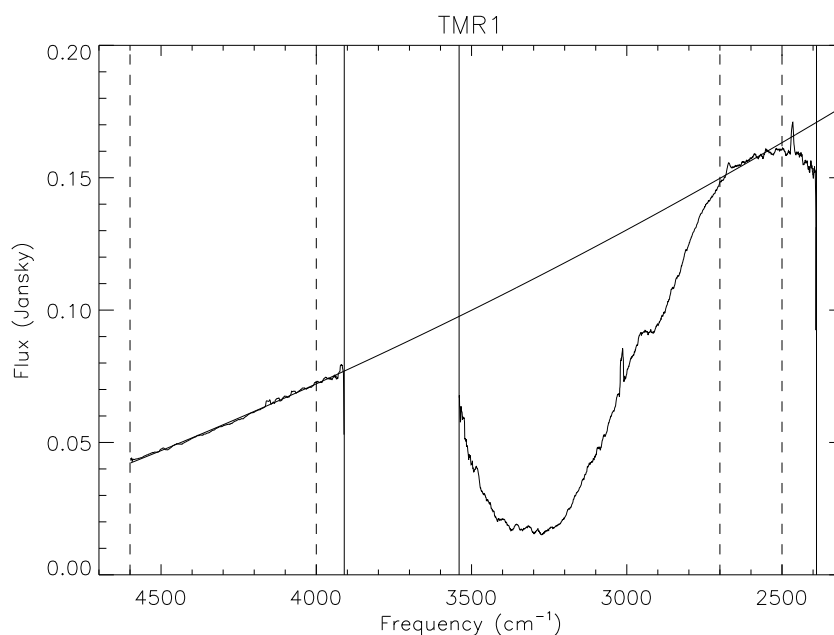
FIG. 5.10 – Exemple de la détermination du continuum pour l'étude de l'absorption à 3,0 \mu\text{m} . Les traits pointillés verticaux délimitent les intervalles de fréquence utilisés pour ajuster le continuum.
