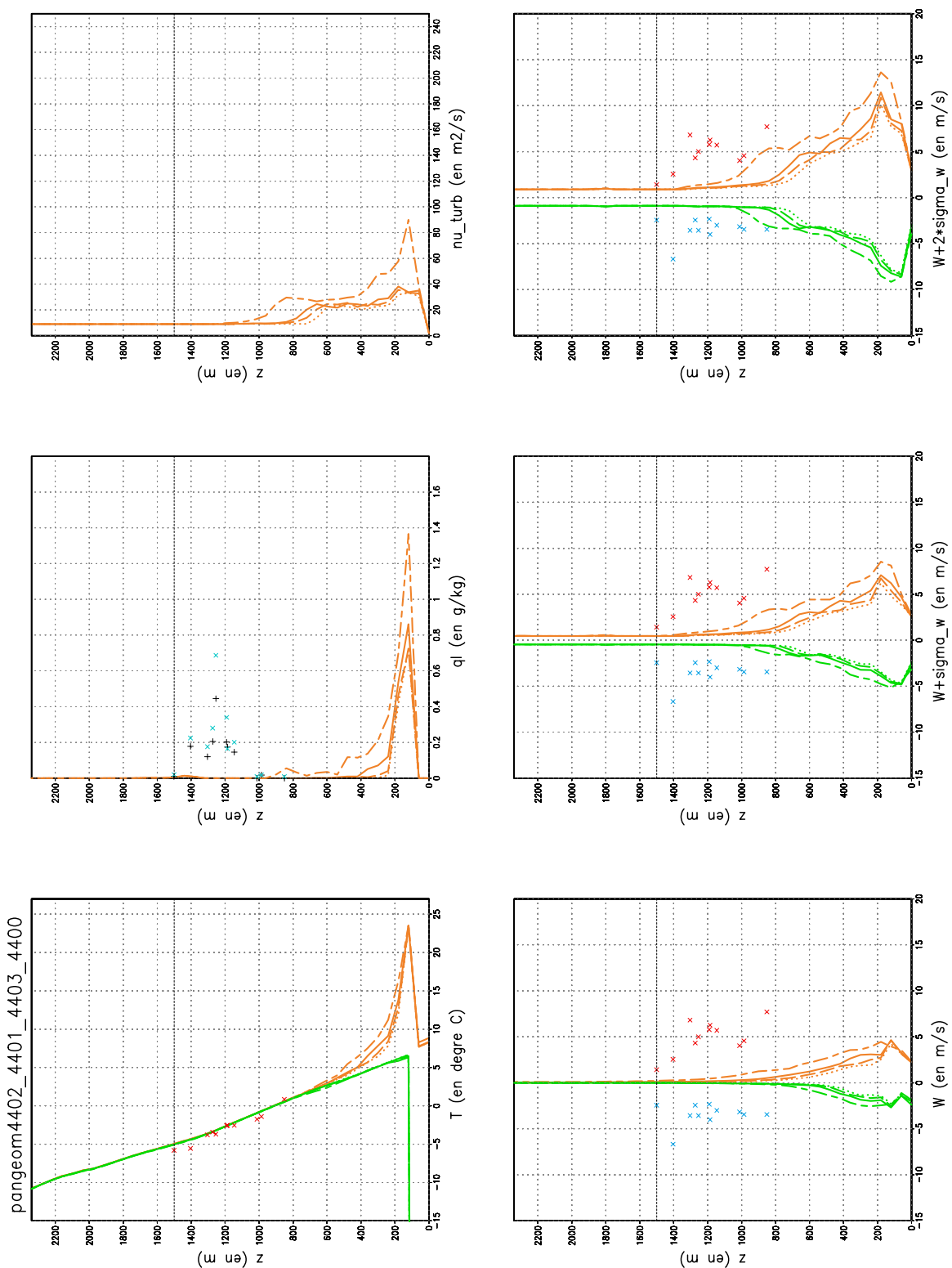
FIG. B.22 – Le 07 mars 1980 10h52. "Tableau de bord" sur la sensibilité à la turbulence au rejet.
