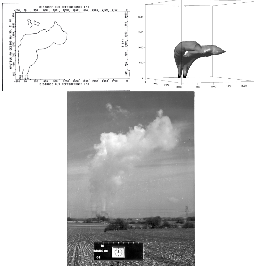
FIG. B.13 – Le 10 mars 1980, photo, croquis et simulation réalisé à 12h15.
