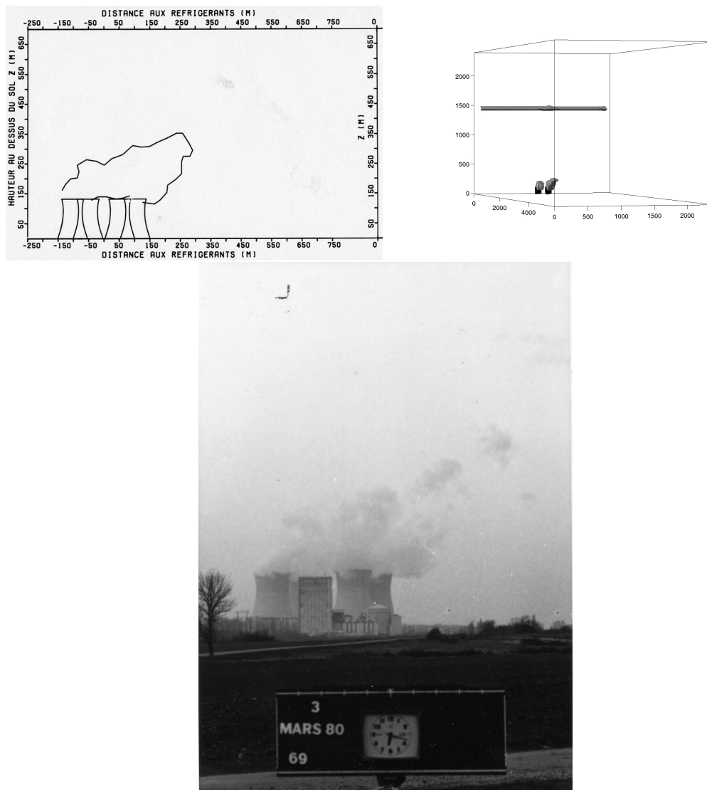
FIG. B.9 – Le 3 mars 1980, photo et croquis à 18h15 et simulation réalisé à 15h50.
