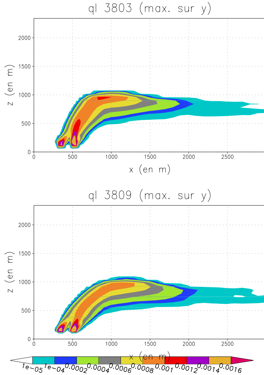
FIG. B.38 – Le 4 mars 1980 11h. Figure du haut : cas avec le maillage standard \Delta Z constant ( \Delta Z = 60m ). Figure du bas : cas avec un maillage raffiné à la hauteur du rejet \Delta Z = 15m de part et d'autre de Z = 128m et \Delta Z augmente progressivement vers le sol et le sommet de domaine ( \Delta Z_{max} = 100m ).
