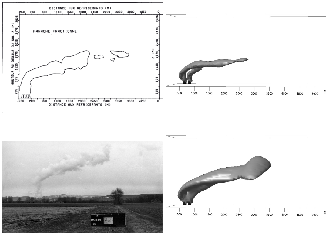
FIG. B.16 – Le 13 mars 1980, photo et croquis à 17h20 et simulation réalisé à 16h30. La simulation est réalisée avec des profils de température corrigés et sous des conditions de simulation standard en haut ( \nu_t = 27m^2/s au rejet en haut), en bas ces conditions sont modifiées au niveau du rejet où l'on prend \nu_t = 90m^2/s .
