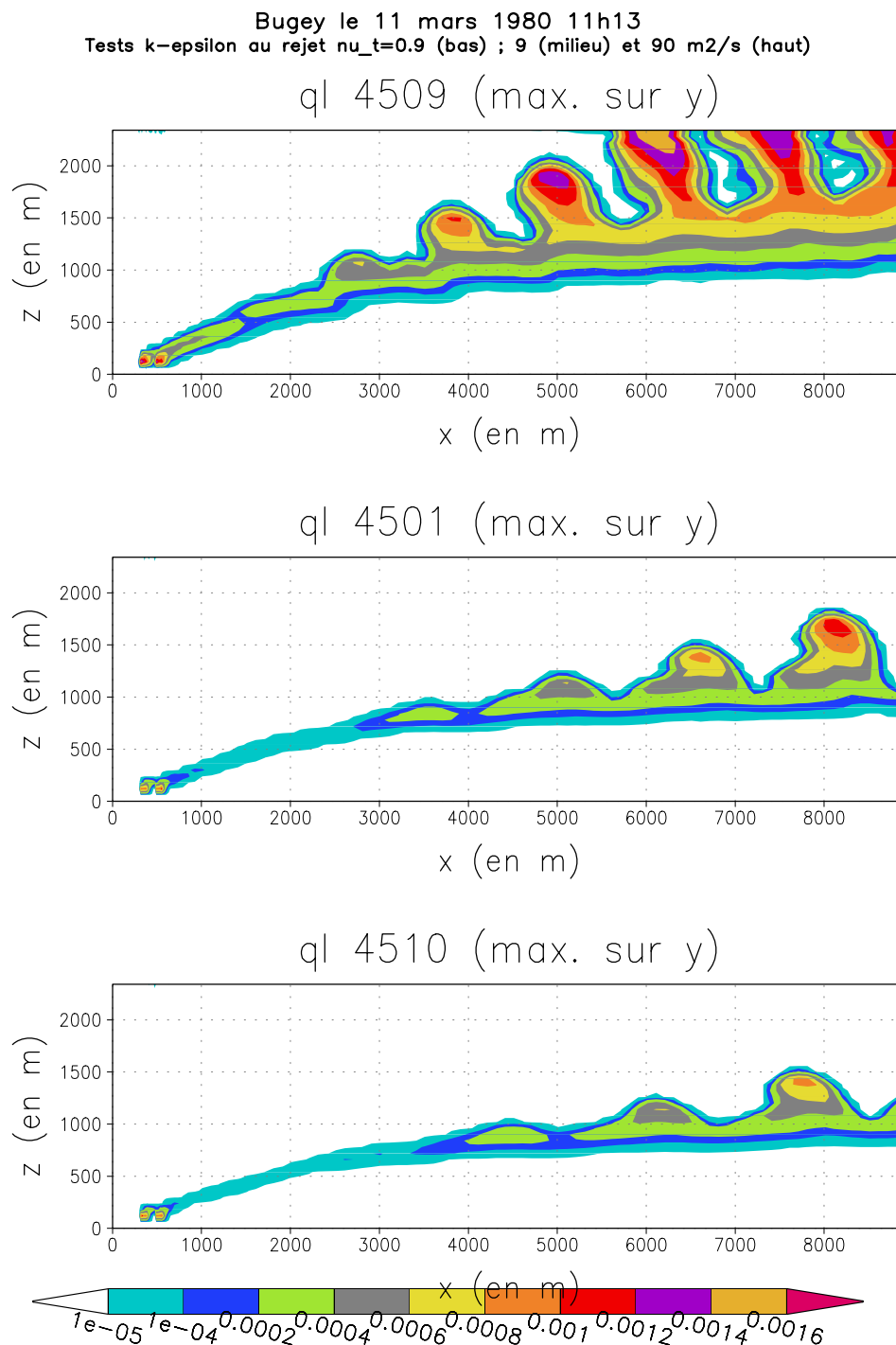
FIG. 8.1 – Le 11 mars 1980 11h13, test de différentes valeurs de turbulences en sortie des tours. Figure du haut : cas \nu_t = 90m^2.s^{-1} ( k = 10m^2.s^{-2} et \varepsilon = 0.1m^2.s^{-3} ). Figure du milieu : cas \nu_t = 9m^2.s^{-1} ( k = 1m^2.s^{-2} et \varepsilon = 0.01m^2.s^{-3} ). Figure du bas : cas \nu_t = 0.9m^2.s^{-1} ( k = 0.5m^2.s^{-2} et \varepsilon = 0.025m^2.s^{-3} ). On représente ici le maximum du contenu en eau liquide q_l selon l'axe horizontal Y .
