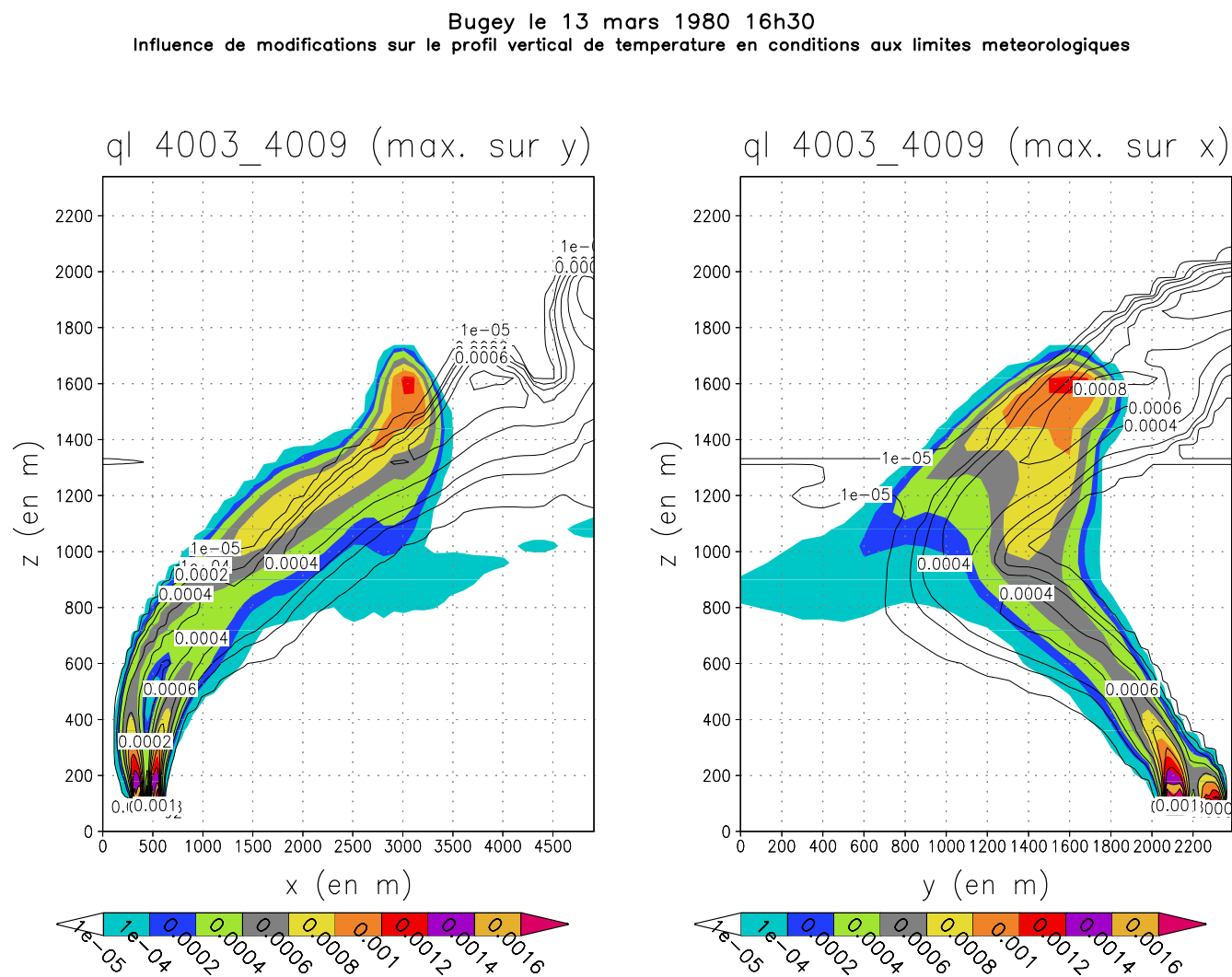
FIG. 8.8 – Le 13 mars 1980 16h30, test sur le profil vertical de température atmosphérique. Les surfaces colorées correspondent à la simulation avec un profil corrigé (température rehaussée à partir de radiosondages différents, des valeurs utilisées par Louis et al. (1984) et des mesures de température aéroportées). Les isolignes noires correspondent à la simulation avec un profil vertical de température en conditions aux limites donné par l'interpolation standard, cf. profils A.18.
