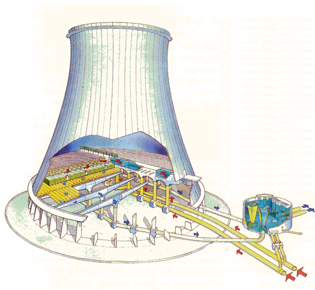
FIG. 5.2 – Vue éclatée d'un aéroréfrigérant
