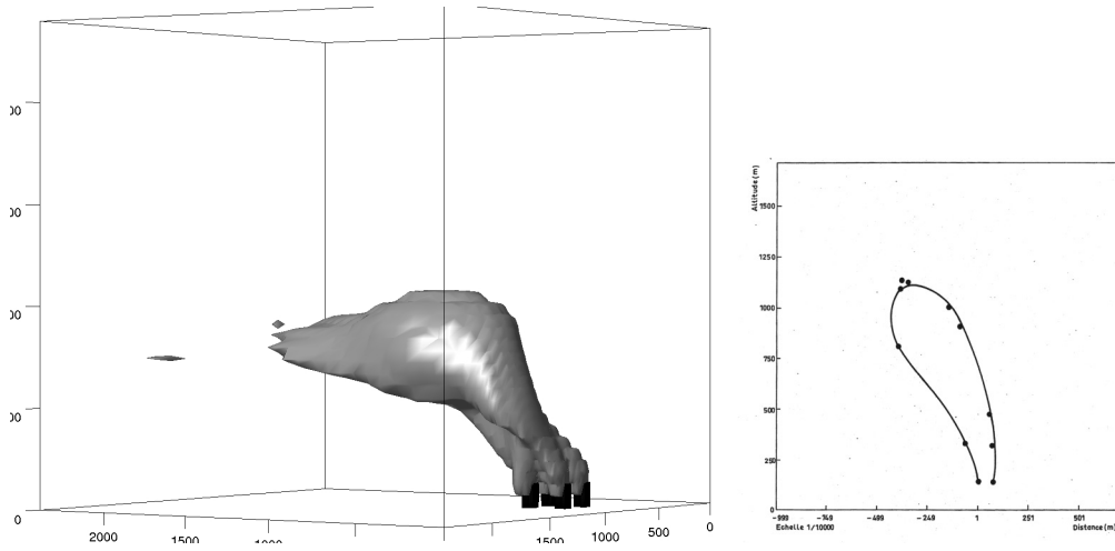
FIG. 7.13 – Le 4 mars 1980, photogramm trie   10h35, simulation r alis e   11h00. Vue de c t .
