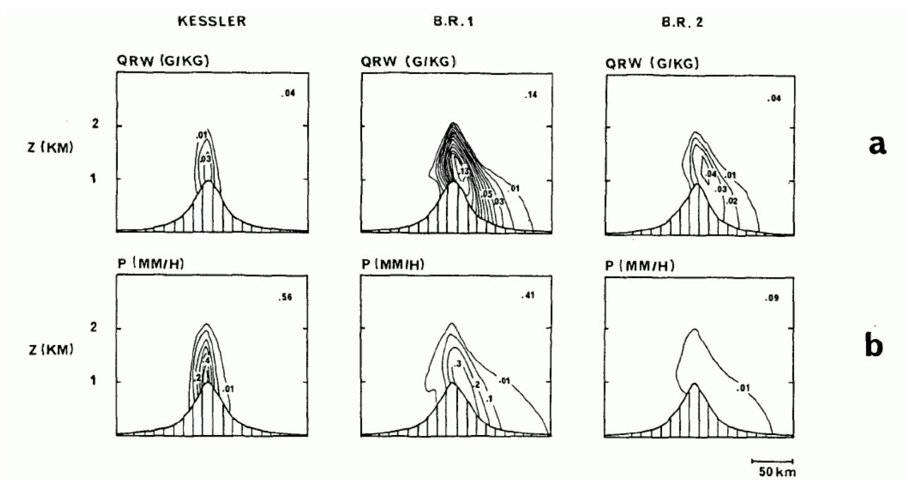
FIG. 12.14 – Idem que la figure 12.13 mais pour le run B. (Tiré de la Fig. 9 de RC)
