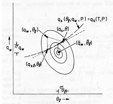
FIG. 4.4 – Diagramme schématique de la distribution des variables \theta_l et q_w à l'intérieur d'un maille. D'après Somméria et Deardorff (1977).
