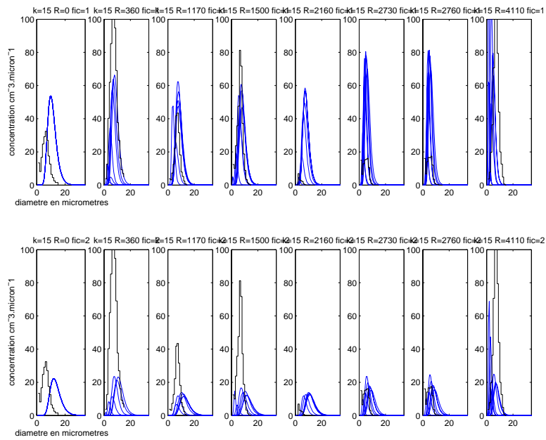
FIG. B.66 – Idem figure B.58. Palier n°10.
