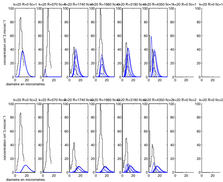
FIG. B.61 – Idem figure B.58. Palier n°8.
