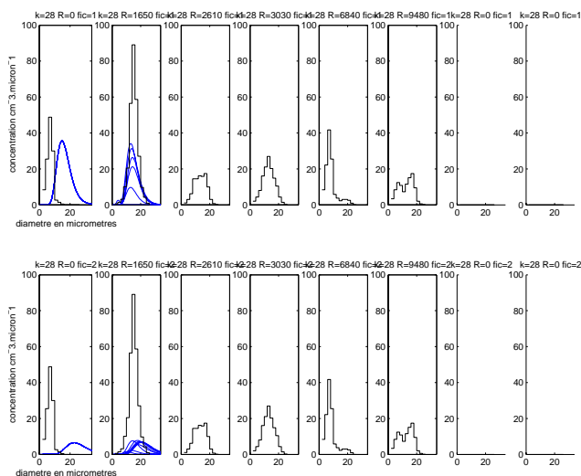
FIG. B.58 – Comparaison des spectres in-situ mesurés par l'avion (histogrammes en noir) avec les spectres simulés (courbe log-normales bleues). La ligne du haut correspond au cas continental, celle du bas au cas maritime. La première colonne correspond au premier spectre mesuré et au spectre simulé issu du point *. La seconde colonne correspond au spectre mesuré à la distance en mètres R (notée au dessus de chaque graphique) du premier spectre mesuré et aux courbes log-normales issues des petits cercles situés à la même distance R du point *. Idem pour la troisième, la quatrième, etc ... . Pour la localisation spatiale des spectres, voir figure B.56. Palier n°1.
