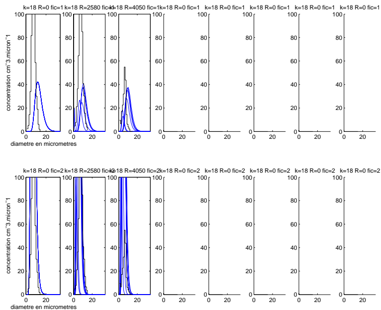
FIG. B.76 – Idem figure B.70. Palier n°11.
