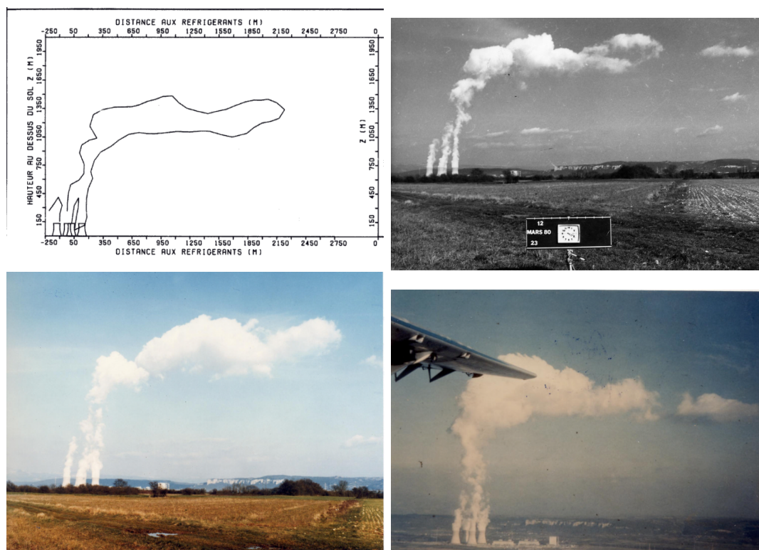
FIG. 7.4 – Le 12 mars 1980, croquis à 16h20 et photos à 16h19, 16h20 et 16h53 (de gauche à droite et de haut en bas).
