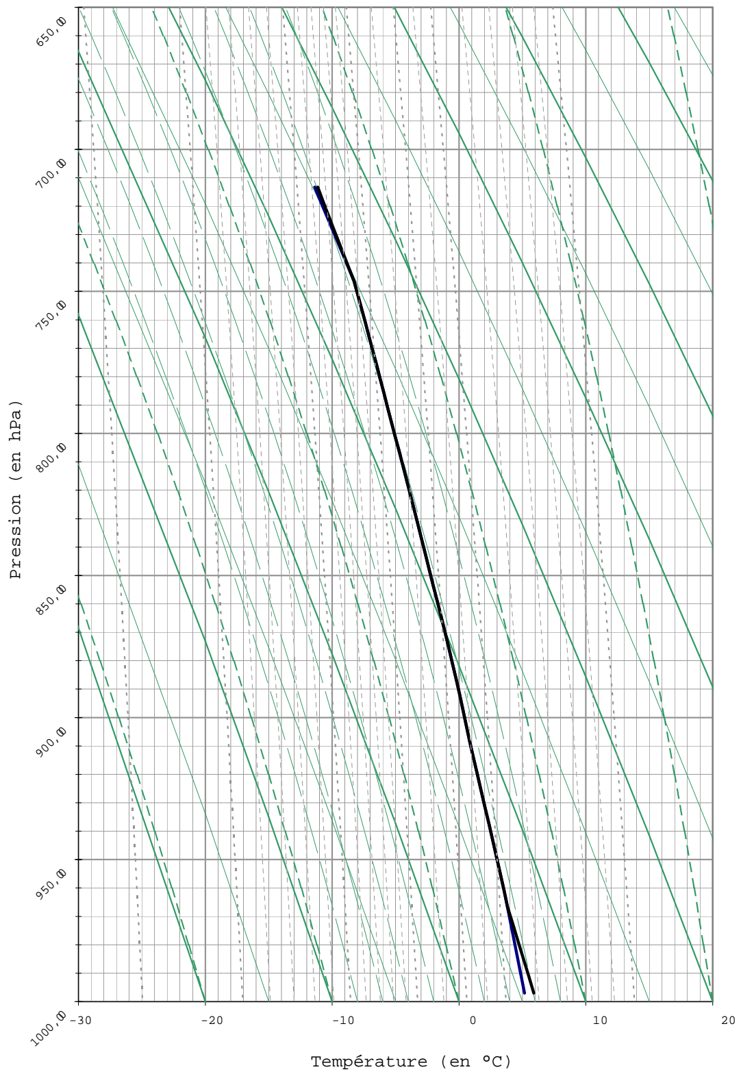
FIG. A.5 – Le 13 mars 1980 13h. Émagramme.
