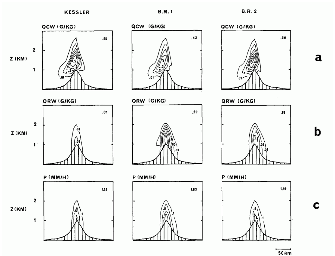
FIG. 12.10 – Coupes verticales des rapports de mélange de l'eau nuageuse q_c , de l'eau de pluie q_r et du taux de précipitations P pour la modélisation de Kessler, BR1 et BR2. Les valeurs maximales sont données dans le coin en haut à droite de chaque figure. (Tiré de la Fig. 6 de RC)
