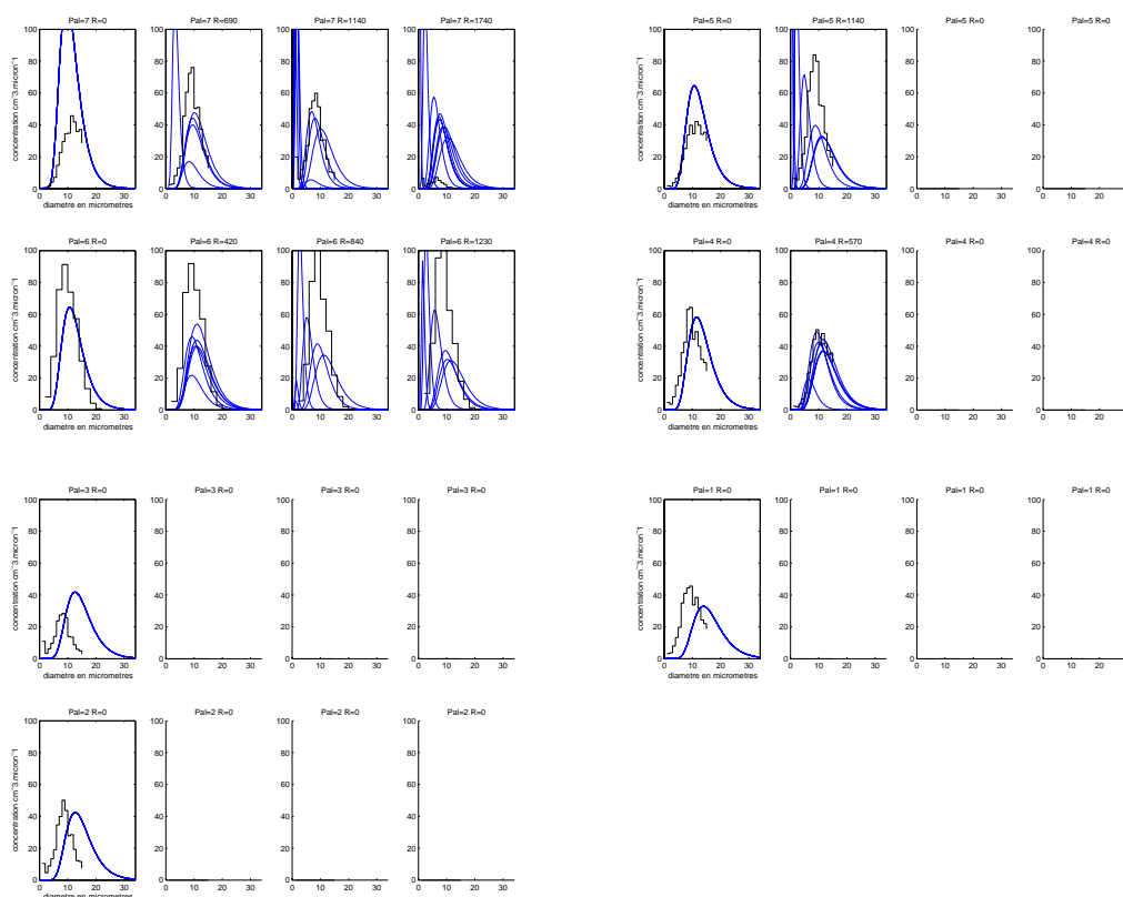
FIG. B.32 – Comparaison des spectres in-situ mesurés par l'avion (histogrammes en noir) avec les spectres simulés (courbe log-normales bleues) le 12 mars 1980 à 10h45. Représentation de la densité de concentration en cm^{-3} \cdot \mu m^{-1} en fonction du diamètre en \mu m . Sur chaque spectre est indiqué le numéro du palier "Pal" et la distance au premier point de mesure R (en m ). La première colonne correspond au premier spectre mesuré et au spectre simulé issu du point *. La seconde colonne correspond au spectre mesuré à la distance en mètres R du premier spectre mesuré et aux courbes log-normales issues des petits cercles situés à la même distance R du point *. Idem pour la troisième colonne, la quatrième, etc ... Pour la localisation spatiale des spectres, voir figure B.31.
