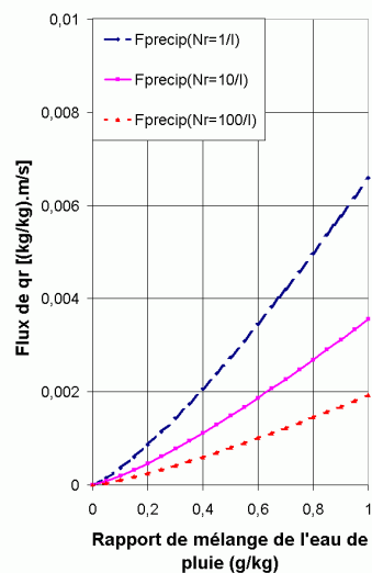
FIG. 11.4 – Idem Fig. 11.3 mais pour la modélisation du flux de précipitation utilisée dans le code MERCURE. Pour différentes valeurs de N_r (voir légende).
