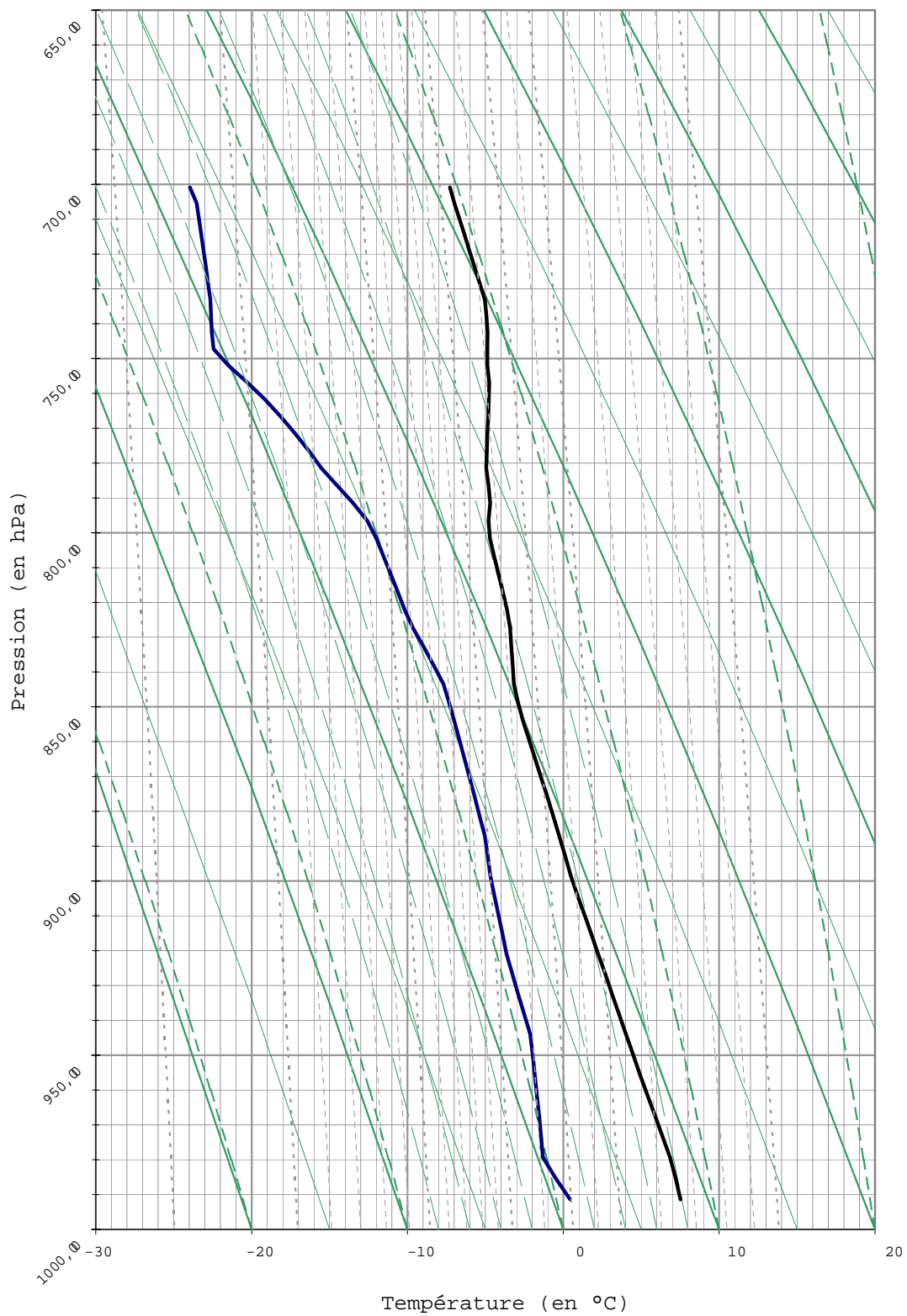
FIG. A.4 – Le 12 mars 1980 16h30. Émagramme.
