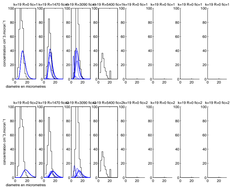
FIG. B.62 – Idem figure B.58. Palier n°4.
