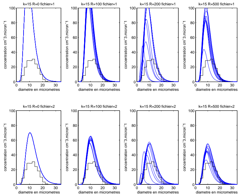
FIG. B.82 – Idem figure B.80. Palier n°6.
