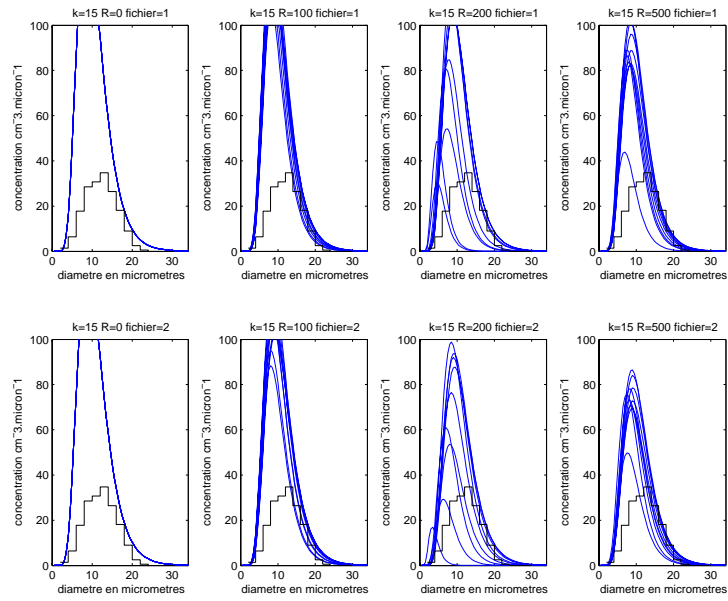
FIG. B.52 – Idem figure B.51. Palier n°4.
