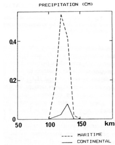
FIG. 12.7 – Cumul des précipitations, en cm , sur la durée de la simulation (6 heures) pour le cas maritime et continental . (Tiré de la Fig. 6. de l'article de CRPN).
