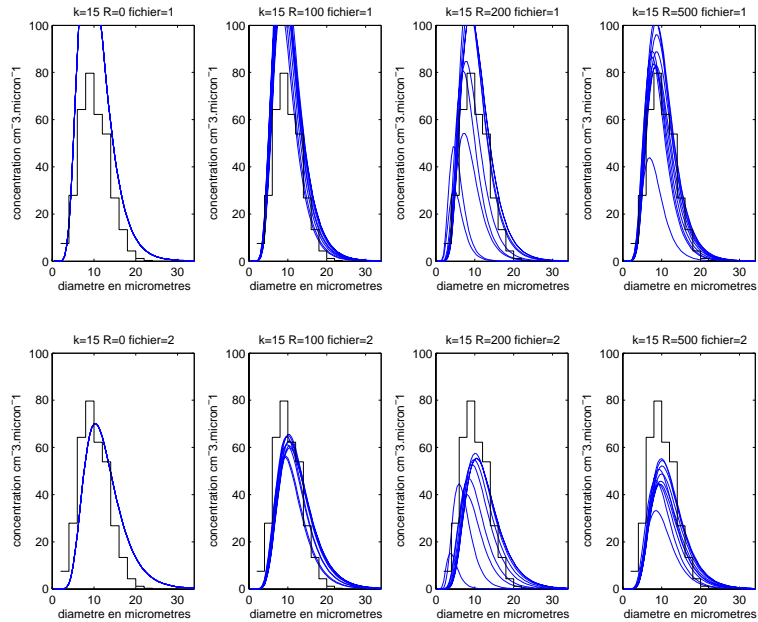
FIG. B.83 – Idem figure B.80. Palier n°7.
