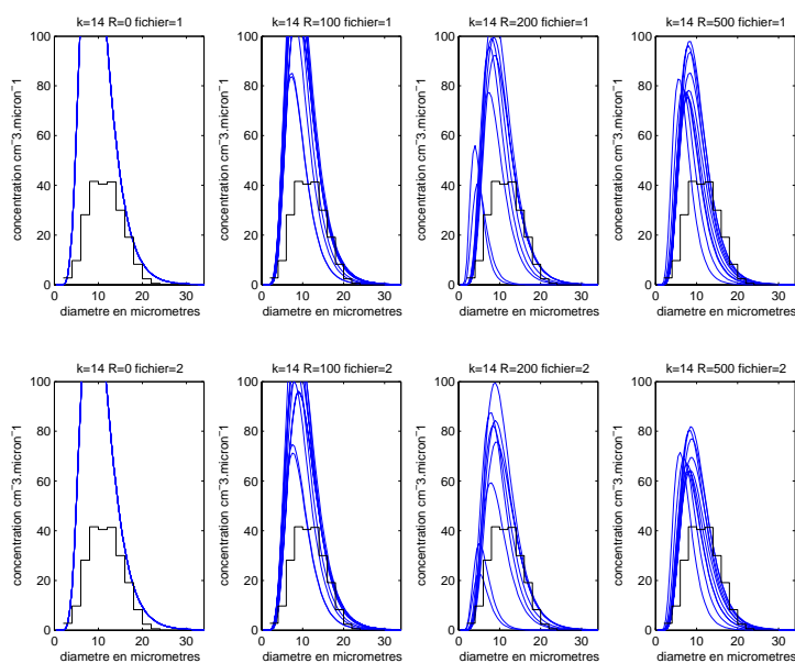
FIG. B.51 – Comparaison des spectres in-situ mesurés par l’avion (histogrammes en noir) avec les spectres simulés (courbe log-normales bleues). La ligne du haut correspond au cas continental, celle du bas au cas maritime. La première colonne correspond au spectre simulé issu du point *, la seconde aux spectres issus des petits cercles situés à 100 m du point *, la troisième aux spectres à 200 m et la quatrième aux spectres à 500 m. Pour la localisation des spectres, voir figure B.50. Le 4 mars 1980 11h, palier n°5.
