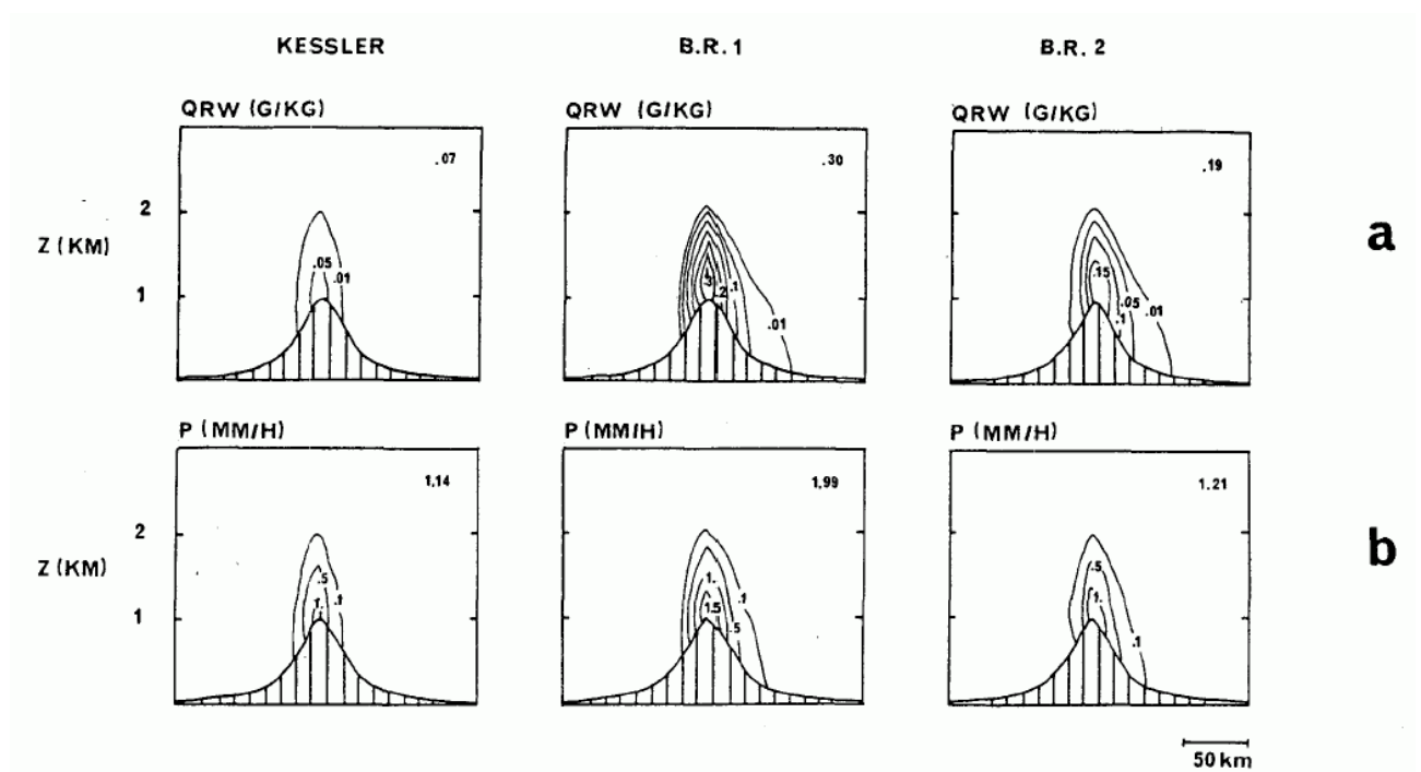
FIG. 12.15 – Idem que la figure 12.13 mais pour le run C. (Tiré de la Fig. 10 de RC)
