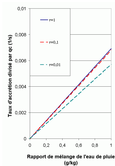
FIG. 11.2 – Idem Fig. 11.1 mais pour la modélisation de l'accrétion utilisée dans le code MERCURE. Pour différentes valeurs de \tau = \frac{q_r}{q_l} , où q_l = q_c + q_r ; notre modèle est indépendant de N_r .
