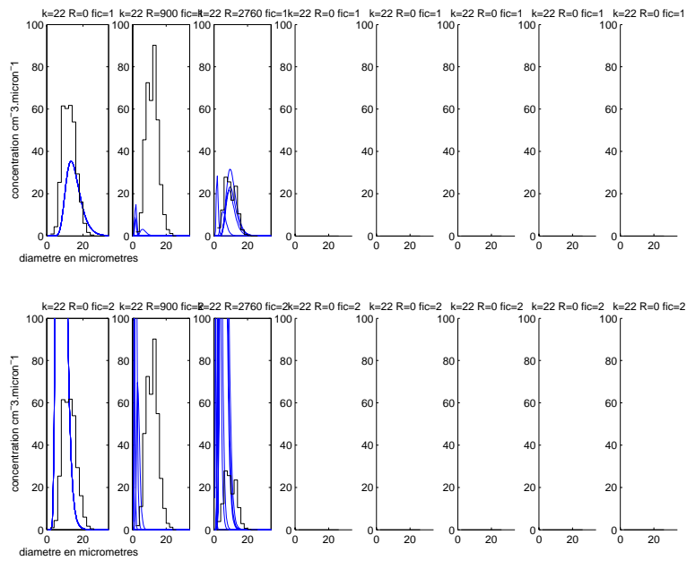
FIG. B.72 – Idem figure B.70. Palier n°3.
