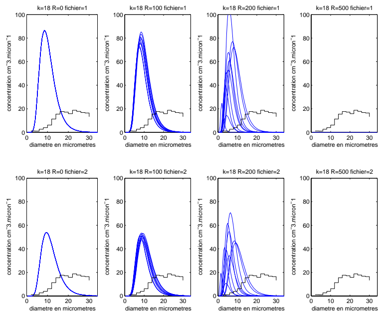
FIG. B.84 – Idem figure B.80. Palier n°9.
