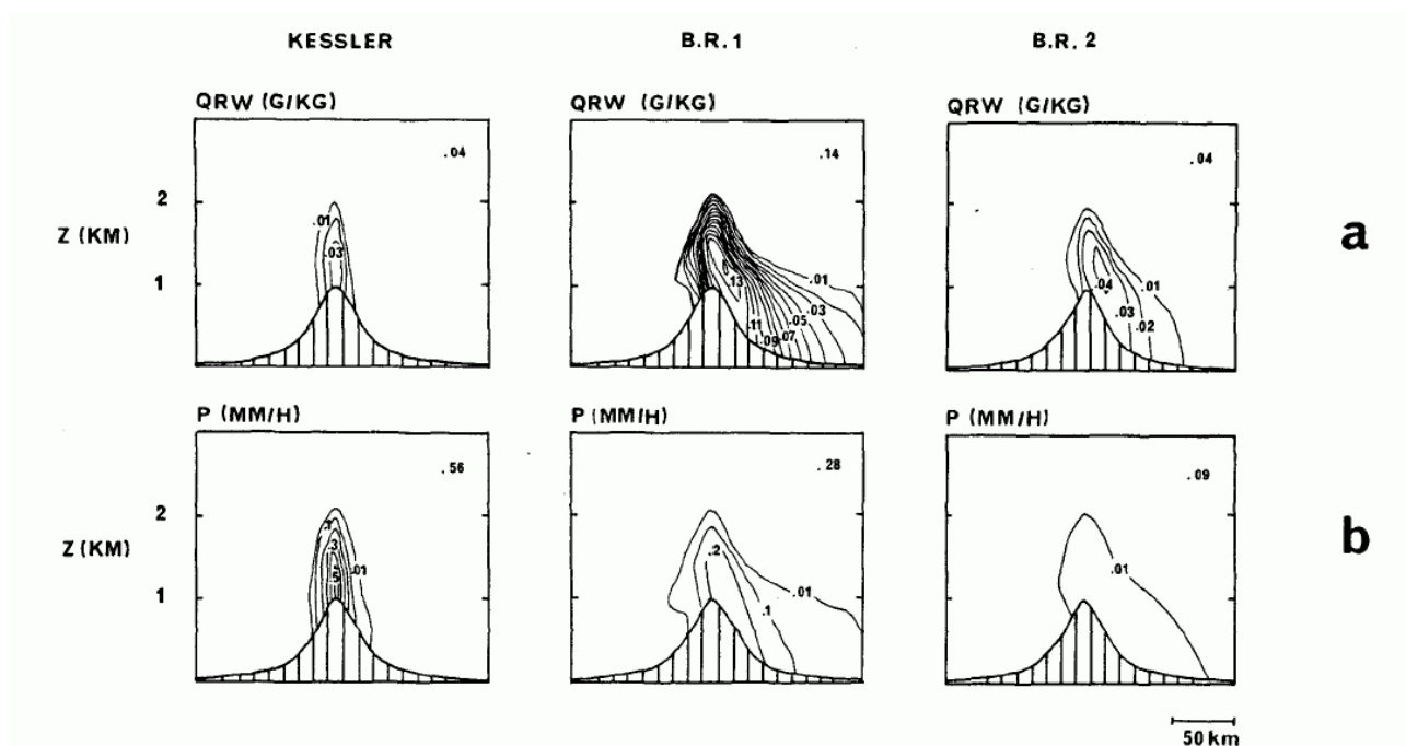
FIG. 12.13 – Coupes verticales du rapport de mélange q_r et du taux de précipitations P pour la modélisation de Kessler, BR1 et BR2 obtenus pour le run A. Les valeurs maximales sont données dans le coin en haut à droite de chaque figure. (Tiré de la Fig. 8 de RC)
