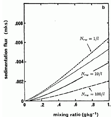
FIG. 11.3 – Flux de sédimentation (ou précipitation) du rapport de mélange de l’eau de pluie q_r en fonction de cette même variable q_r . Pour la modélisation de Kessler (1969) (trait fin) et pour la modélisation utilisée par RC, pour différentes valeurs de N_r (traits épais continus et épais tiretés). (Tiré de la figure 4.b de RC).
