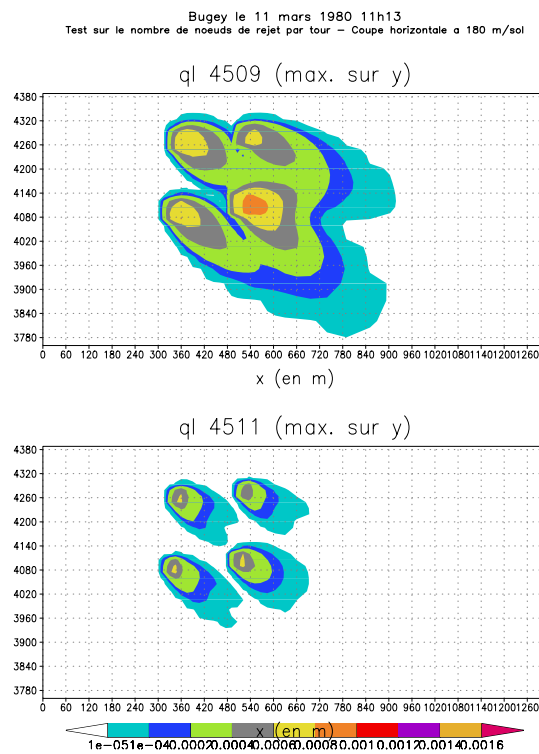
FIG. 8.6 – Coupe horizontale au niveau de la maille immédiatement supérieure à la maille de rejet. Nous présentons les fractions massiques en eau liquide nuageuse (en kg/kg). En haut, pour la modélisation standard, en bas pour la modélisation sur 9 nœuds uniquement.
