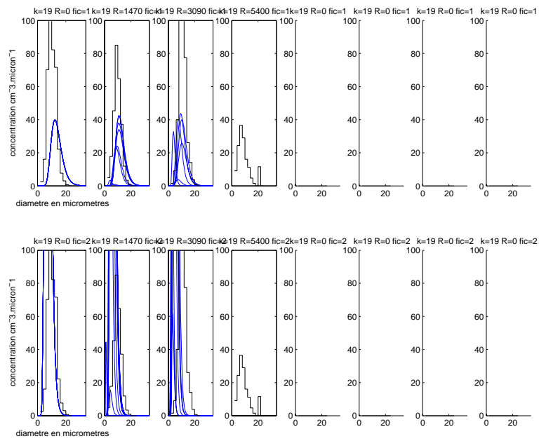
FIG. B.74 – Idem figure B.70. Palier n°4.
