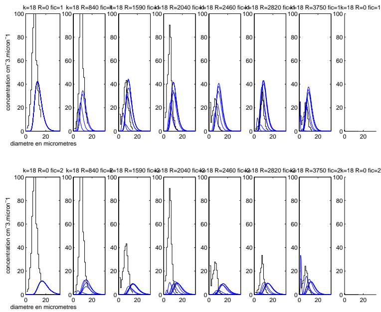
FIG. B.64 – Idem figure B.58. Palier n°9.
