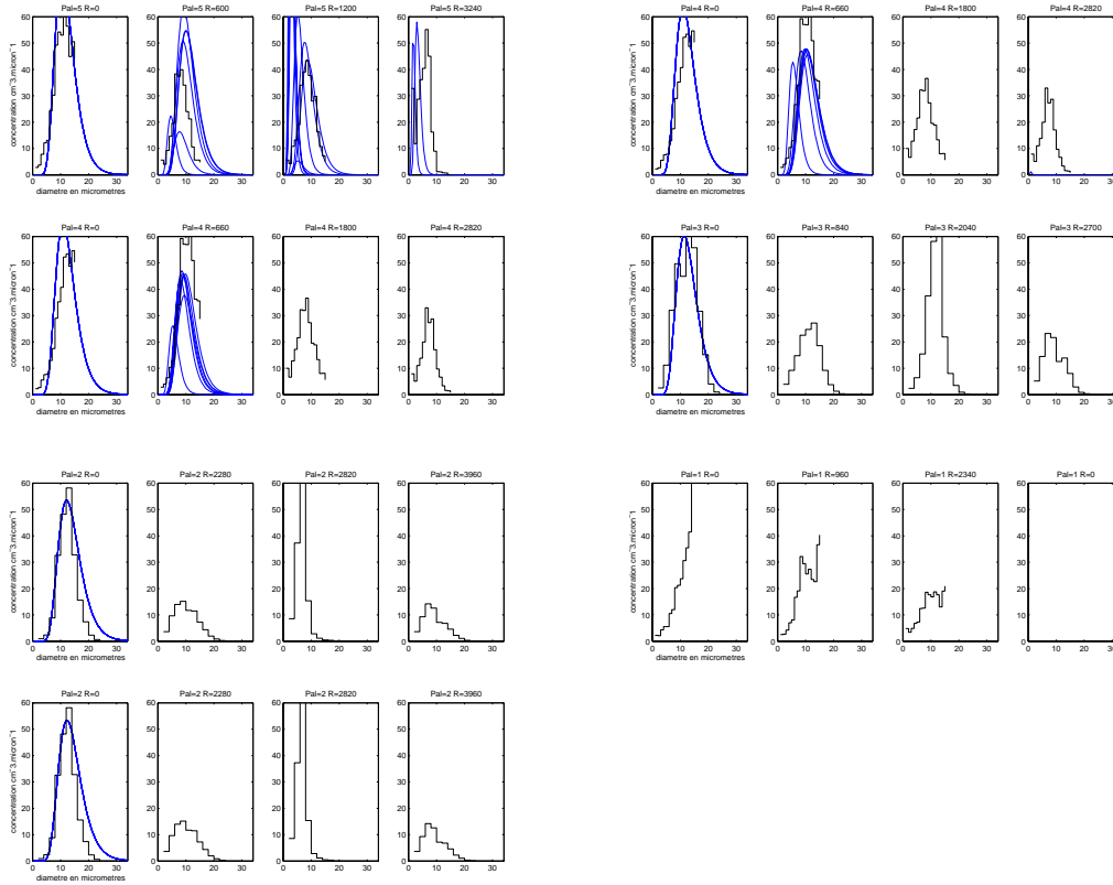
FIG. B.34 – Comparaison des spectres in-situ mesurés par l'avion (histogrammes en noir) avec les spectres simulés (courbe log-normales bleues) le 13 mars 1980 à 16h30 avec correction de la température ambiante et pour des valeurs de turbulence au rejet non standards ( \nu_t = 90 \text{ m}^2/\text{s} ). Représentation de la densité de concentration en \text{cm}^{-3} \cdot \mu\text{m}^{-1} en fonction du diamètre en \mu\text{m} . Sur chaque spectre est indiqué le numéro du palier "Pal" et la distance au premier point de mesure R (en \text{m} ). La première colonne correspond au premier spectre mesuré et au spectre simulé issu du point *. La seconde colonne correspond au spectre mesuré à la distance en mètres R du premier spectre mesuré et aux courbes log-normales issues des petits cercles situés à la même distance R du point *. Idem pour la troisième colonne, la quatrième, etc ... . Pour la localisation spatiale des spectres, voir figure B.33.
