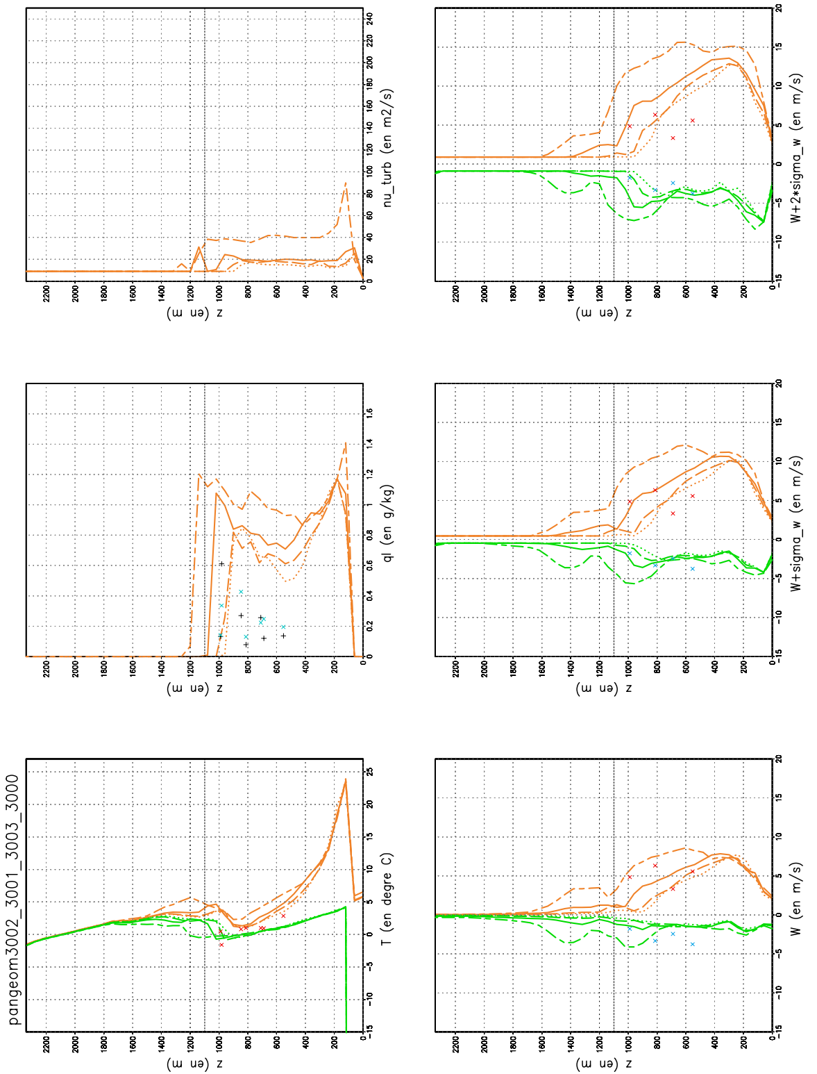
FIG. B.18 – Le 27 février 1980 16h04. "Tableau de bord" sur la sensibilité à la turbulence au rejet.
