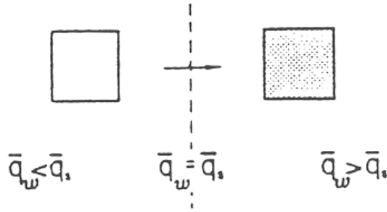
FIG. 4.1 – Schéma de condensation "tout ou rien"
