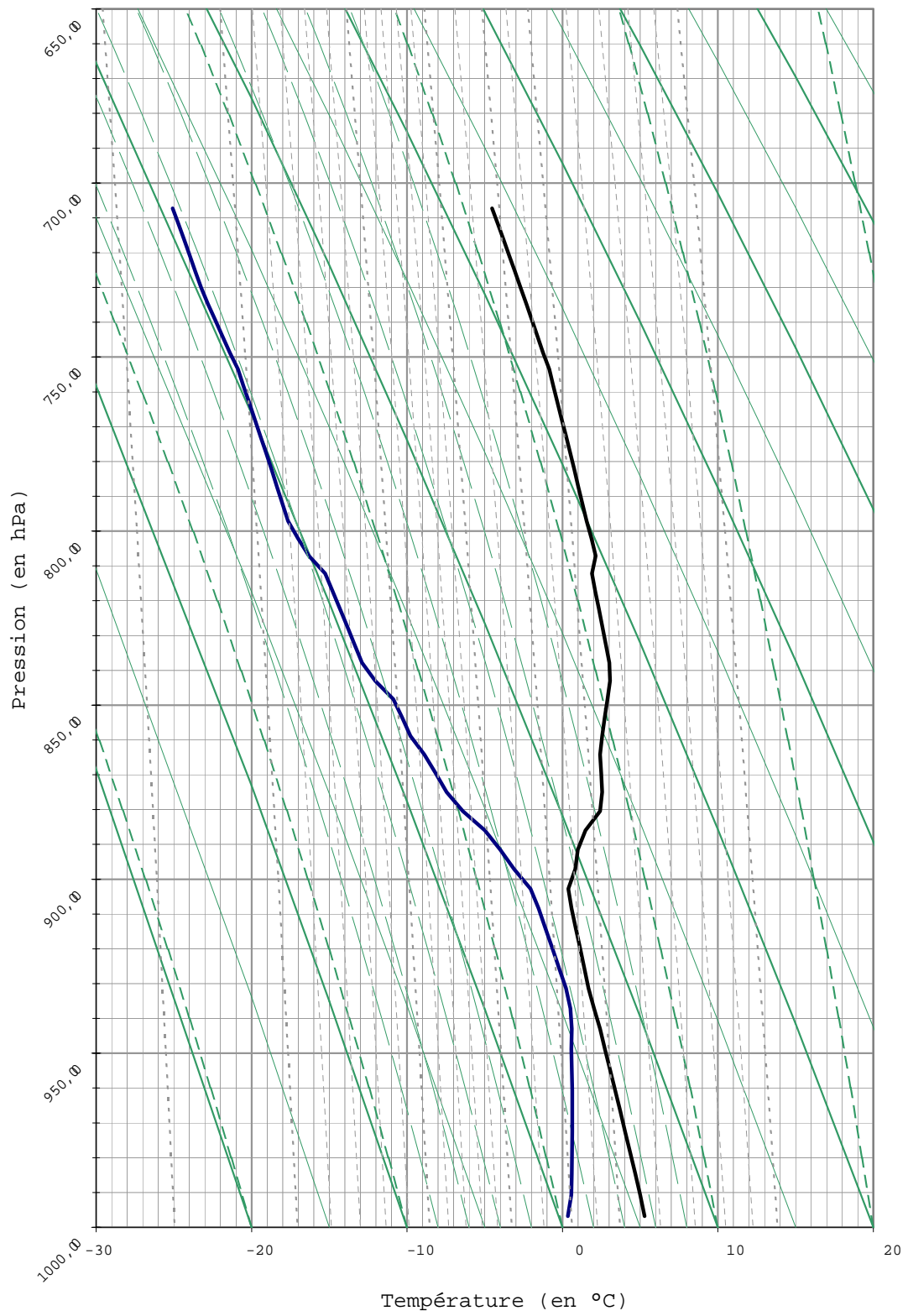
FIG. A.1 – Le 27 février 1980 16h04. Émagramme.
