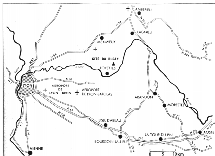
FIG. 6.3 – Plan de la région du Bugey. Localisation du site du Bugey et des localités où sont effectués les radiosondages (Loyettes et l'aéroport de Satolas).
