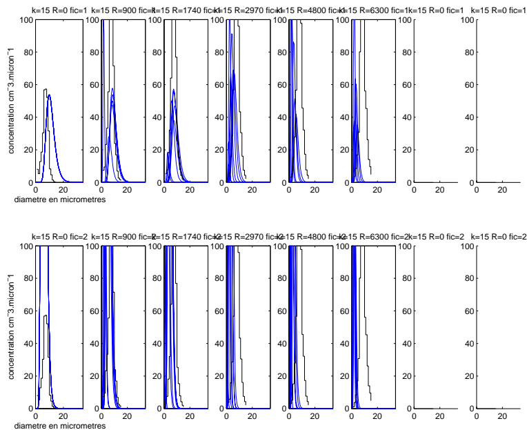
FIG. B.78 – Idem figure B.70. Palier n°5.
