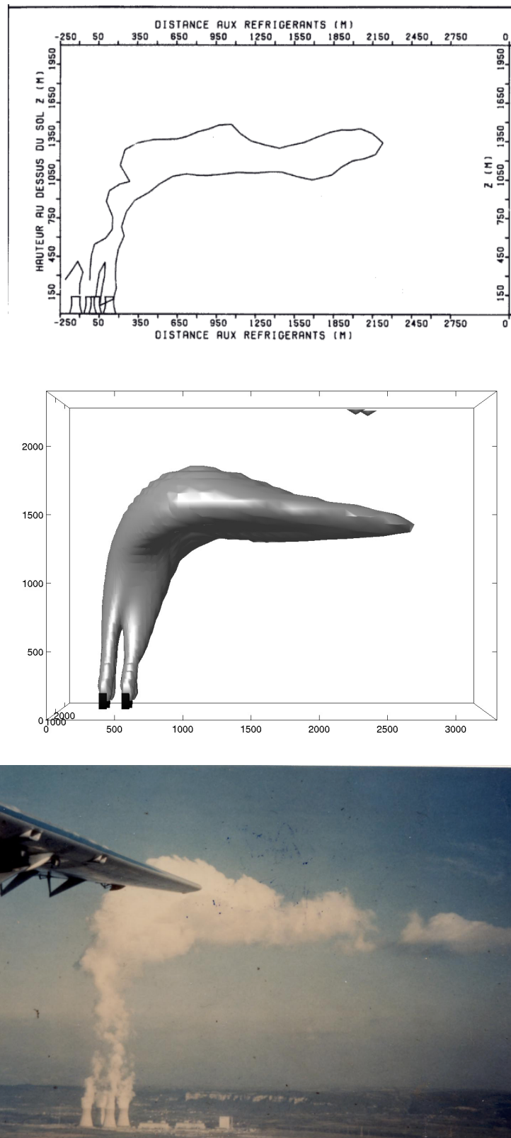
FIG. 7.3 – Le 12 mars 1980, photo 16h53 et croquis à 16h20, simulation réalisée à 16h30.
