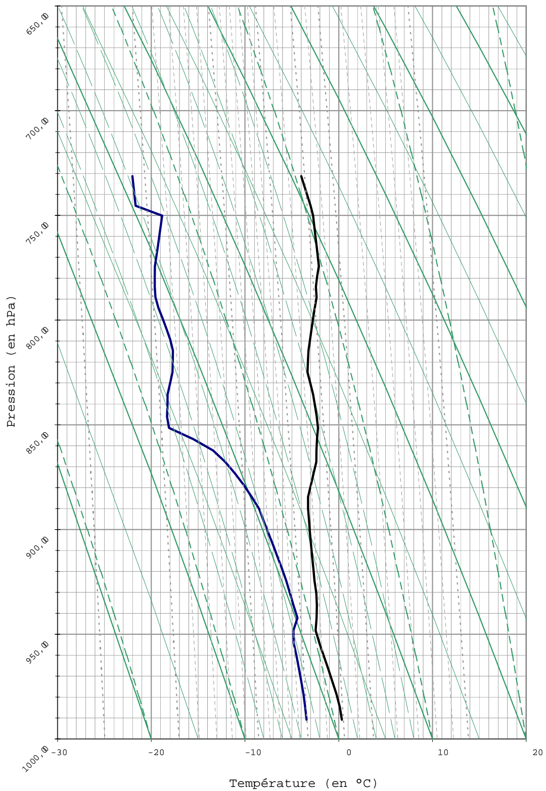
FIG. A.2 – Le 04 mars 1980 11h00. Émagramme.
