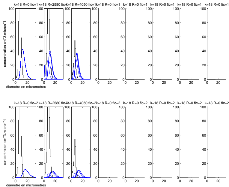
FIG. B.65 – Idem figure B.58. Palier n°11.
