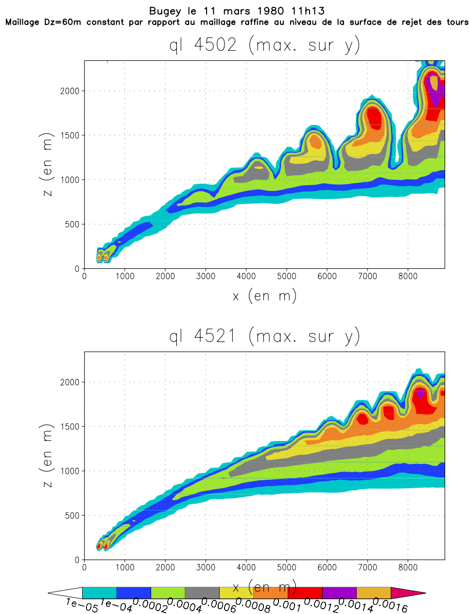
FIG. 8.4 – Le 11 mars 1980 11h13, test sur la résolution du maillage. Figure du haut : cas avec le maillage standard \Delta Z constant ( \Delta Z = 60m ). Figure du bas : cas avec un maillage raffiné à la hauteur du rejet \Delta Z = 15m de part et d'autre de Z = 128m et \Delta Z augmente progressivement vers le sol et le sommet de domaine ( \Delta Z_{max} = 100m ).
