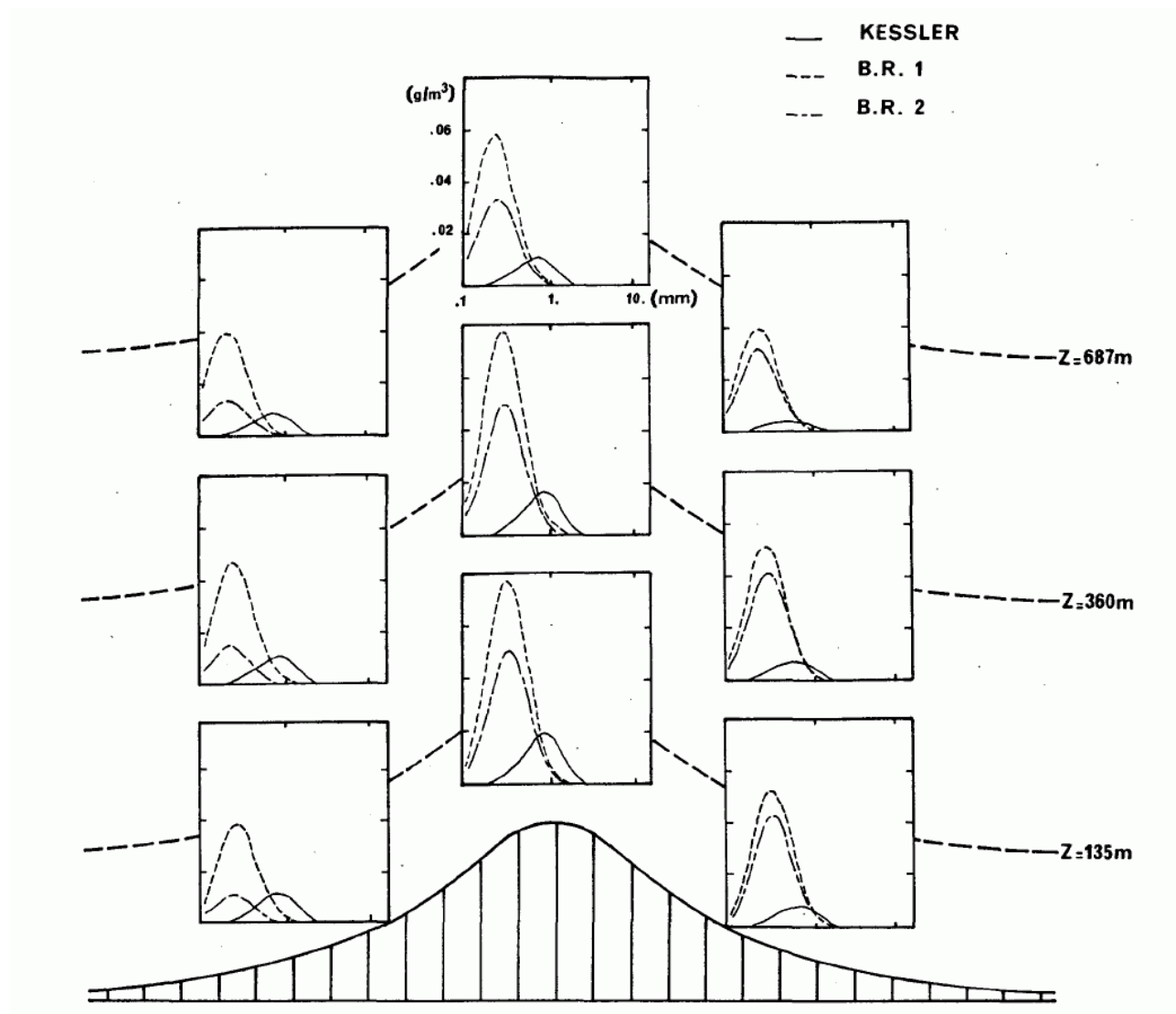
FIG. 12.19 – Fonctions de densité en masse pour les gouttes de pluie, obtenues avec Kessler, BR1 et BR2 pour trois points de grille situés au sommet, à l'amont et à l'aval de la montagne et pour trois niveaux verticaux du modèle ( Z = 135, 360 et 687m au dessus du sol). (Tiré de la Fig. 7 de RC).
