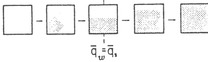
FIG. 4.2 – Schéma de condensation à l'échelle sous-maille
