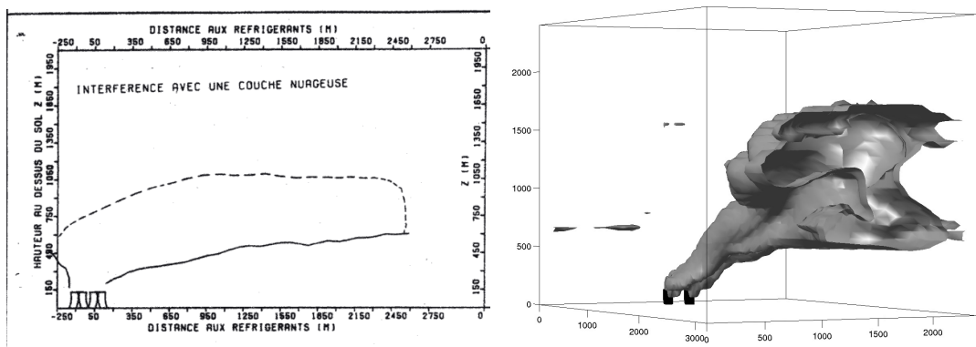
FIG. B.15 – Le 12 mars 1980, croquis à 10h55 et simulation réalisé à 10h45.
