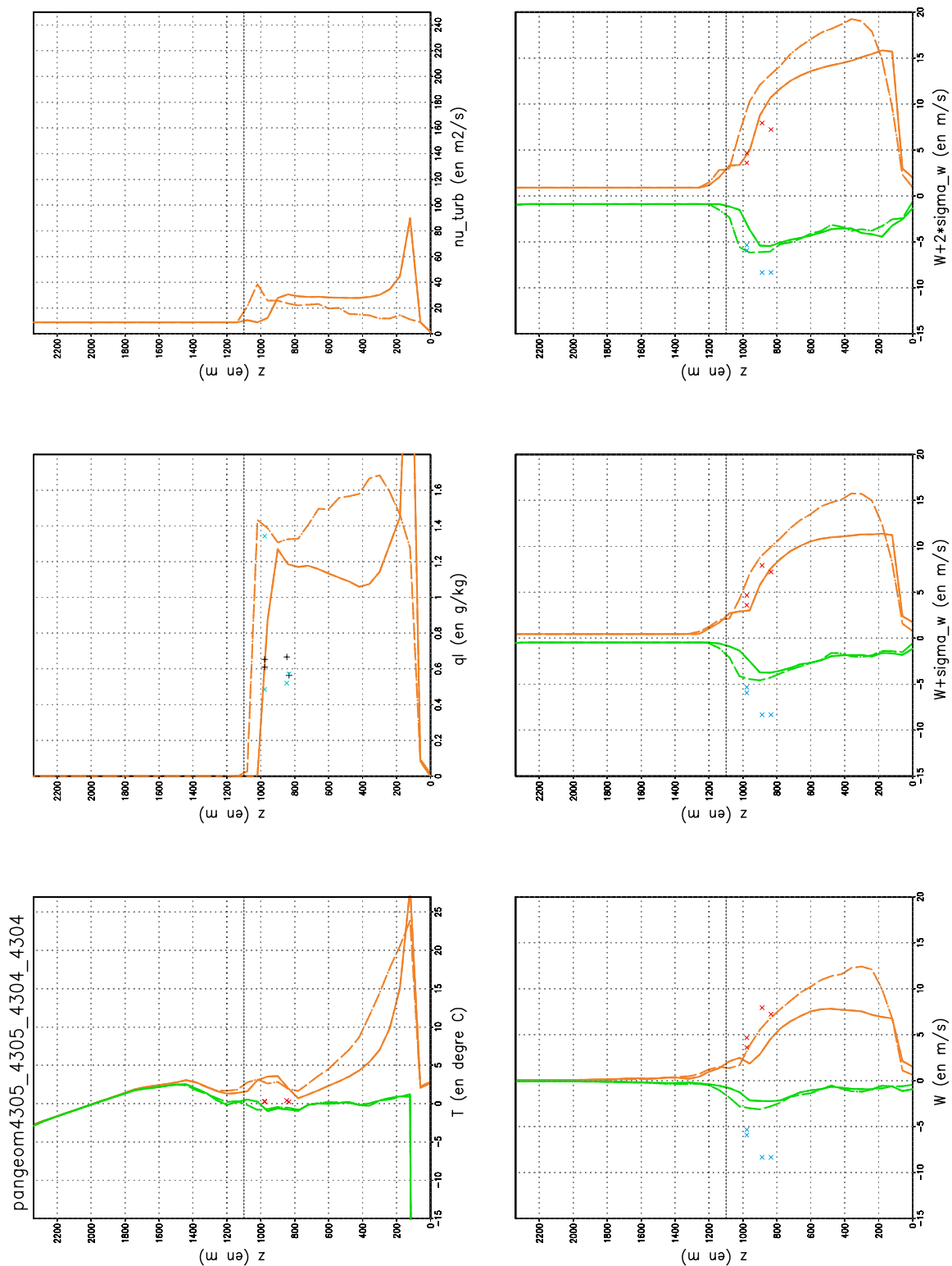
FIG. B.39 – Le 27 février 1980 10h45. "Tableau de bord" sur la modélisation du rejet, légende page 272.
