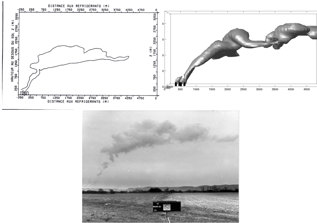
FIG. B.14 – Le 10 mars 1980, photo à 16h52, croquis à 16h55 et simulation réalisé à 17h00.
