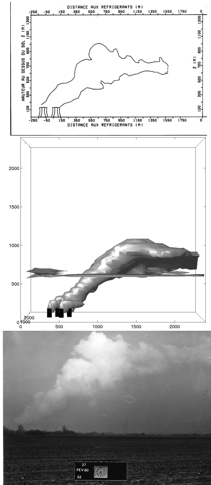
FIG. 7.2 – Le 27 février 1980, photo et croquis à 17h38, simulation réalisé à 16h04.
