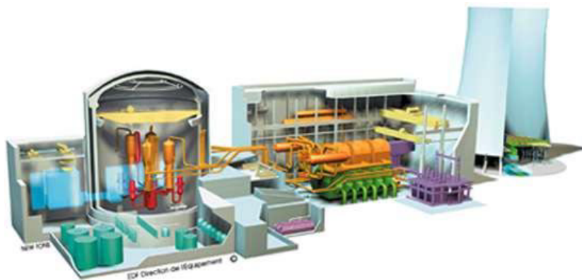
FIG. 5.1 – Du cœur de réacteur aux tours de réfrigération.
