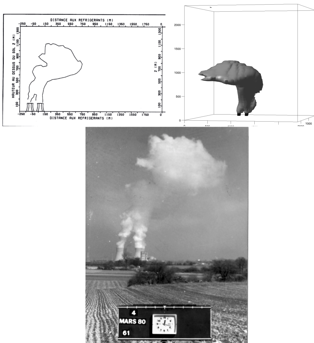
FIG. B.11 – Le 4 mars 1980, croquis et simulation réalisé à 12h15, photo à 12h18.
