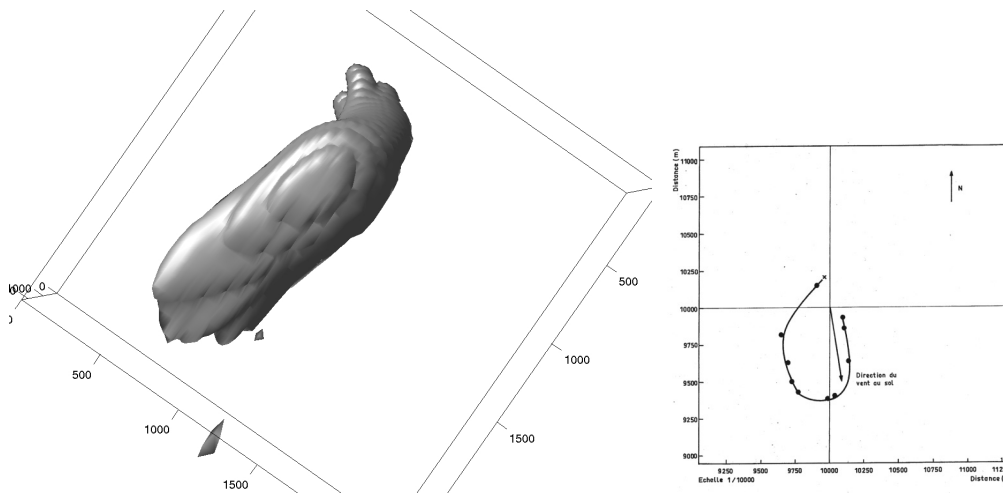
FIG. 7.14 – Le 4 mars 1980, photogramm trie   10h35, simulation r alis e   11h00. Vue de dessus.
