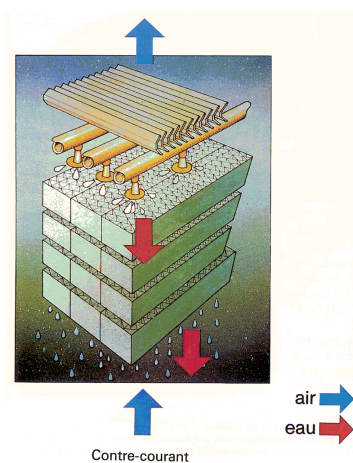
FIG. 5.3 – Zone d'échange à l'intérieur des aéroréfrigérants
