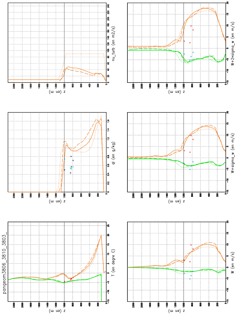
Bugey le 04 mars 1980 11h Tests de sensibilité k-epsilon en conditions aux limites meteorologiques
