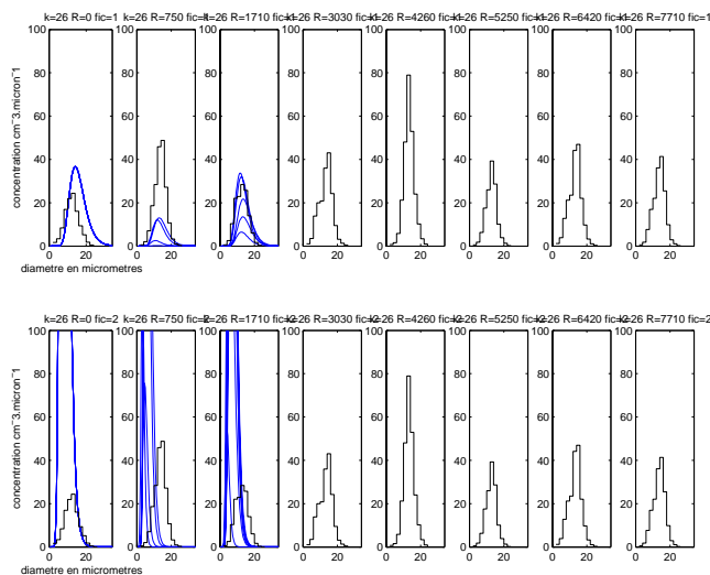
FIG. B.71 – Idem figure B.70. Palier n°2.
