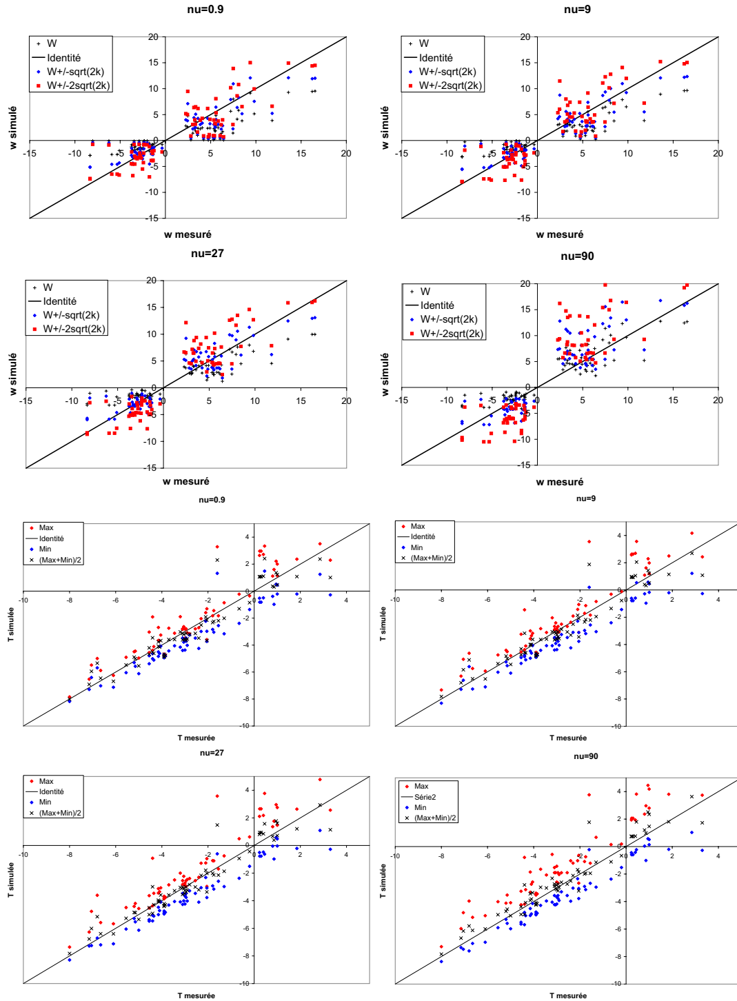
FIG. 8.2 – Synthèse des comparaisons entre les mesures et les simulations pour la vitesse verticale instantanée maximale et minimale w et son estimation par W , W \pm \sqrt{2k} et W \pm 2\sqrt{2k} (en haut) et pour la température moyenne T lors des traversées du panache (en bas). Simulations réalisées avec différentes valeurs de turbulence au rejet, la valeur de \nu_t utilisée est indiquée au dessus de chaque graphique.
