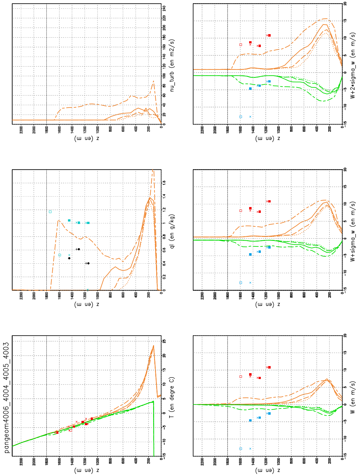
Bugey le 13 mars 1980 16h30 (T modifiée) Tests de sensibilité k-epsilon au rejet
