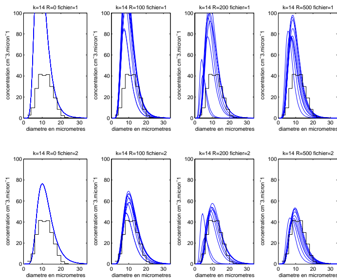
FIG. B.80 – Comparaison des spectres in-situ mesurés par l’avion (histogrammes en noir) avec les spectres simulés (courbe log-normales bleues). La ligne du haut correspond au cas N_c = 1.10^4 \text{ cm}^{-3} en sortie des tours, celle du bas N_c = 5.10^3 \text{ cm}^{-3} au cas . La première colonne correspond au spectre simulé issu du point *, la seconde aux spectres issus des petits cercles situés à 100 m du point *, la troisième aux spectres à 200 m et la quatrième aux spectres à 500 m. Pour la localisation des spectres, voir figure B.56. Palier n°5.
