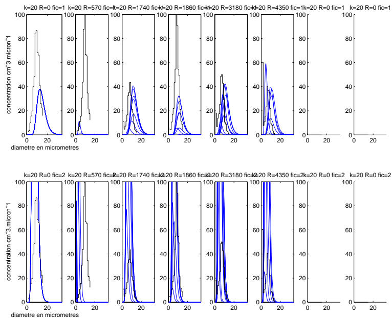
FIG. B.73 – Idem figure B.70. Palier n°8.
