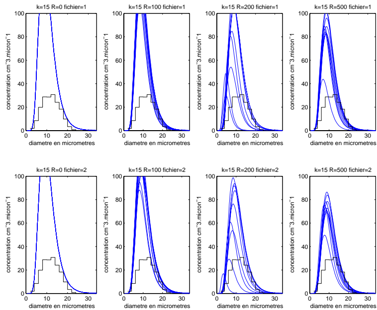
FIG. B.53 – Idem figure B.51. Palier n°6.
