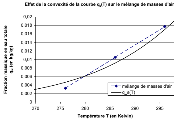
FIG. 7.19 – Effet de la convexité sur le mélange de masse d'air de la courbe de la fraction massique de vapeur d'eau à saturation en fonction de la température à pression constante P = 1000hPa .
