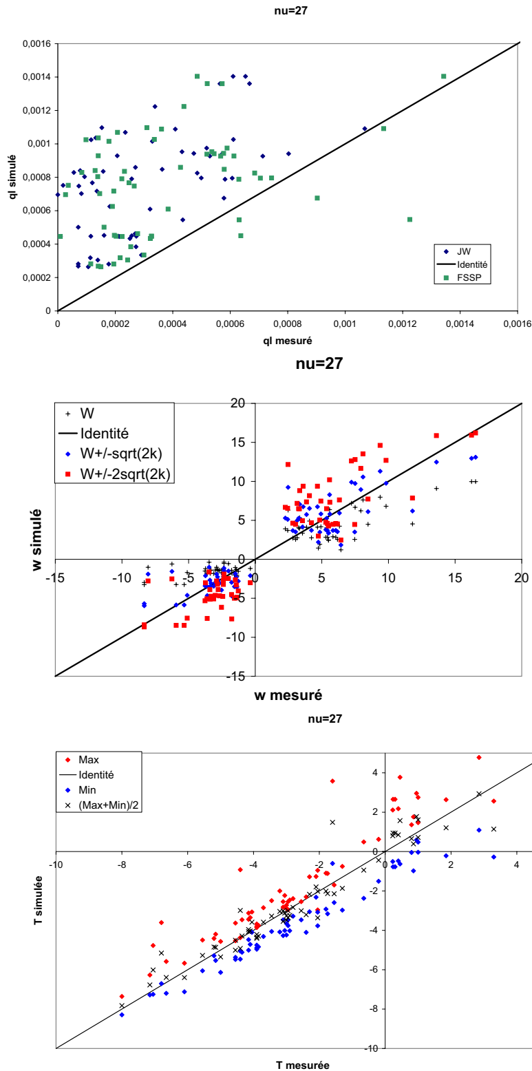
FIG. 7.20 – Synthèse des comparaisons entre les mesures et les simulations pour le contenu spécifique en eau liquide maximal q_l , la vitesse verticale instantanée maximale et minimale w et son estimation par W , W \pm \sqrt{2k} et W \pm 2\sqrt{2k} et la température moyenne T lors des traversées du panache.
