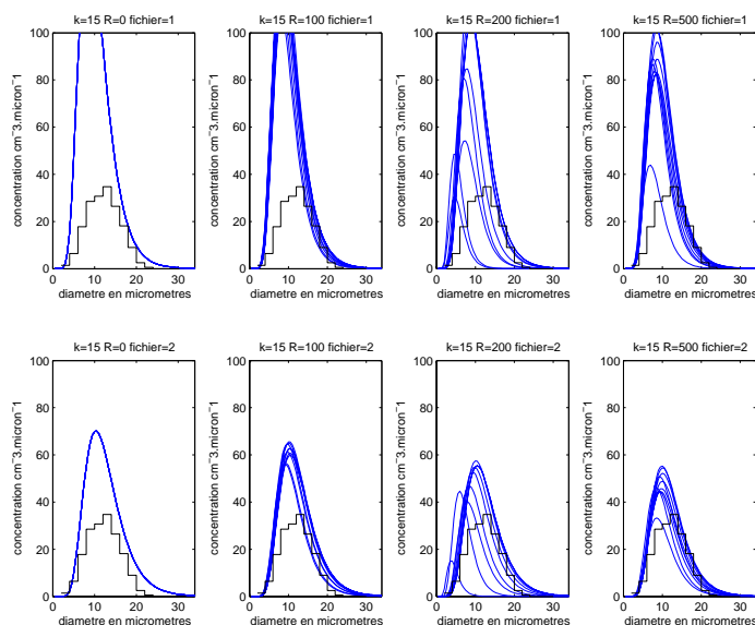
FIG. B.81 – Idem figure B.80. Palier n°4.
