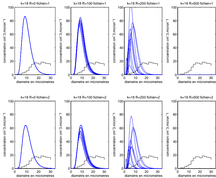
FIG. B.55 – Idem figure B.51. Palier n°9.
