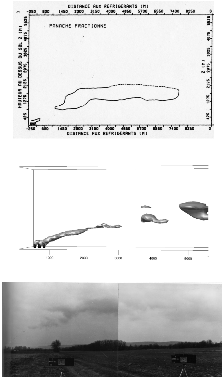
FIG. B.8 – Le 3 mars 1980, photo et croquis à 12h50 et simulation réalisé à 11h33.
