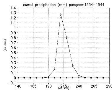
FIG. 12.8 – Idem Fig 12.7 pour les sorties MERCURE avec le même maillage que celui de CRPN.
