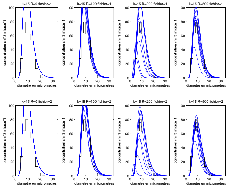
FIG. B.54 – Idem figure B.51. Palier n°7.
