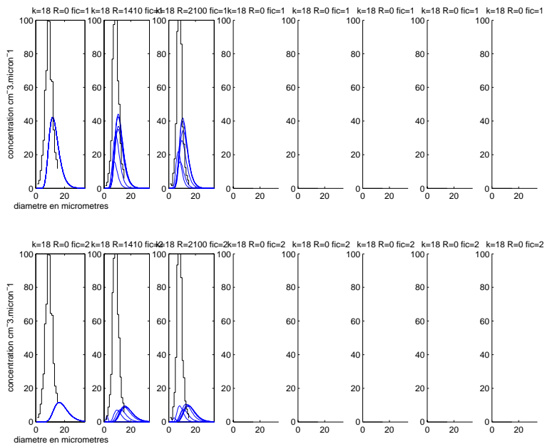
FIG. B.63 – Idem figure B.58. Palier n°7.
