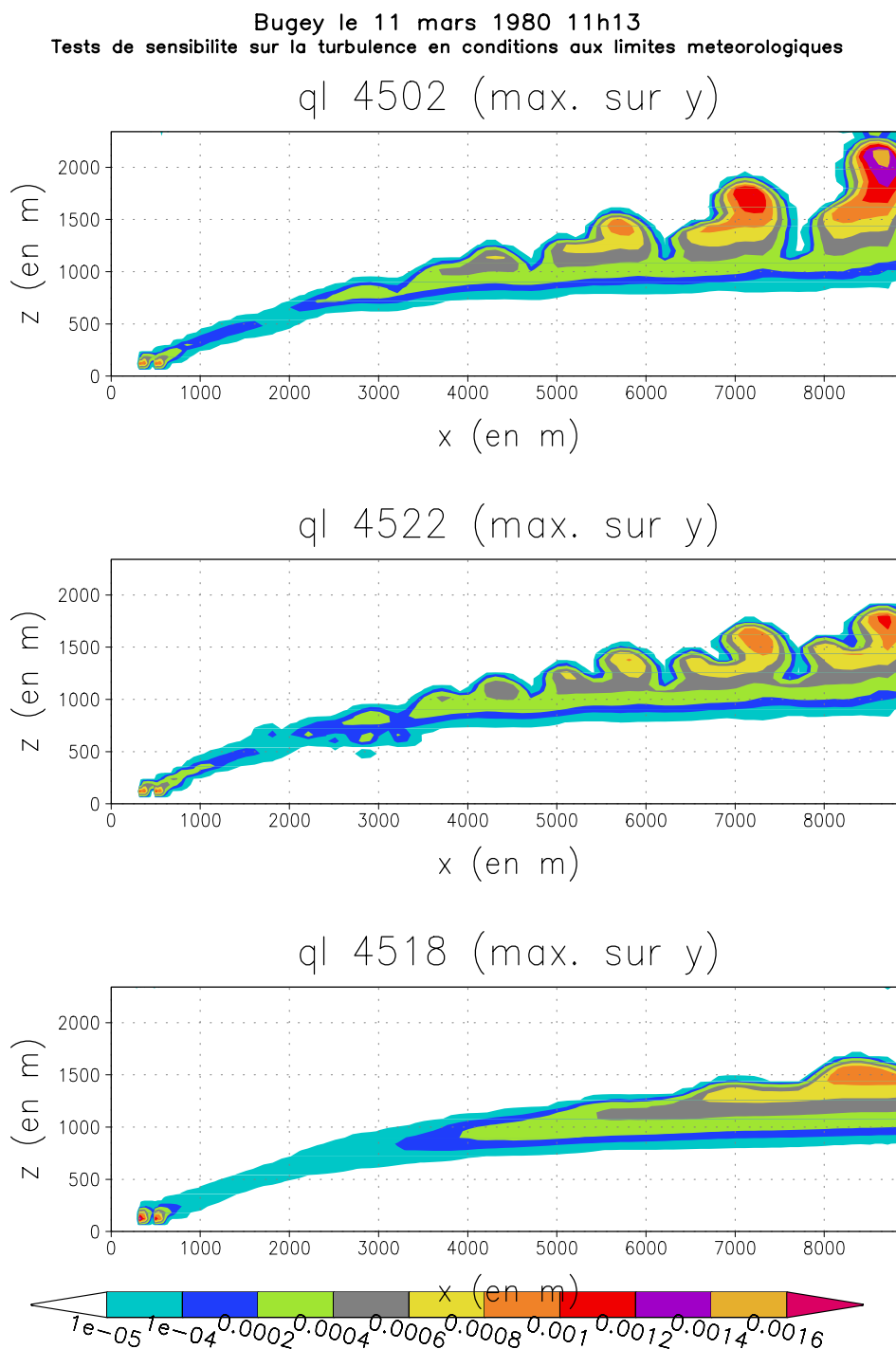
FIG. 8.3 – Le 11 mars 1980 11h13, test sur le profil de turbulence atmosphérique. On représente ici le maximum du contenu en eau liquide q_l selon l'axe horizontal Y . Figure du haut : cas avec un profil vertical de k et de \varepsilon standard ( k = 0.1m^2.s^{-2} et \varepsilon = 0.0001m^2.s^{-3} ). Figure du milieu : cas avec un profil vertical de k et de \varepsilon diagnostiqué à partir de formules de Musson-Genon (1995). Figure du bas : cas avec un profil de k et de \varepsilon modifié de 0 à 1000 m au dessus du sol, par rapport au profil standard ( k = 1m^2.s^{-2} et \varepsilon = 0.001m^2.s^{-3} ).
