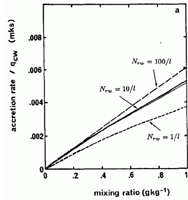
FIG. 11.1 – Taux d'accrétion divisé par le rapport de mélange de l'eau nuageuse q_c en fonction du rapport de mélange de l'eau de pluie q_r . Pour la modélisation de Kessler (1969) (trait fin) et pour la modélisation de Berry et Reinhardt (1974, Part III), utilisée par RC, pour différentes valeurs de N_r (traits épais continus et épais tiretés). (Tiré de la figure 4.a de RC).
