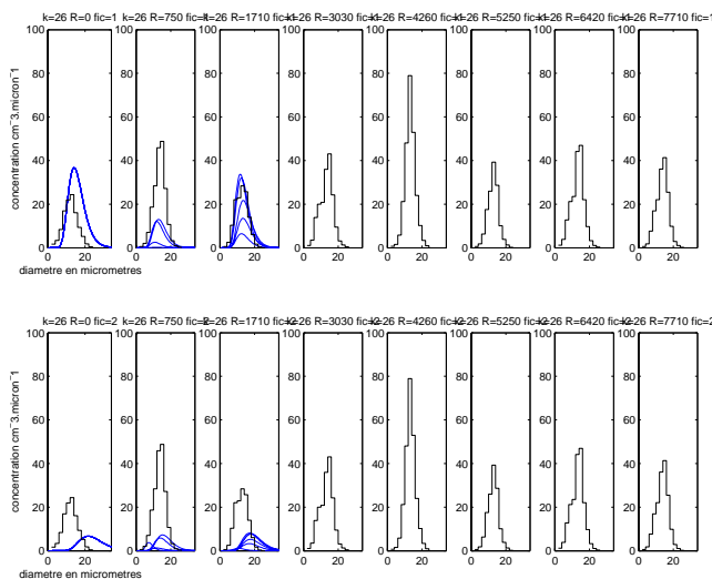
FIG. B.59 – Idem figure B.58. Palier n°2.
