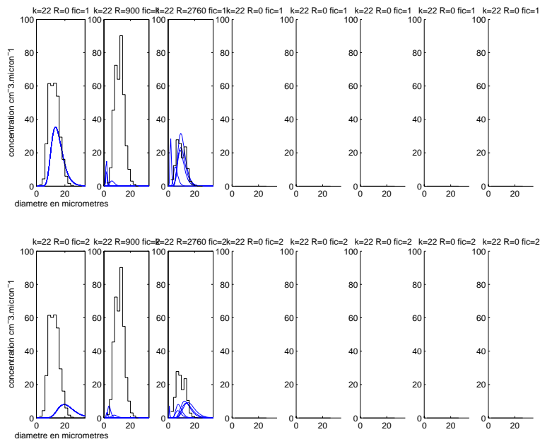
FIG. B.60 – Idem figure B.58. Palier n°3.
