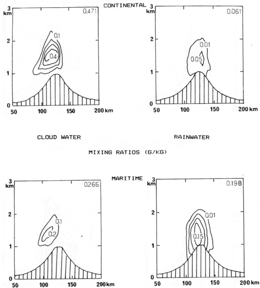
FIG. 12.4 – Coupe verticale de la fraction massique d'eau liquide nuageuse q_c et de l'eau de pluie q_r (de gauche à droite) pour le cas continental et maritime (de haut en bas). (Tiré de la Fig. 5. de l'article de CRPN).
