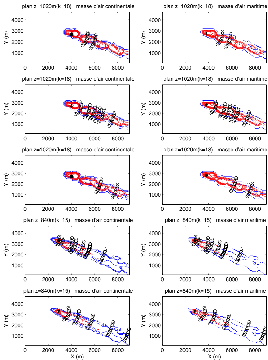
FIG. B.57 – Idem figure B.56 mais pour des paliers plus bas, de 1020 à 840 m , indiquée en haut à droite de chaque figures.
