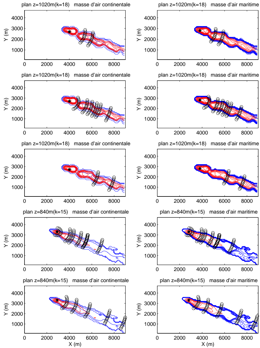
FIG. B.69 – Idem figure B.56 mais pour des paliers plus bas, de 1020 à 840 m , indiquée en haut à droite de chaque figures.
