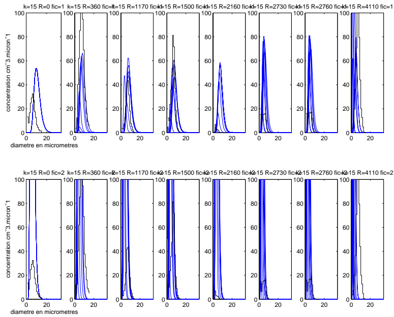
FIG. B.77 – Idem figure B.70. Palier n°10.
