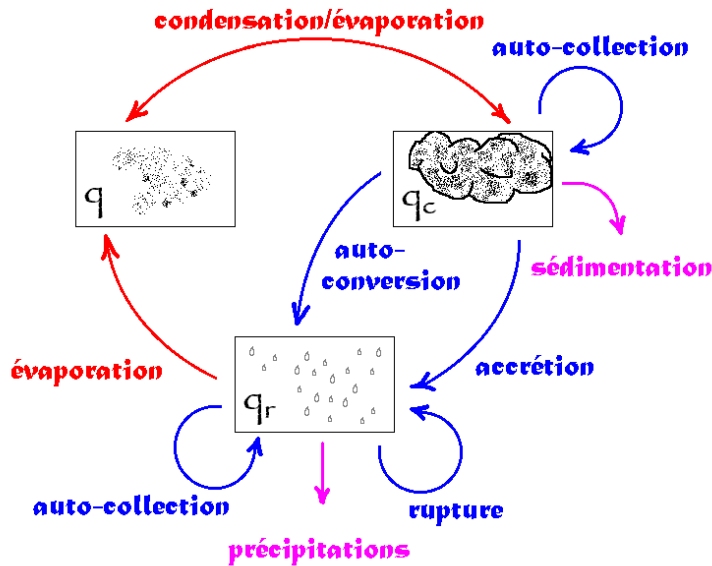
FIG. 3.1 – Schéma des flux de masse entre la vapeur d'eau q , l'eau liquide nuageuse q_c et l'eau de pluie q_r . Sur ce schéma la nucléation est incluse dans le terme de condensation entre la vapeur d'eau et l'eau liquide nuageuse.
