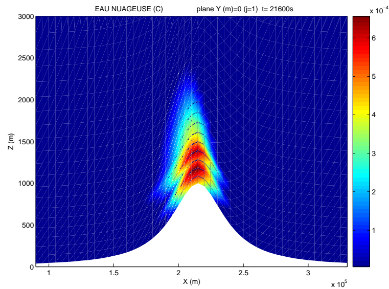
FIG. 9.1 – Simulation du nuage continental de CRPN mais avec un maillage fin. Visualisation du contenu en l'eau liquide nuageuse en (kg/kg).
