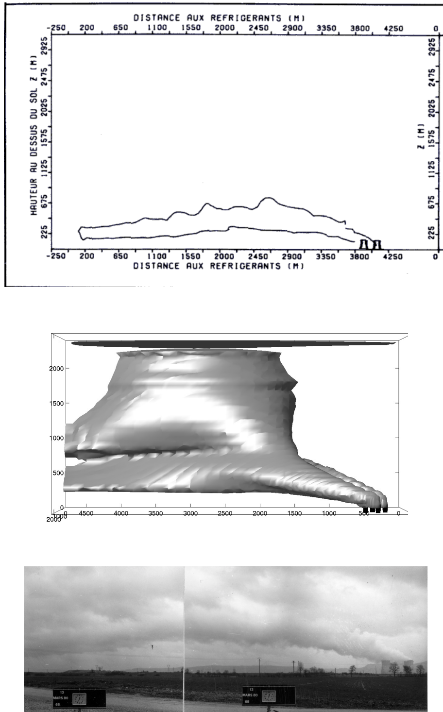
FIG. 7.5 – Le 13 mars 1980, photo et croquis à 12h35 et simulation réalisé à 13h00.
