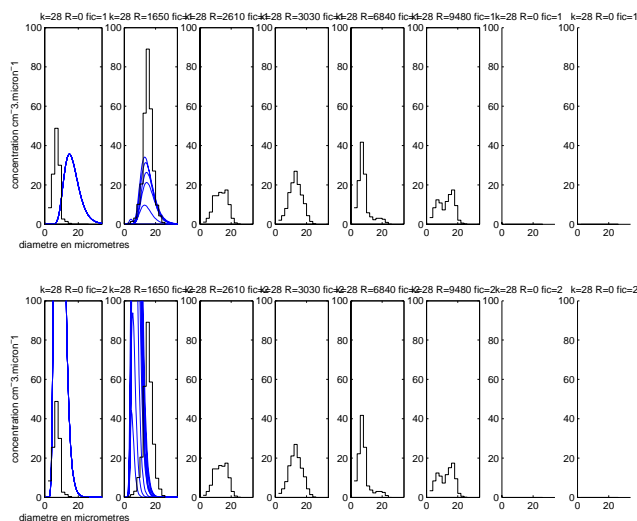
FIG. B.70 – Comparaison des spectres in-situ mesurés par l’avion (histogrammes en noir) avec les spectres simulés (courbe log-normales bleues). La ligne du haut correspond au cas continental, celle du bas au cas pollué. La première colonne correspond au premier spectre mesuré et au spectre simulé issu du point *. La seconde colonne correspond au spectre mesuré à la distance en mètres R (notée au dessus de chaque graphique) du premier spectre et aux courbes log-normales issues des petits cercles situés à la même distance R du point *. Idem pour la troisième, la quatrième, etc ... Pour la localisation spatiales des spectres, voir figure B.56. Palier n°1.
