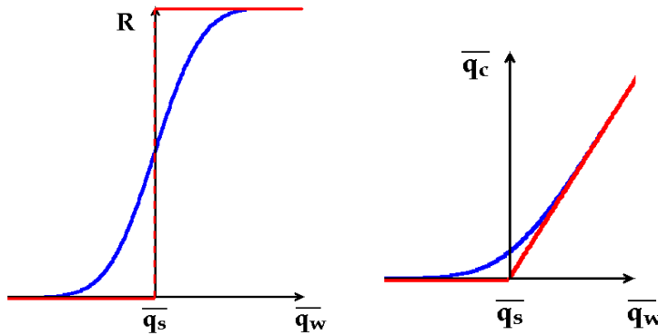
FIG. 4.3 – Effet du type du schéma sous-maille gaussien par rapport au schéma "tout ou rien" pour le calcul de la nébulosité R et du contenu spécifique en eau liquide nuageuse moyenne \bar{q}_c . On représente ici, la variation de R (à gauche) et de \bar{q}_c (à droite) en fonction de \bar{q}_w et de \bar{q}_s(T) pour le schéma "tout ou rien" (en rouge) et pour le schéma sous-maille gaussien (en bleu).
