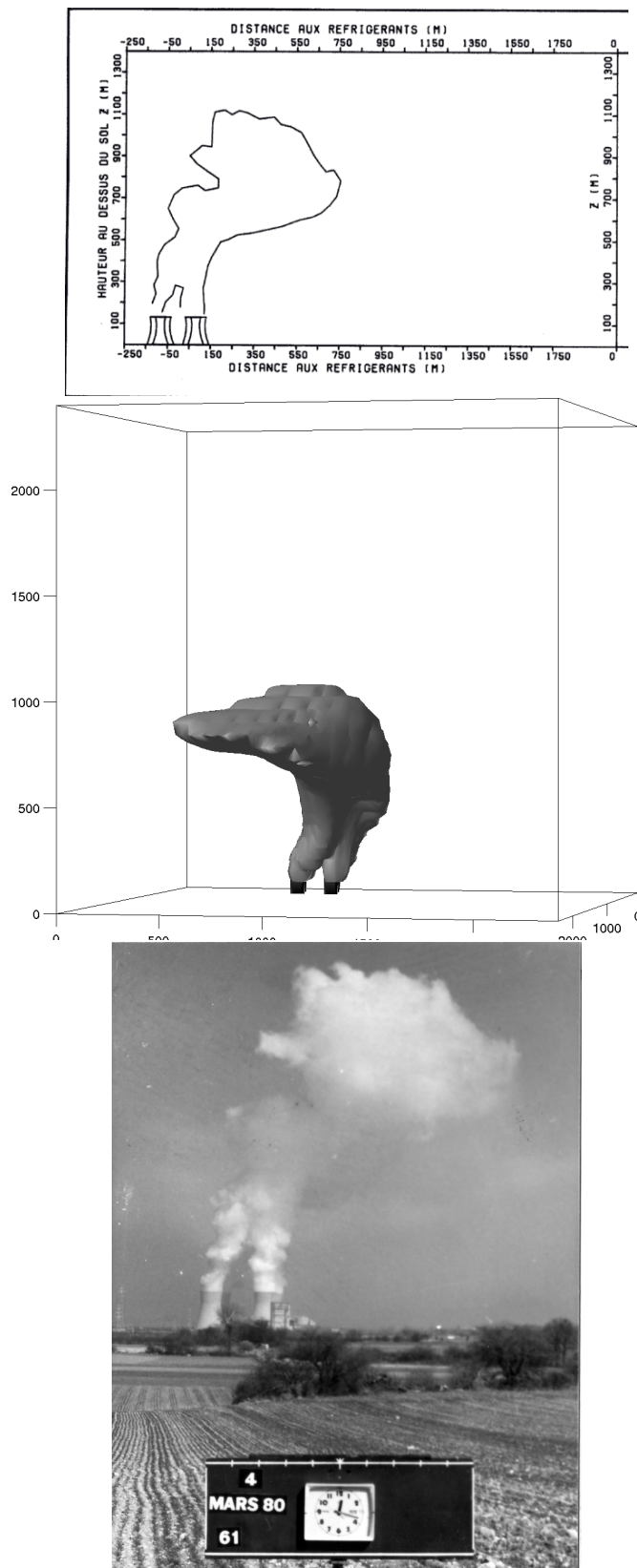
FIG. 7.12 – Le 4 mars 1980, photo et croquis à 12h15, simulation réalisé à 11h00.
