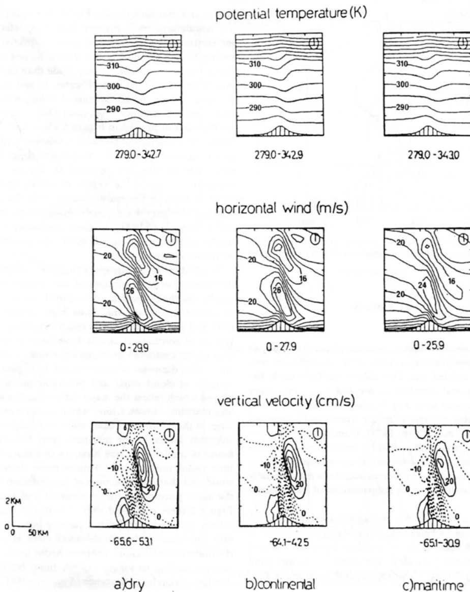
FIG. 12.1 – Température potentielle, composante horizontale et verticale de la vitesse du vent (de haut en bas). Les cas traités sont le cas sec, le cas de continental et le cas maritime (de gauche à droite). Les valeurs des principaux iso-contours sont annotées. (Tiré de la Fig. 3. de l'article de CRPN).
