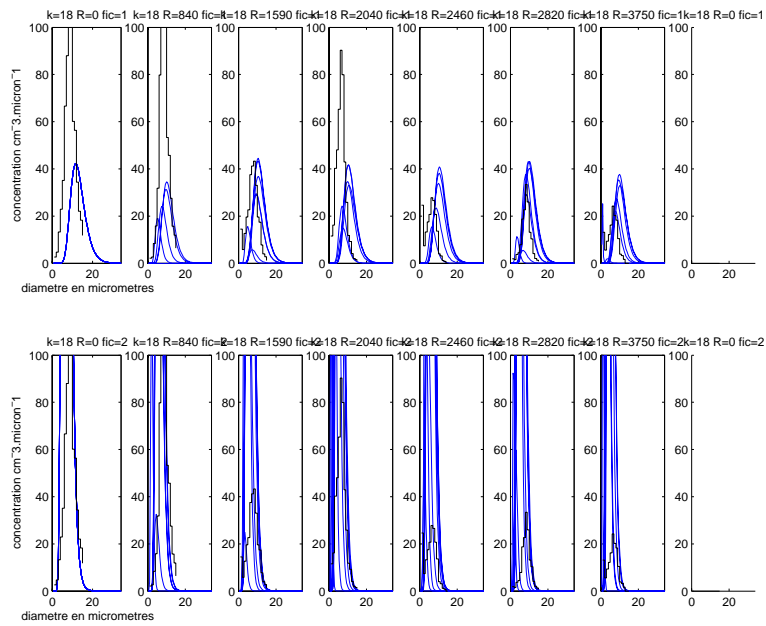
FIG. B.75 – Idem figure B.70. Palier n°9.
