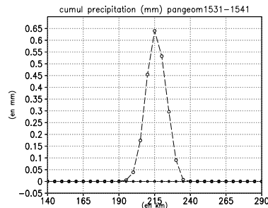
FIG. 12.9 – Idem Fig 12.7 pour les sorties MERCURE avec le maillage raffiné (50 niveaux sur la verticale au lieu de 15 et \Delta X = 5km ).
