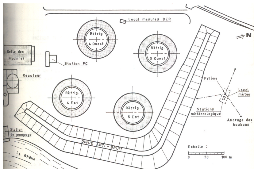
FIG. 6.2 – Plan des tours aéroréfrigérantes de la centrale du Bugey
