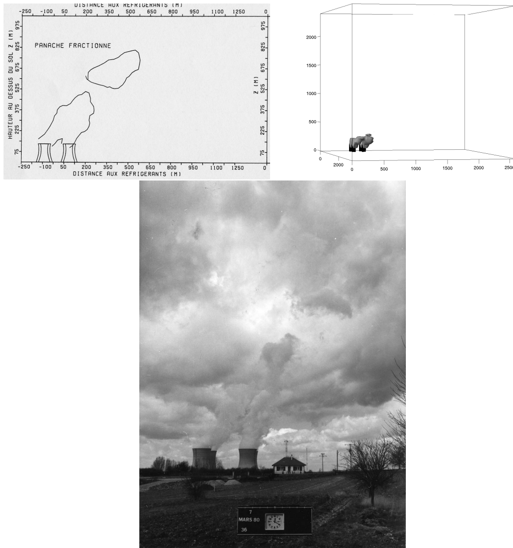
FIG. B.12 – Le 7 mars 1980, photo à 12h22, croquis à 12h20 et simulation réalisé à 10h52.
