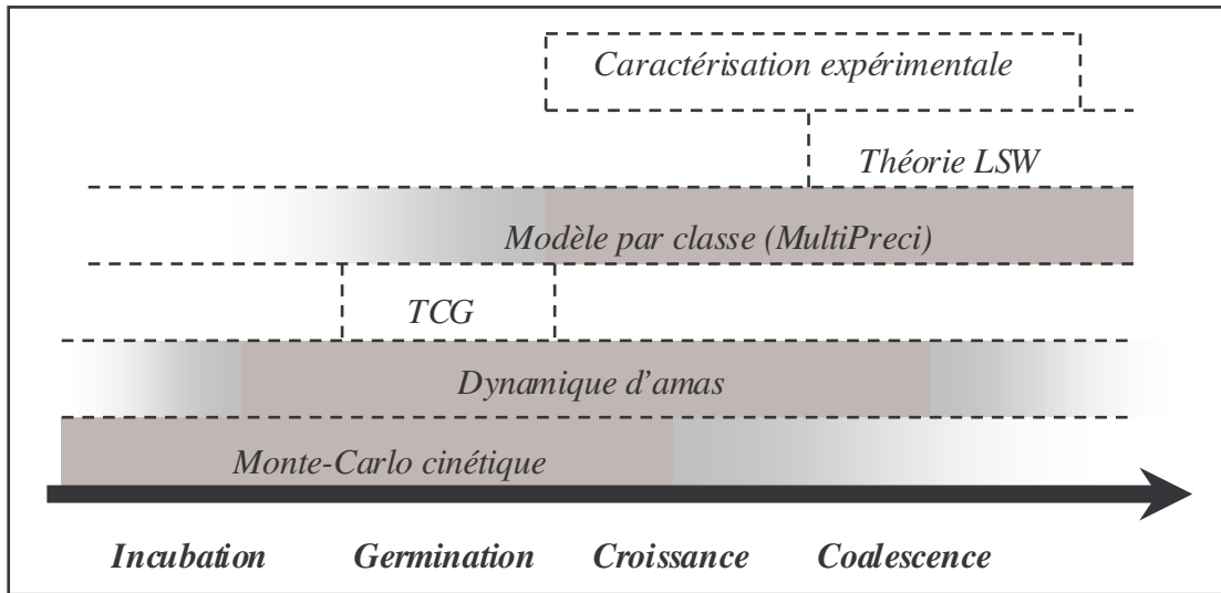
Fig. III.12 : positionnement de quelques modèles et outils de simulation sur l'échelle des phénomènes de précipitation.
