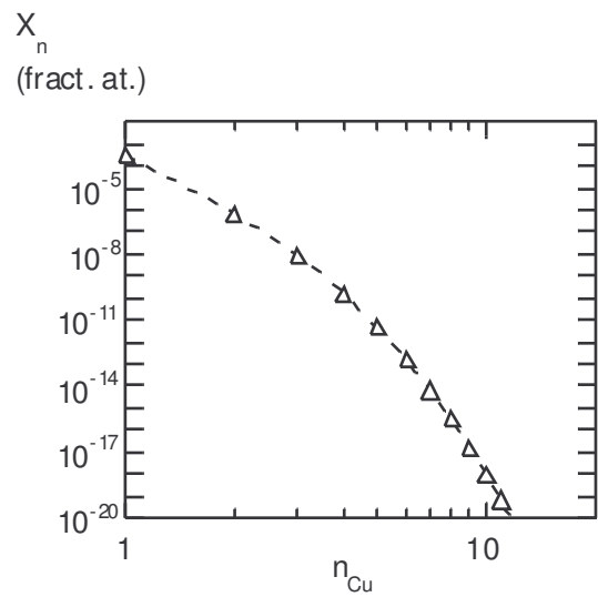
Fig. IV.2 : distribution de Boltzmann des amas à l'équilibre thermique à 500 °C.
