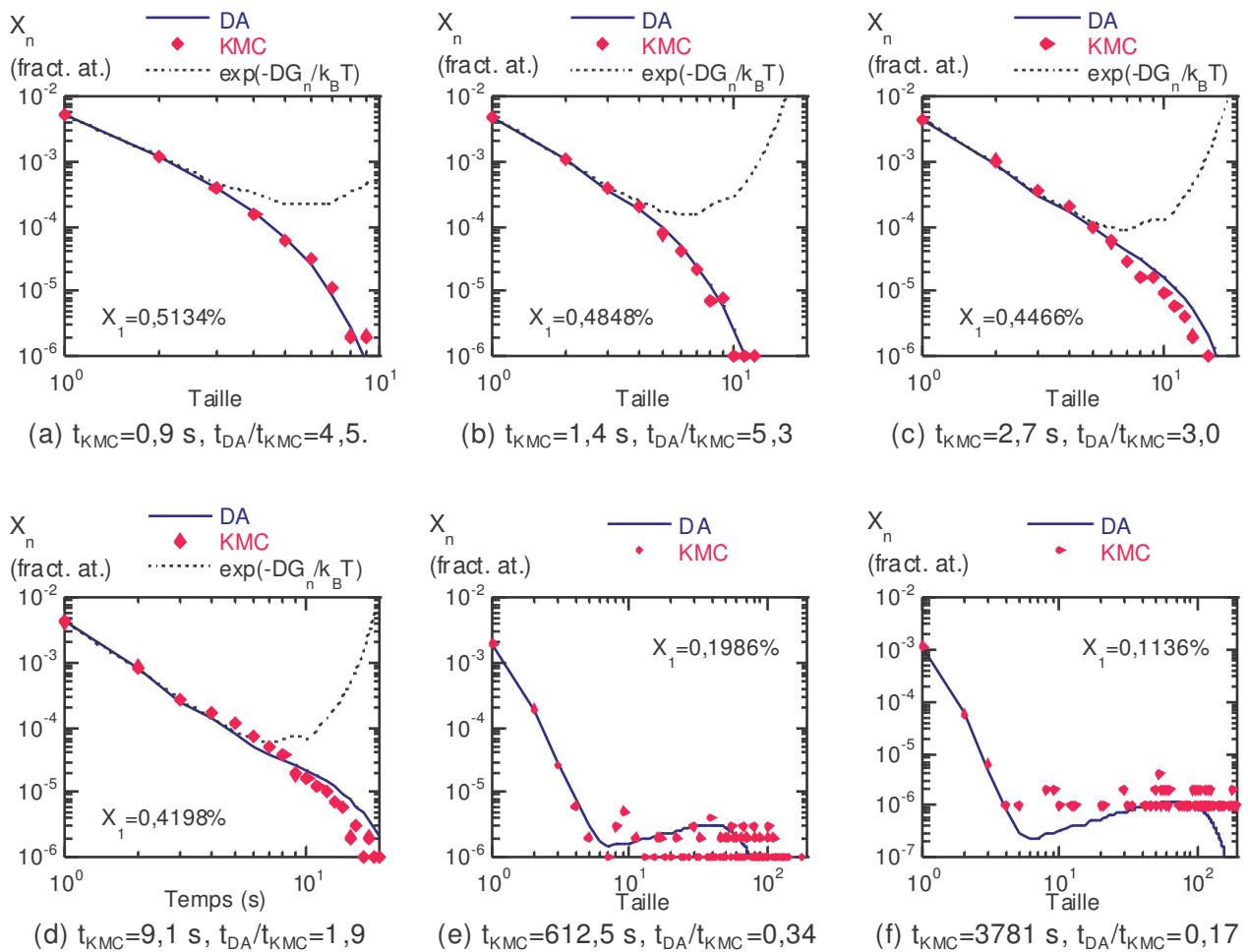
Fig. V.5 : comparaison des distributions d'amas en dynamique d'amas et en Monte Carlo Cinétique pour le système \underline{AlZr}(1\%) , à 450°C.
