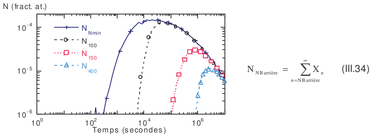
Fig. III.10 : évolution de la densité de précipités définie à l'aide de la formule III.34 lors d'une simulation sur le système fer -cuivre (méthode n^2 , X_{Cu}^0=1\% , 773K , \sigma=0,38 J.m^{-2} ) et diverses tailles barrière.
