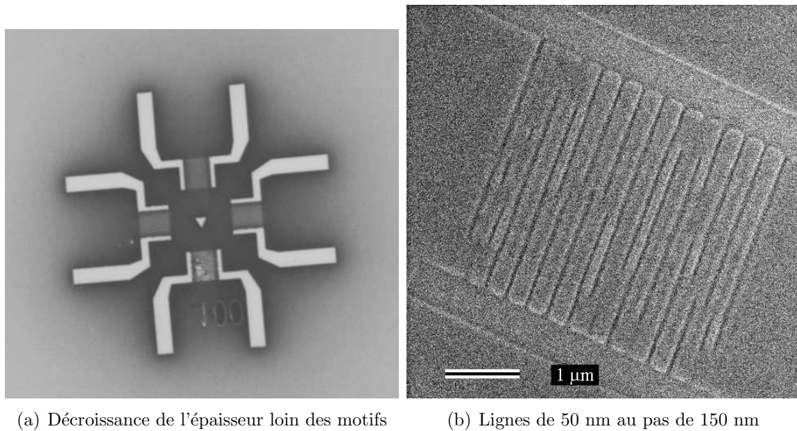
Figure 3.17 Limitations de la résine époxy-siloxane en terme de profil et de résolution
