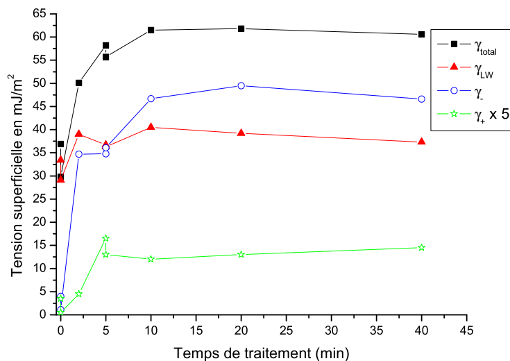
Figure 3.25 Variation des différentes composantes l'énergie de surface du LaF_3 en fonction du temps d'exposition au traitement UV/ozone.
