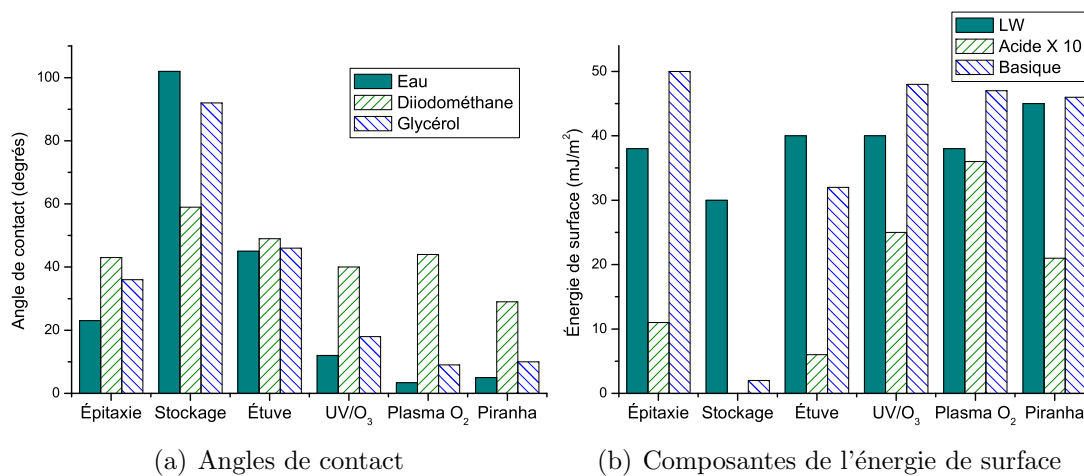
Figure 3.24 Effet de différentes méthodes de nettoyage sur l'énergie de surface du LaF 3 .
