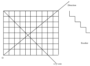
FIG. 1.2 – Suites sturmiennes.
