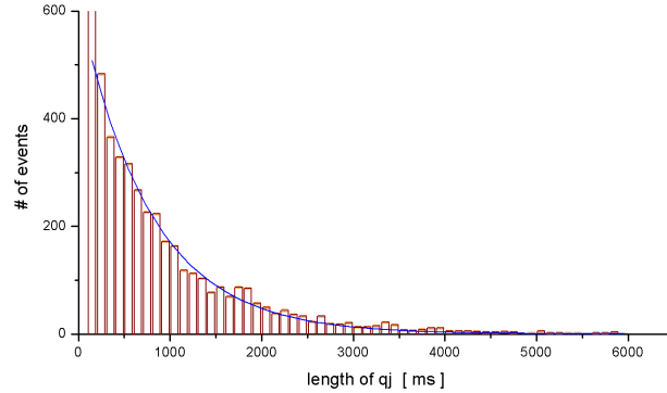
Fig. 4.3: Histogramme des sauts quantiques, représentant la décroissance exponentielle du niveau 3D_{5/2} .
