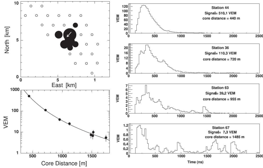
FIG. 2.18 – Événement 255146 : Un événement typique au dessus de 5 \cdot 10^{18} eV En haut à gauche : Réseau prototype avec les 8 stations touchées par l'événement. En bas à gauche : Ajustement de la LDF. A droite : Les traces ADC de 4 stations pour des distances comprises entre 439 m et 1480 m de l'axe de la gerbe. Le signal est en unité de VEM
