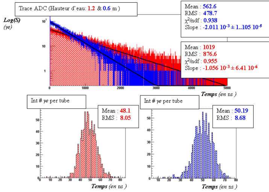
FIG. 3.3 – 1000 électrons de 10 MeV
