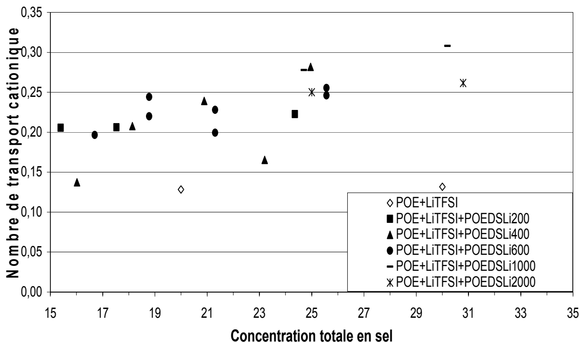
Figure 69 : Nombre de transport cationique des électrolytes polymères POE+LiTFSI+POEDSLi
