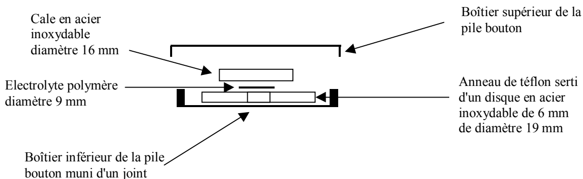
Schéma 7 : Schéma d'une cellule électrochimique de type pile bouton pour les mesures de conductivité
