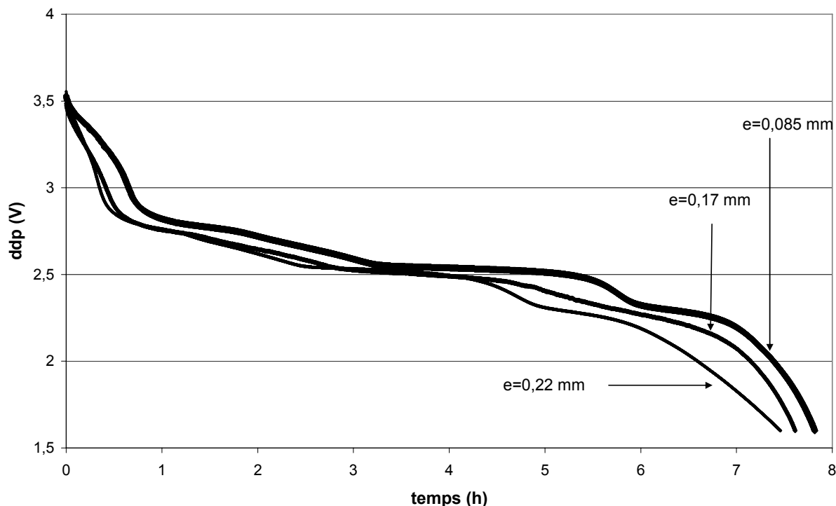
Figure 13 : Décharge d'accumulateurs lithium polymère
