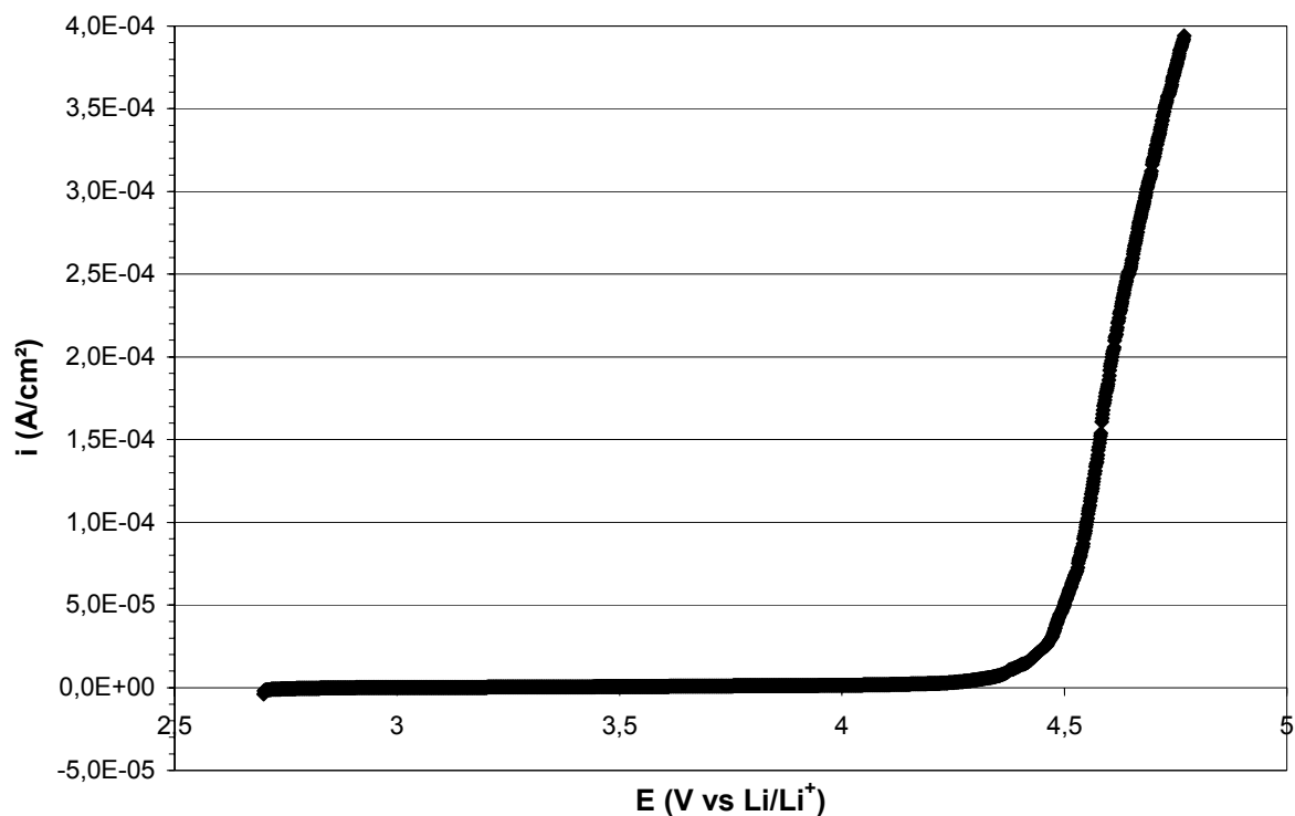
Figure 104 : Oxydation du polyélectrolyte P(OE/SLi) (10) en milieu liquide
