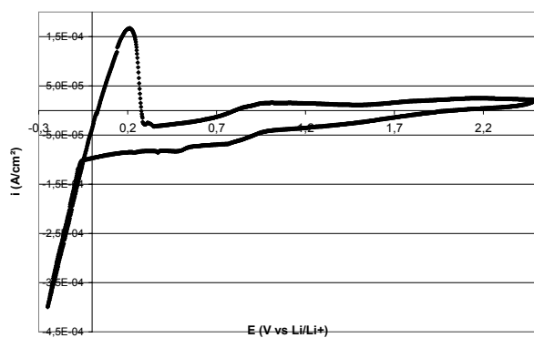
Figure 59 : Etude voltampérométrique d'électrolytes polymères POE
