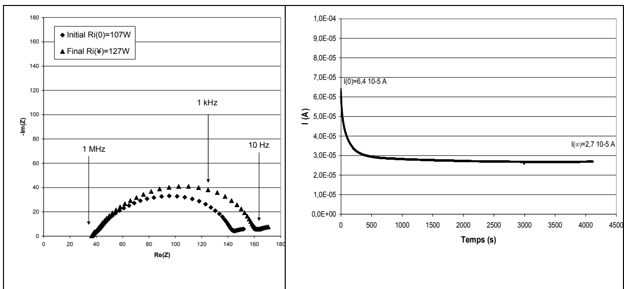
Figure 123 : Résultats d'une expérience sur l'électrolyte POE POEMSLi164 O/Li=30 LiTFSI O/Li=30 pour la méthode 1. Le paramétrage en fréquence est donné sur le graphe
