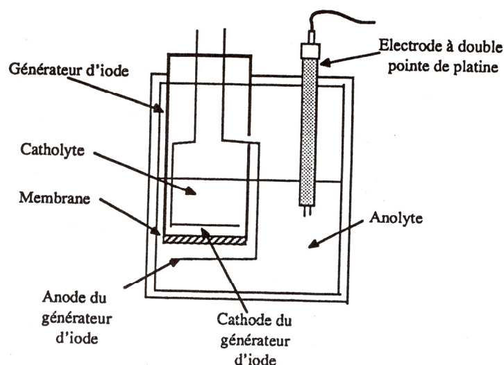
Schéma 6 : Schéma de la cellule de dosage coulométrique de type Karl Fisher
