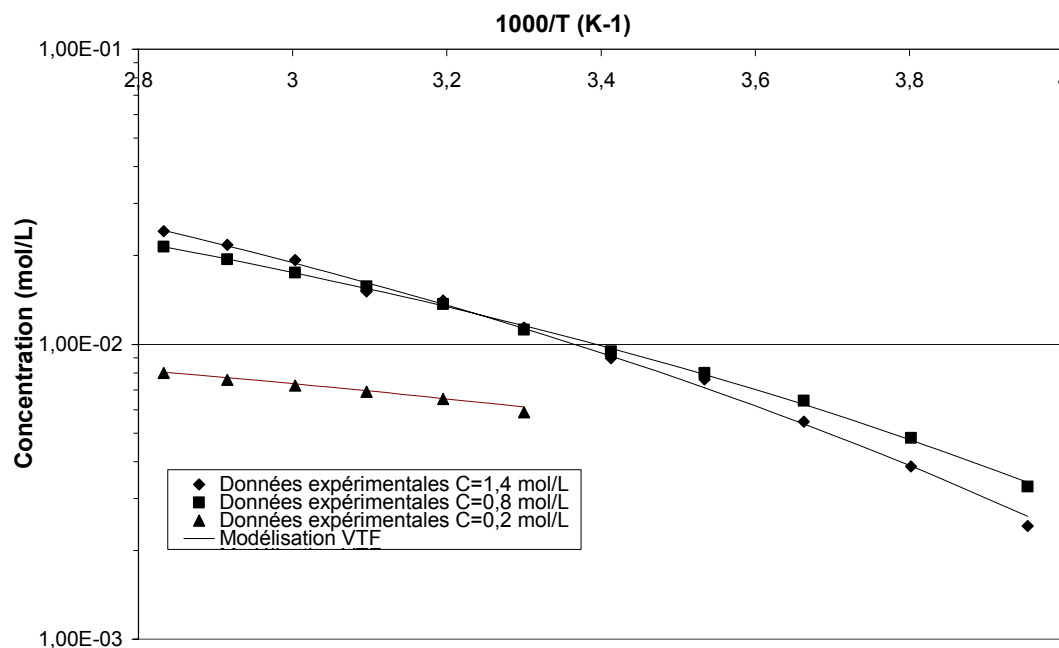
Figure 6 : Mesure de conductivité en fonction de la température pour différentes concentrations en LiPF 6 dans EC/DMC (1/1) et modélisation VTF
