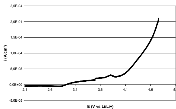
Figure 59 : Etude voltampérométrique d'électrolytes polymères POE
