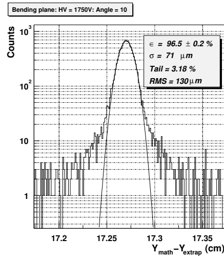
FIG. 3.44 – Résidu typique à 1750 V pour une rotation de 10° autour de l’axe défini par les fils d’anode, pour le plan de courbure.
