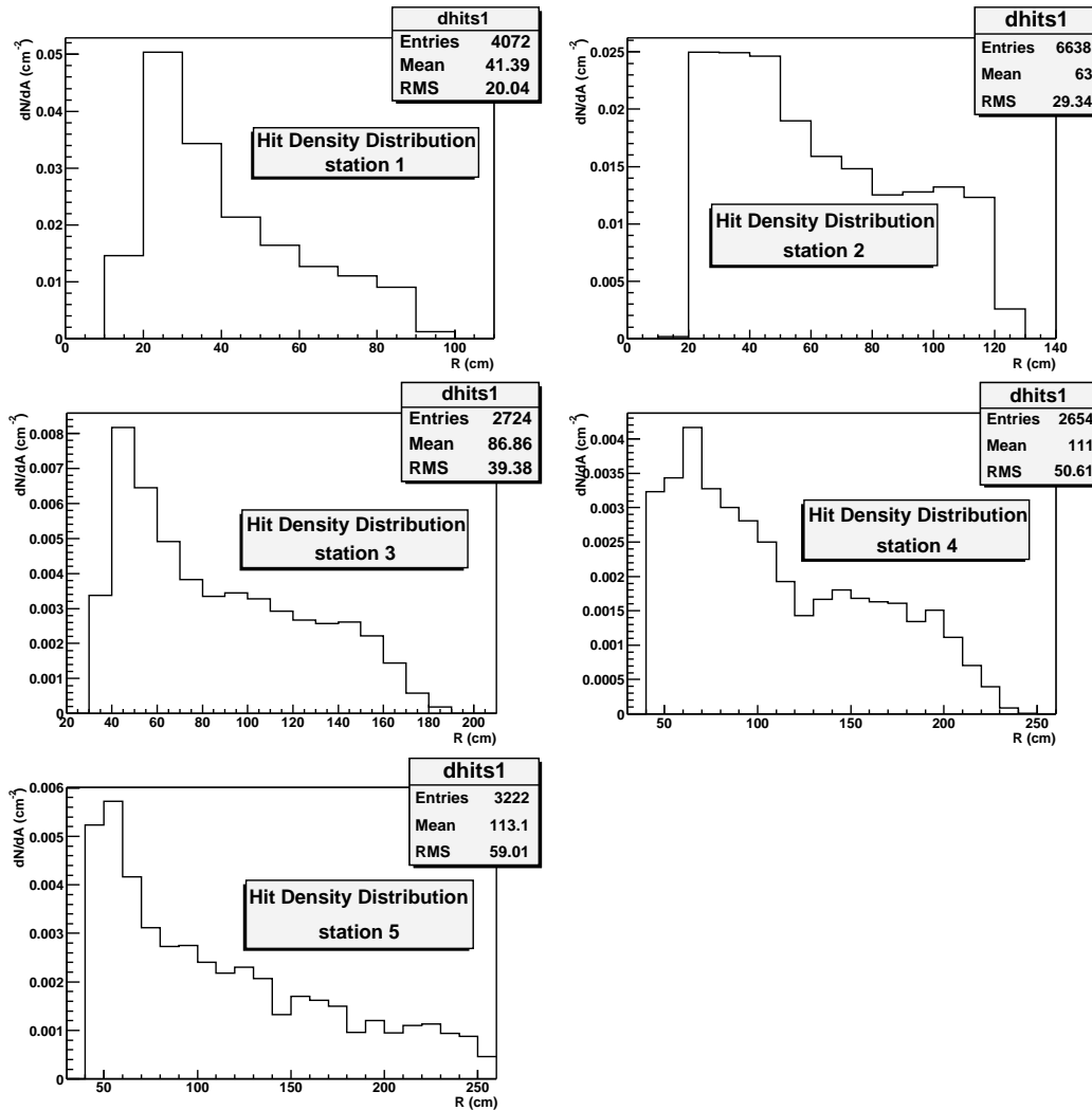
FIG. 3.5 – Densité d'impacts (particules/cm 2 /évènements) dans les chambres en fonction du rayon, pour les 5 stations.
