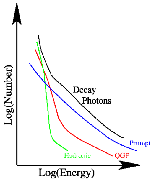
FIG. 1.9 – Modélisation des distributions en énergie des photons directs (“prompt”, “QGP”, “hadrons”) et issus des décroissances (“decay” des \pi^0 ou des \eta ) [35].
