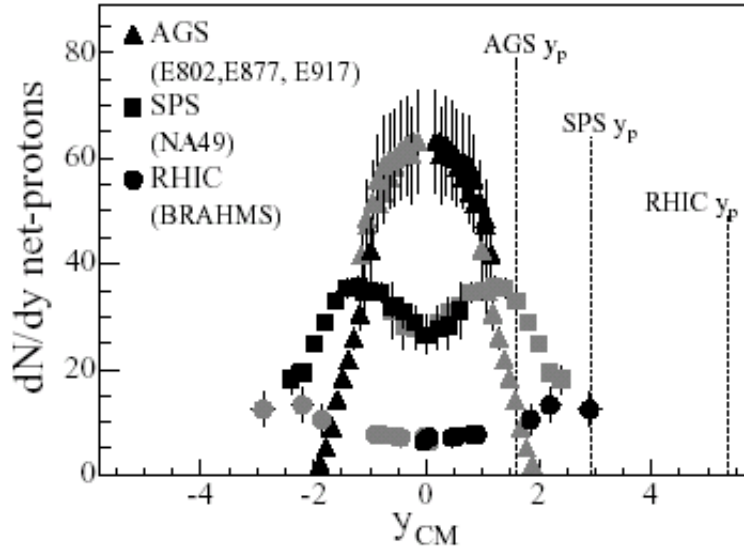
FIG. 1.8 – Etude de la transparence pour des collisions de différentes énergies : les données des collisions Au-Au de \sqrt{s} = 5 GeV à l’AGS sont indiquées par les triangles, celles des collisions Pb-Pb de \sqrt{s} = 17 GeV au SPS sont indiquées par les carrés, et celles des collisions Au-Au de \sqrt{s} = 200 GeV au RHIC sont indiquées par les cercles [34].
