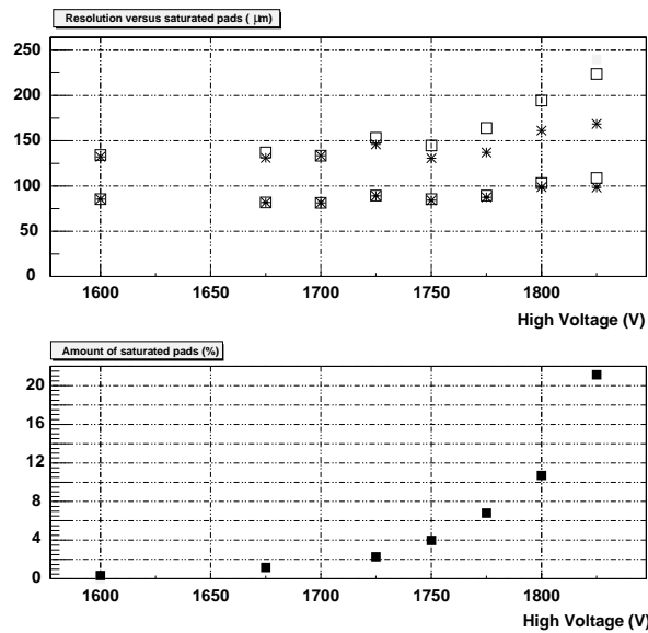
FIG. 3.36 – Etude des effets de saturations en fonction de la haute-tension. Le graphe du haut présente la résolution avec (carrés blancs) ou sans (étoiles noires) saturations pour deux méthodes différentes (RMS : 2 courbes supérieures et ajustement Gaussien : 2 courbes inférieures). La figure du bas donne le pourcentage d’agrégats saturés en fonction de la haute-tension.
