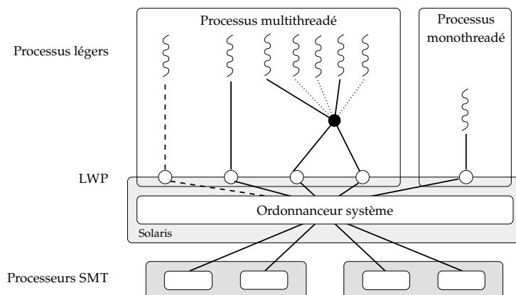
FIG. 3.5 – Le modèle de processus légers de SOLARIS
