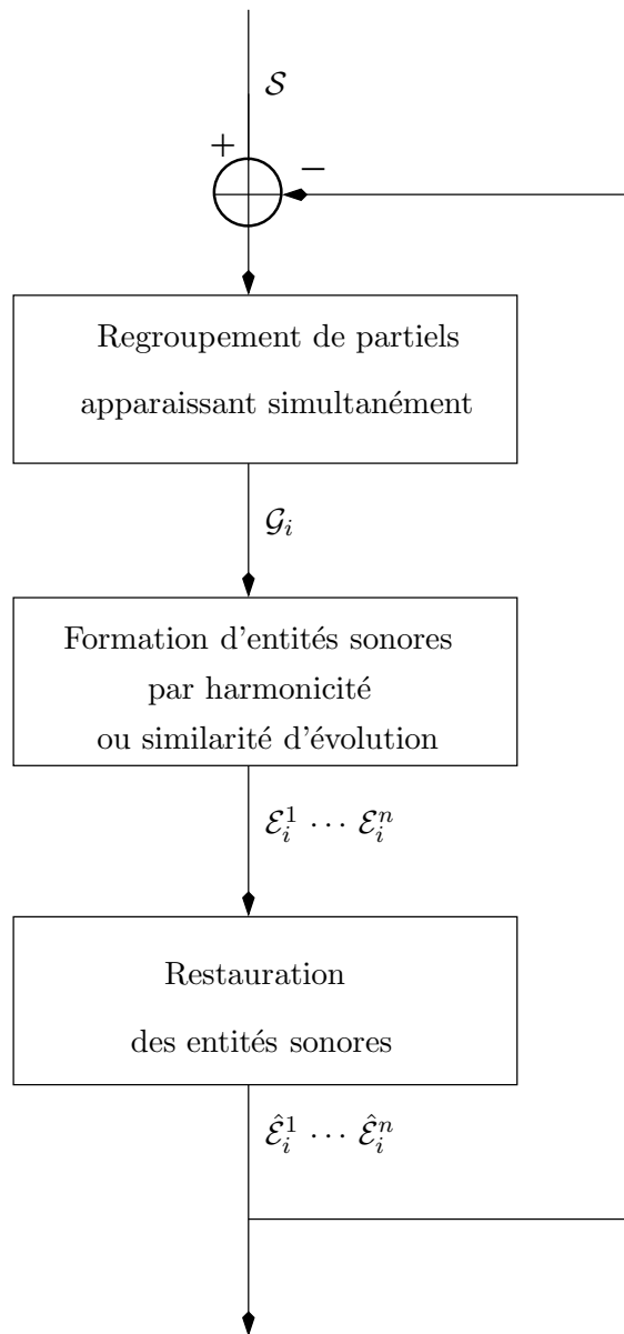
FIG. 5.2 – Sch ma de principe de l'algorithme d'extraction d'entit s sonores. On cherche dans l'ensemble des partiels \mathcal{S} une apparition simultan e de partiels   une trame donn e. On regroupe alors dans \mathcal{G}_1 les partiels qui sont apparus ensemble. De ce groupe sont extraites les entit s sonores \mathcal{E}_1^1 \dots \mathcal{E}_1^n , n  tant le nombre d'entit s trouv es dans le groupe \mathcal{G}_1 . Ces entit s sonores sont ensuite restaur es. Les partiels de \mathcal{S} appartenant   ces entit s restaur es sont ensuite enlev s et une nouvelle apparition simultan e est recherch e pour former \mathcal{G}_2 .
