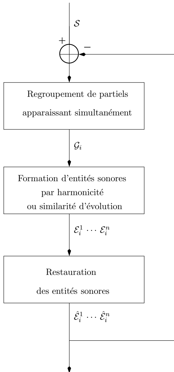
FIG. 5.2 – Sch ema de principe de l'algorithme d'extraction d'entit es sonores. On cherche dans l'ensemble des partiels \mathcal{S} une apparition simultan ee de partiels   une trame donn ee. On regroupe alors dans \mathcal{G}_1 les partiels qui sont apparus ensemble. De ce groupe sont extraites les entit es sonores \mathcal{E}_1^1 \dots \mathcal{E}_1^n , n  tant le nombre d'entit es trouv ees dans le groupe \mathcal{G}_1 . Ces entit es sonores sont ensuite restaur ees. Les partiels de \mathcal{S} appartenant   ces entit es restaur ees sont ensuite enlev es et une nouvelle apparition simultan ee est recherch ee pour former \mathcal{G}_2 .
