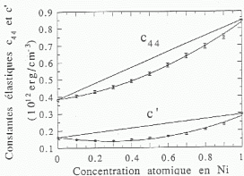
Figure III.10 : Constante élastique c_{44} et c' en 10^{12} \text{ erg cm}^{-3} calculées conformément à l'annexe 4.
