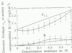
Figure III.11 : Constantes élastiques c_{11} et module de compressibilité B en 10^{12} \text{ erg cm}^{-3} . Voir le texte pour les barres d'erreurs et l'annexe 4 pour la méthode utilisée.
