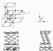
Figure I.17 : Représentations tridimensionnelle de l'épitaxie Fe(211) sur MgO(110) . En haut, construction du plan 2x + y + z = 1 et en bas, visualisation de l'épitaxie selon deux perspectives bien distinctes. La vue de gauche permet de distinguer un des deux domaines possibles.
