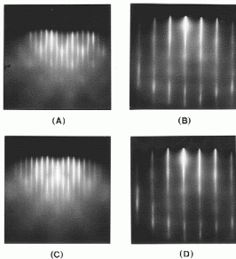
Figure I.21 : Diagramme de diffraction de la surface d'au reconstruite (1 \times 2) selon les azimuts [1\bar{1}0] à gauche et [001] à droite pour un dépôt de 2000 Å d'au, avant recuit (en haut) et après un recuit de 420 K pendant 10 minutes (en bas).
