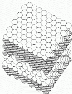
Une multicouche Au(111)/Ni(111) avec une désorientation de 30 degrés.
