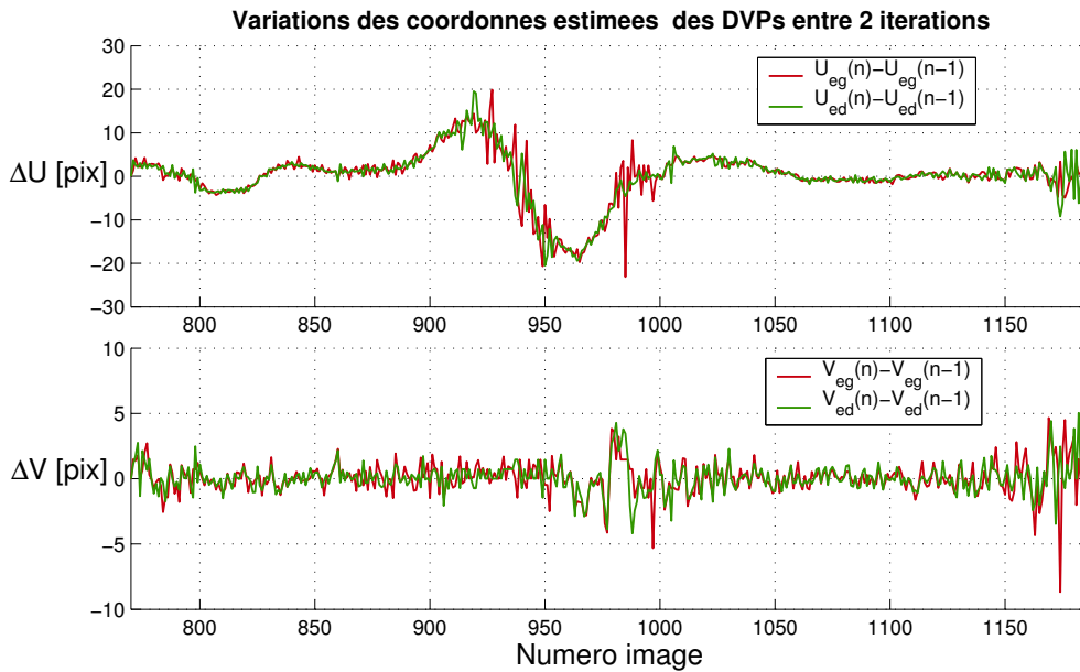
FIG. 5.3 – Ecart s entre les coordonnées mesurées et prédites des DVPs, fournies par le filtre de Kalman. Le comportement du filtre prédictif est conforme à nos attentes : la prédiction fournie est proche de la mesure précédente. Les variations observées sont donc proches du mouvement apparent du DVP entre deux images et peuvent atteindre quelques dizaines de pixels en abscisse et moins de 5 pixels en ordonnée, en faisant exception des erreurs de mesures.
