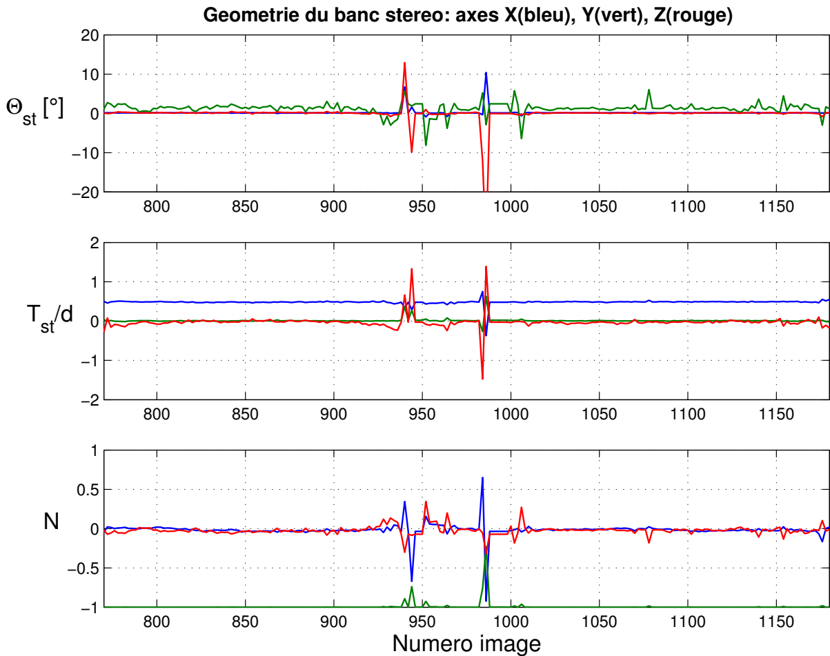
FIG. 4.25 – Décomposition des mouvements de rotation \theta_{st} et translation normalisée \mathbf{T}_{st}/d entre les repères \mathbf{C}_g et \mathbf{C}_d et évolution de la normale au plan de la route \mathbf{N} . Les paramètres intrinsèques des caméras étant inconnus, les valeurs numériques, obtenues à partir d'une matrice générique, sont données à titre indicatif. L'hypothèse de rigidité de la paire stéréo est vérifiée sur la majeure partie de la séquence. Les écarts observés entre les images [936,948] et [986,998] sont dues à une mauvaise répartition des primitives coplanaires détectées sur le plan de la route.
