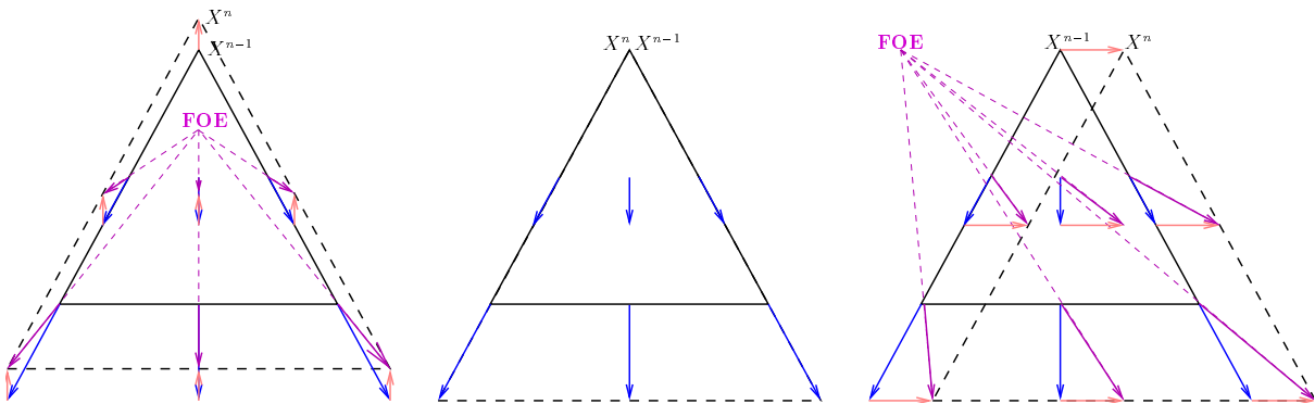
FIG. 5.14 – Champ de composition des vitesses de FPs coplanaires entre deux poses de la caméra. Les vecteurs bleus représentent le mouvement apparent des FPs dû au mouvement de translation selon l'axe optique de la caméra. Leur amplitude augmente linéairement en fonction de leur ordonnée. Les vecteurs roses correspondent, eux, au mouvement de rotation selon l'angle de lacet. L'introduction du mouvement de rotation a écarté le FOE de sa position initiale, localisée en X^{n-1} .
