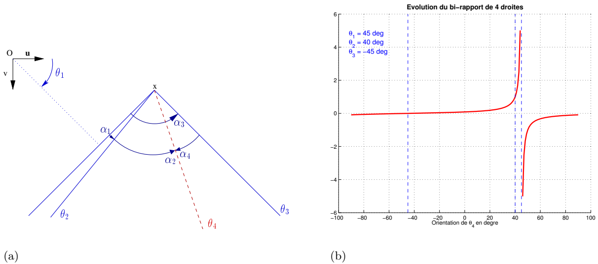
FIG. 3.3 – Le bi-rapport étant invariant par homographie, nous calculons le bi-rapport d'un faisceau de quatre droites dont l'orientation de trois d'entre elles sont fixées à -45^\circ , -40^\circ et 45^\circ . La pente du bi-rapport évolue grandement en fonction de la position relative de la 4 ème droite en fonction des trois autres, ce qui justifie qu'un critère d'invariance fixe ne permettra pas forcément d'identifier deux représentations différentes d'un même faisceau de quatre droites.
