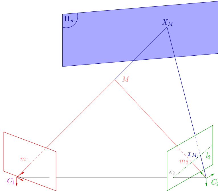
FIG. 3.7 – Projection d'un point dans deux images. La projection x_{M_2} du point m_1 par H_\infty permet d'obtenir l'extrémité de la projection dans l'image \mathcal{I}_2 du rayon passant par le point M . Le correspondant m_2 du point m_1 se trouve donc entre l'épipôle e_2 et H_\infty \cdot m_1 .
