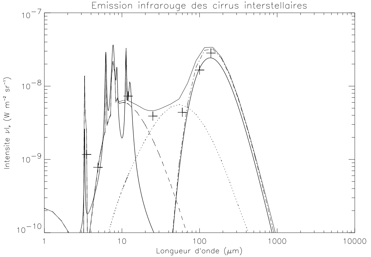
FIG. 1.1 – Spectre infrarouge des poussières interstellaires. Les observations, croix et lignes en gras, sont normalisées à une densité de colonne de 10^{20} \text{ H cm}^{-2} d'hydrogène. La raie à 3.3 \mu\text{m} provient de Giard et al. (1994) [117], les autres bandes sont des profils lorentziens calées sur les observations ISOCAM de \rho \text{ Oph} par Boulanger et al. (1998) [88], les croix sont les mesures DIRBE du plan galactique par Bernard et al. [18] et enfin le spectre submillimétrique, résumé par l'équation 1.1, provient de FIRAS (Lagache et al. 1999 [45]). Le modèle en trait fin est exactement celui publié en 1990 [12]. Il se décompose de gauche à droite en l'émission des PAHs, des petits grains VSGs et des gros grains.
