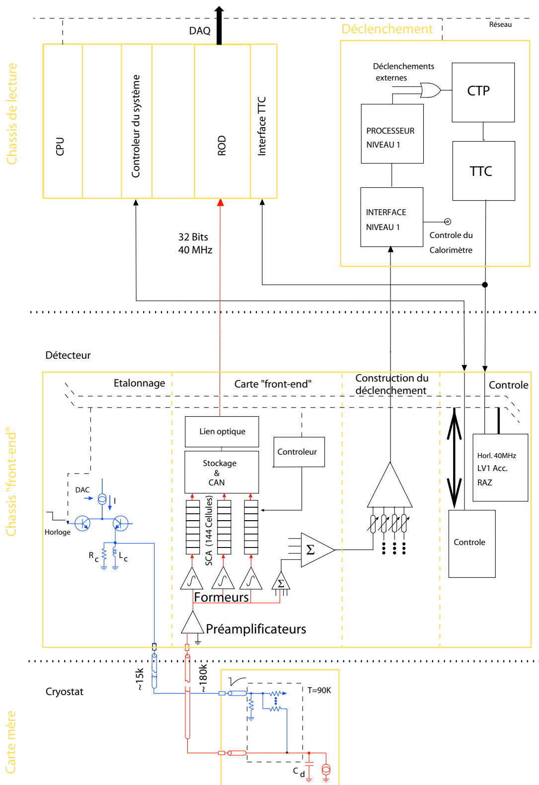
FIG. 3.1 – Schéma électrique de la chaîne de lecture et d'étalonnage du calorimètre EM d'ATLAS. On peut distinguer la partie acquisition (en rouge) et le système d'étalonnage (en bleu).
