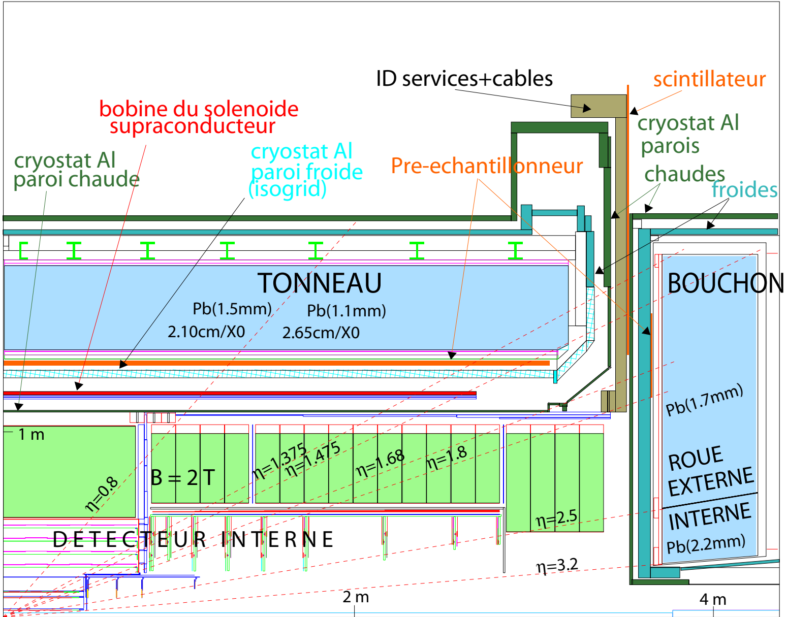
FIG. 2.18 – Coupe longitudinale d'un quart du détecteur ATLAS mettant en évidence les parties tonneau et bouchon du calorimètre électromagnétique.
