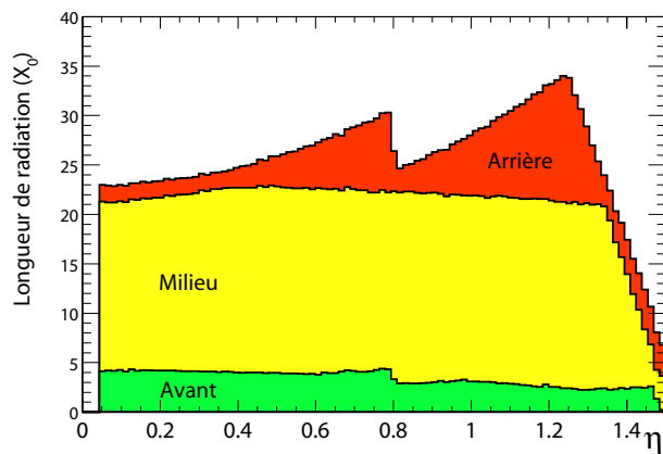
FIG. 2.22 – Variation de la longueur de radiation avec \eta pour les différents compartiments du calorimètre électromagnétique tonneau [36].
