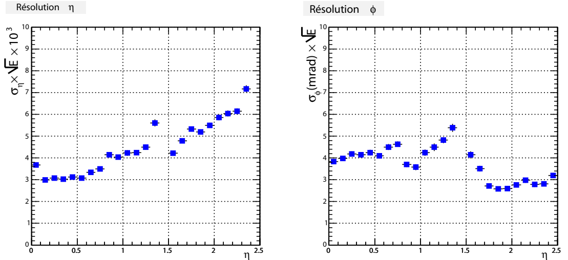
FIG. 5.13 – Résolution globale sur la mesure de la position moyenne selon \eta et \phi en fonction de la position \eta de la gerbe électromagnétique dans le calorimètre pour des photons non convertis avec p_T = 60 \text{ GeV} .
