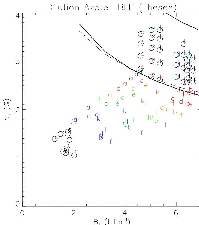
Figure IV-11 : Sensibilité des résultats de simulation à la variable N_T de dilution de l'azote dans la biomasse aérienne ( B_T ). Chaque année (1986 à 1994) est représentée par une lettre de l'alphabet et chaque niveau d'enrichissement en azote (0 à 250 kg ha -1 ) par une couleur. Les lettres entourées sont exclues de l'étude. Les courbes de dilutions optimales et maximales définies par STICS sont représentées en trait plein.
