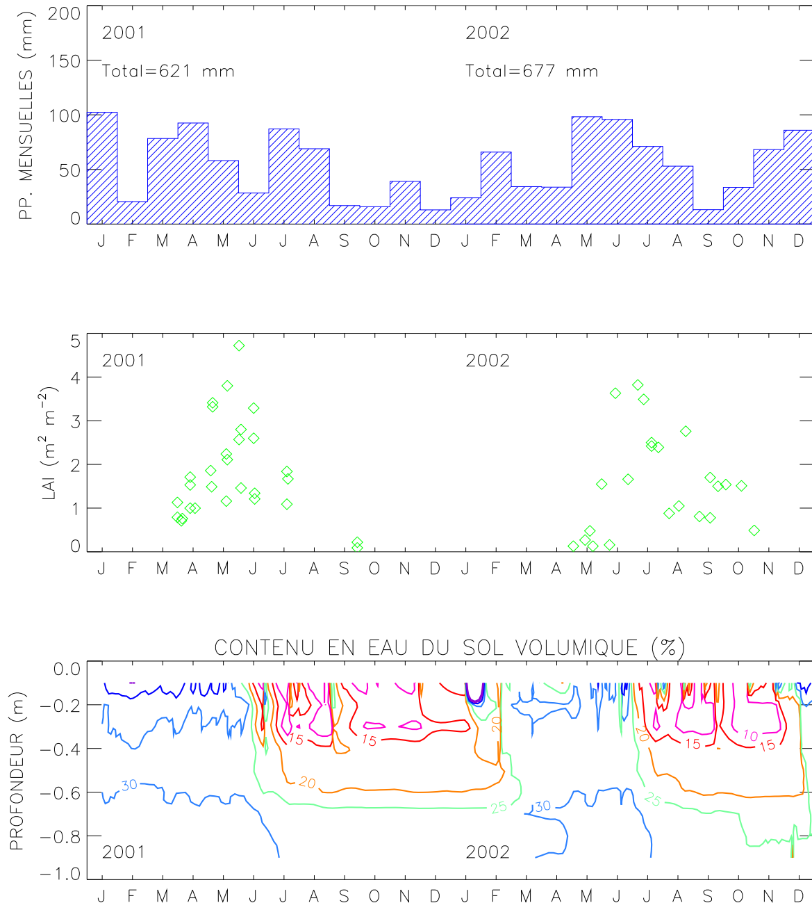
Figure IV-14 : Mesures de précipitations mensuelles, indice foliaire (LAI) et contenu en eau volumique sur le site de SMOSREX pour les années 2001 et 2002.
