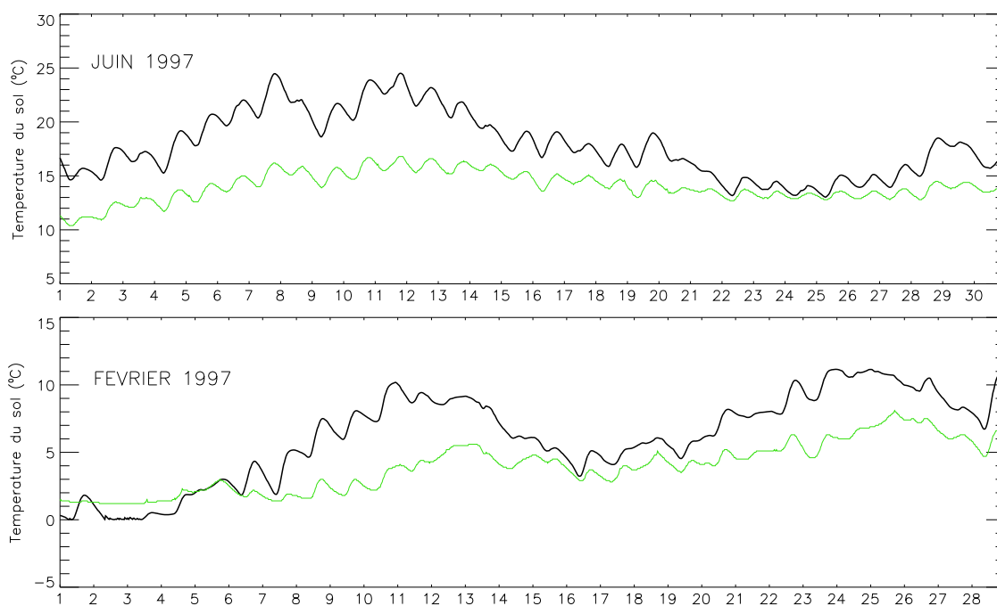
Figure III-26 : Evolution de la température du sol à 10 cm mesurée sur le site pour les périodes de juin 1997 et février 1997 (trait clair) et la simulation de température profonde T_2 du modèle (trait foncé).
