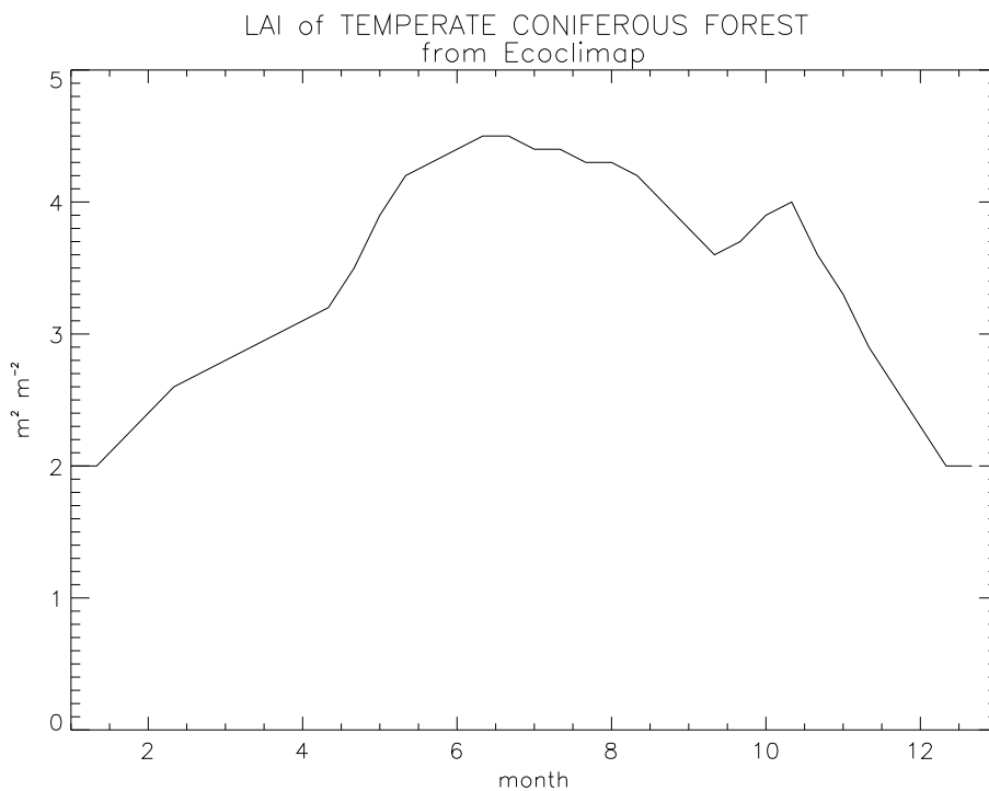
Figure III-17 : évolution annuelle du LAI de la classe "forêt de conifère tempérée" extraite de la base ECOCLIMAP (Masson et al. , 2002).
