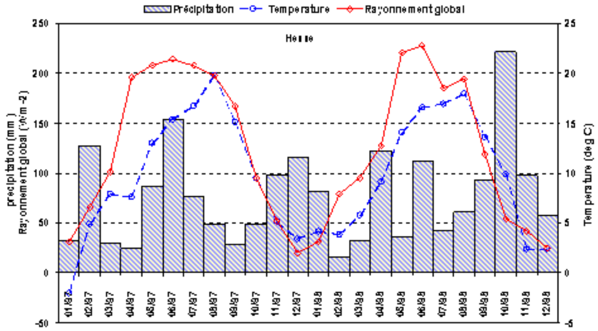
Figure III-3 : Évolution des variables climatiques moyennées du site de "Hesse" sur la période d'étude ; précipitations (mm), température ( ^{\circ}C ) et rayonnement global ( W m^{-2} ).
