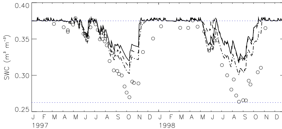
Figure III-29 : Simulations du contenu volumique en eau dans la colonne de sol ( d_2=1.6 m) avec la version ISBA-Standard (traits alternés), la version ISBA-A-g s , végétation imposée (AST, trait plein) et végétation dynamique (LST, trait tiretés). Les observations sont présentées (ronds) ainsi que la capacité au champ ( w_{fc} ) et le point de flétrissement ( w_{wilt} ) en pointillés.
