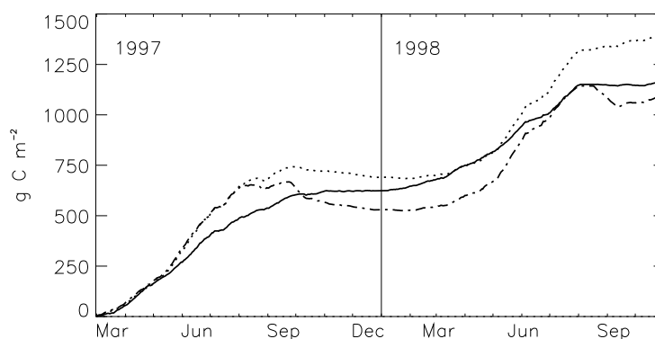
Figure III-46: 2 ans d'évolution du cumul journalier net de carbone (NEE). Sont présentés avec le cumul observé (trait plein), la simulation ISBA-A-g s incluant le sous-bois de molinie en mode végétation forcée (trait alternés), et la simulation avec la seule paramétrisation du pin (trait tireté).
