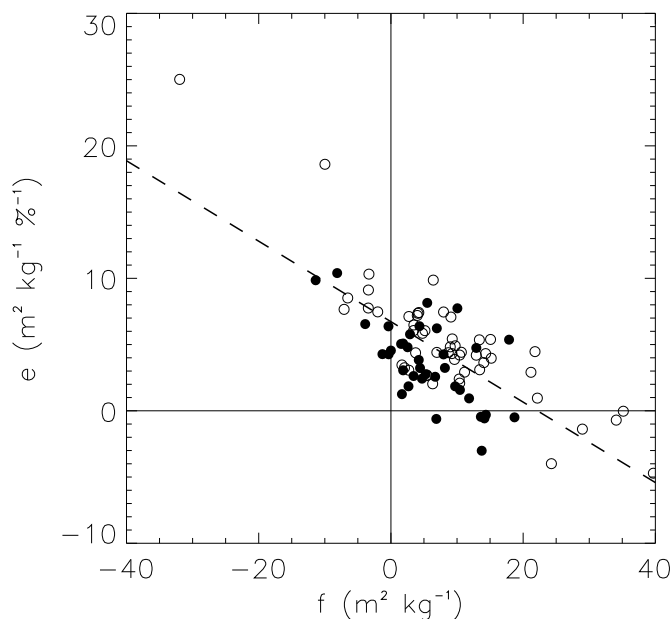
Figure IV-4 : Relation entre les paramètres e et f , herbacées (cercles) et ligneux (points) confondus et la régression associée (IV-22) (traits tirés). Données des Tableau IV-2 et Tableau IV-3.
