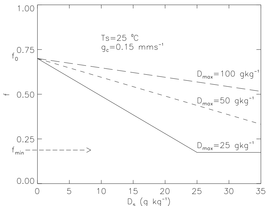
Figure I-4 : évolution du paramètre f en fonction du déficit de vapeur d'eau de l'air pour différentes valeurs de D_{max} , g_m(25^\circ C) = 1 \text{ mm s}^{-1}
