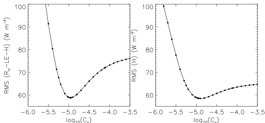
Figure III-21 : Résultats de l'optimisation du paramètre de capacité thermique de la végétation. Les résultats présentent les valeurs de \epsilon_{RMS}(R_n-LE-H) et \epsilon_{RMS}(H) en fonction du logarithme décimal de C_v .
