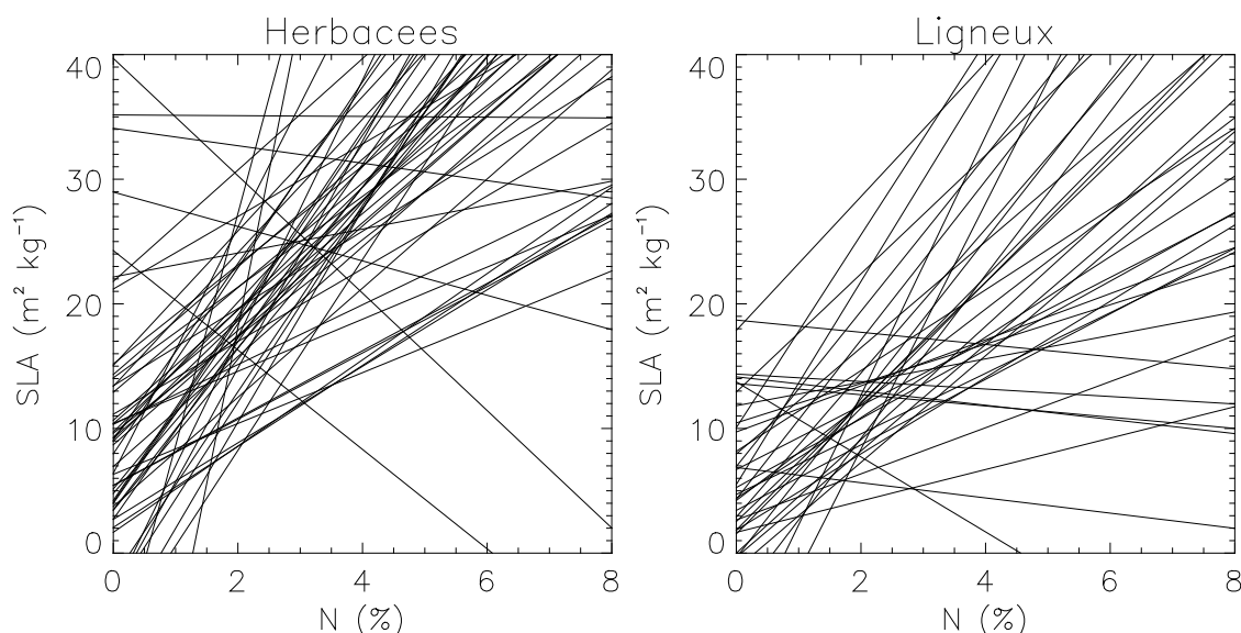
Figure IV-6 : Faisceau de droites reliant la surface spécifique foliaire (SLA) à la teneur en pourcentage d'azote dans la biomasse aérienne (N). Les pentes et ordonnées à l'origine des droites sont respectivement les paramètres e et f des tableaux Tableau IV-2 et Tableau IV-3.
