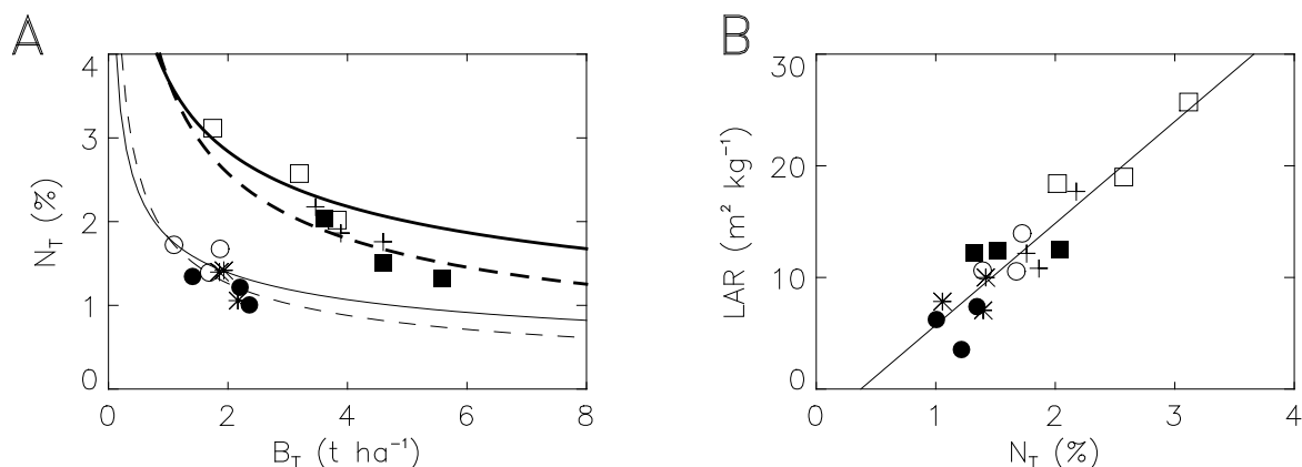
Figure IV-2 : Relations allométriques observées et simulées reliant la concentration en azote, la biomasse et le LAI pour un ray-grass pérenne. Extrait de Calvet et Soussana (2001). (A) Concentration en azote des parties aériennes en fonction de la biomasse totale aérienne. (B) Rapport LAI/B_T en fonction de la concentration aérienne en azote. Les mesures sont extraites des travaux de Casella et al. (1996) et Soussana et al. (1996) et sont représentés par des astérisques et des ronds pour un faible traitement azoté, des croix et des carrés pour un fort traitement azoté, des symboles vides pour une concentration en carbone atmosphérique actuelle et pleins pour une concentration doublée, et les croix et astérisques pour une concentration doublée et une augmentation de la température de l'air de 3^\circ C .
