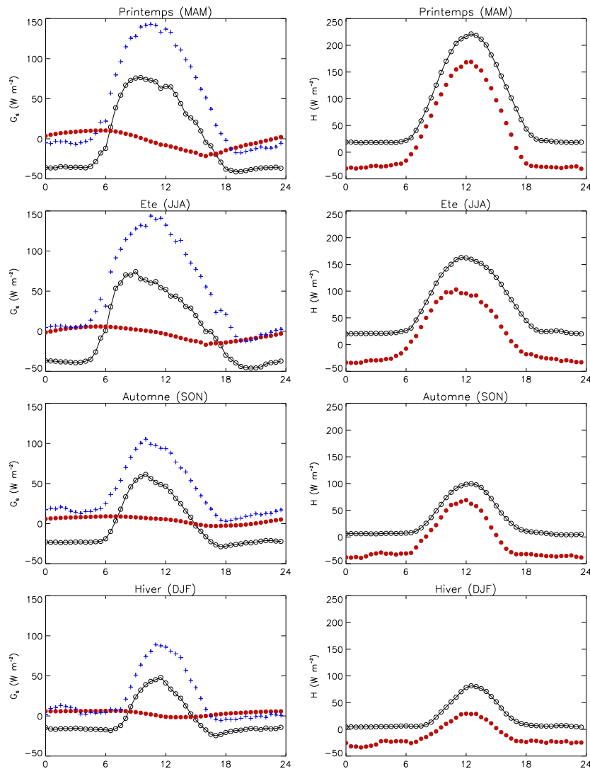
Figure III-28 : A gauche , cycle diurne du flux de conduction observé dans le sol (cercles pleins), résultant du défaut de bilan R_n-LE-H (croix) et simulé par le modèle dans sa version AST (cercles liés). A droite cycle diurne du flux de chaleur sensible observé (cercles pleins) et simulé (cercles liés).
