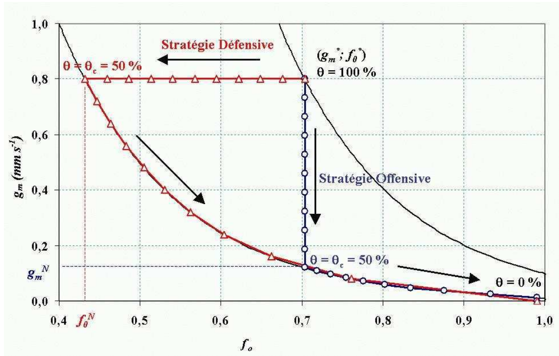
Figure II-14 : Schéma simplifié présentant l'évolution pour les plantes ligneuses des paramètres A-g_s g_m et f_0 , relatifs à une augmentation du stress hydrique. Les deux stratégies, défensive (triangles rouges) et offensive (rond bleu), sont présentées. \theta correspond la réserve utile normalisée. Les flèches présentent le sens d'évolution des paramètres lors d'une diminution de \theta . Le schéma présente des valeurs de g_m^* , f_0^* et \theta_c respectivement de 0.8 \text{ mm s}^{-1} , 0.7 et 50 \% .
