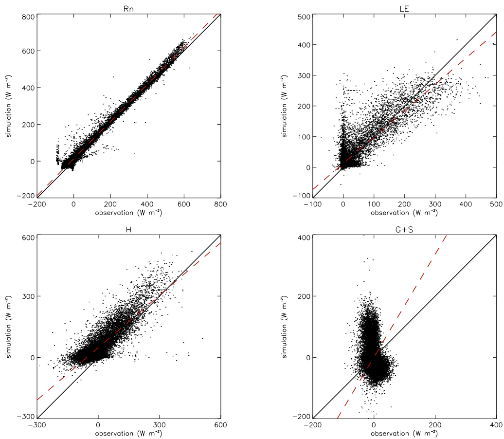
Figure III-27 : Comparaison entre les flux simulés par le modèle (version AST) et mesurés sur le site pour le rayonnement net (Rn), le flux de chaleur latente (LE), le flux de chaleur sensible (H) et le flux de conduction dans le sol + Stockage dans l'air (G+S).
