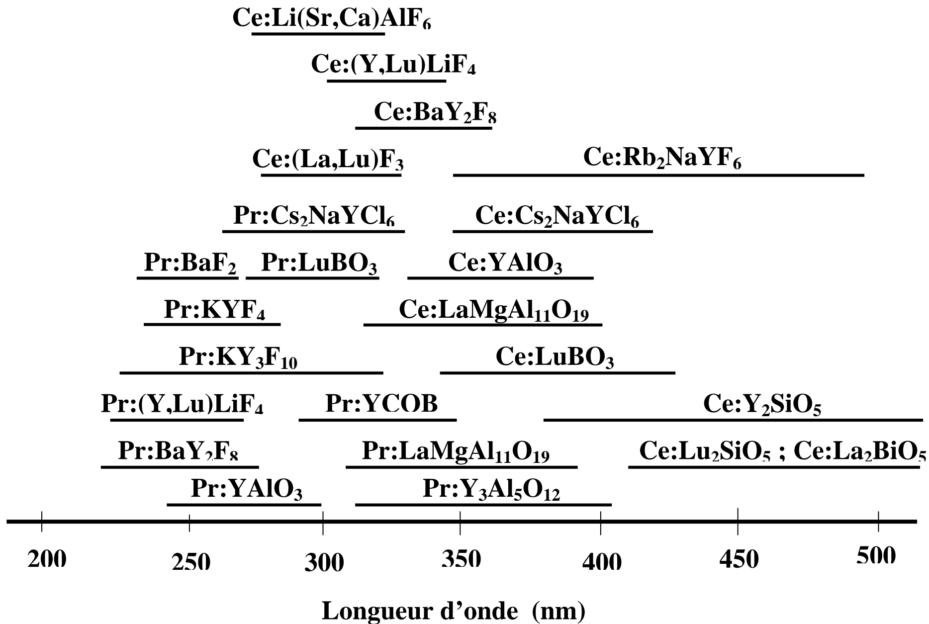
Domaines d'émission UV-VISIBLE de quelques matériaux dopés Ce 3+ ou Pr 3+
